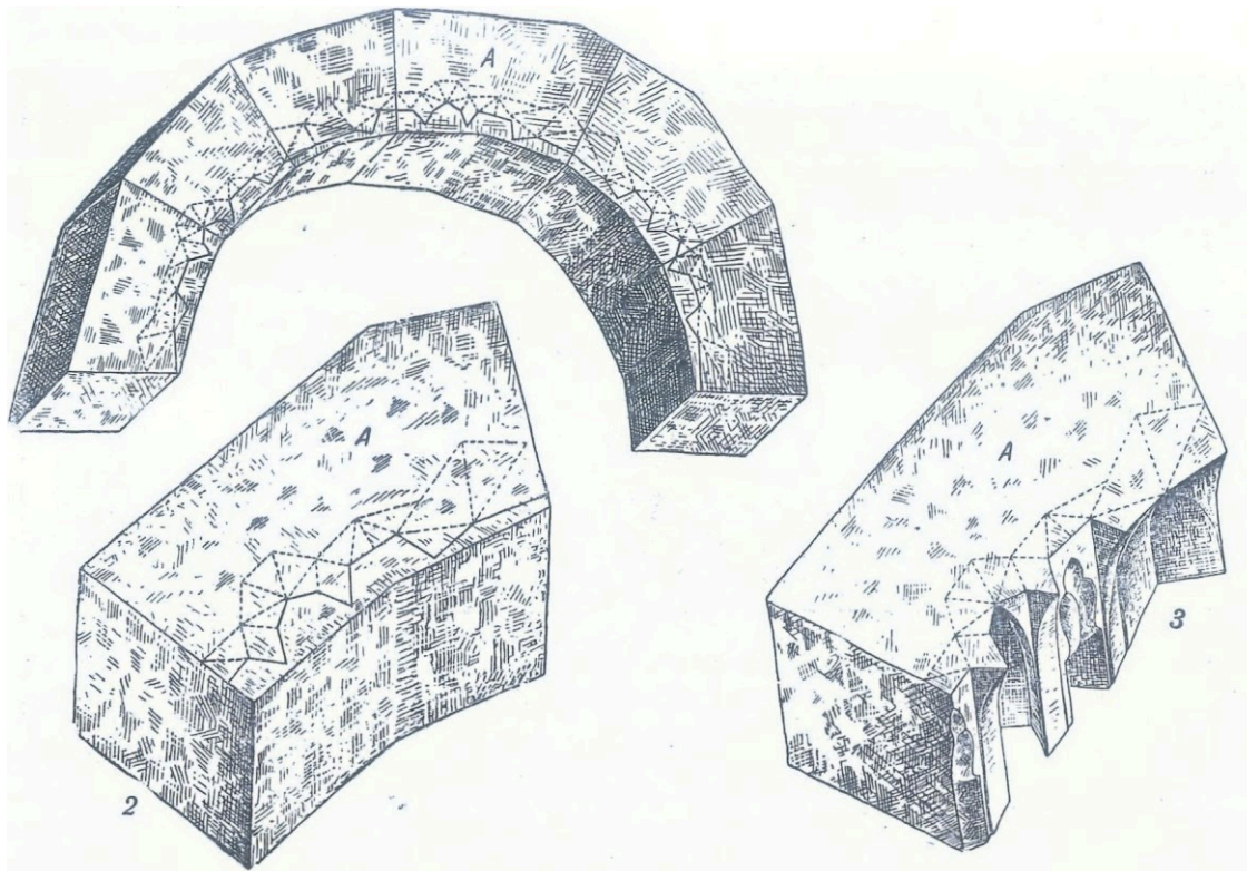
Рис. 64. Схема построения и изготовления сталактитов в камне.
