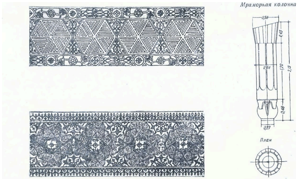
Рис. 75. Проект реконструкции колонной галереи мечети и развертка декораций колонны.
