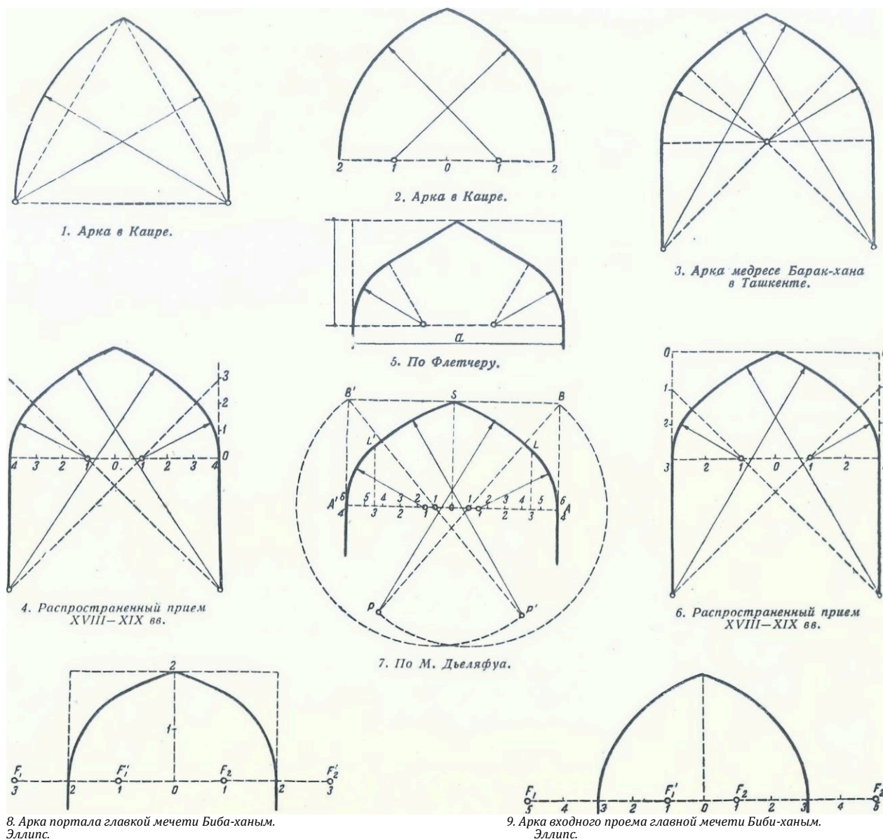
Рис. 50. Способы построения стрельчатых арок.
