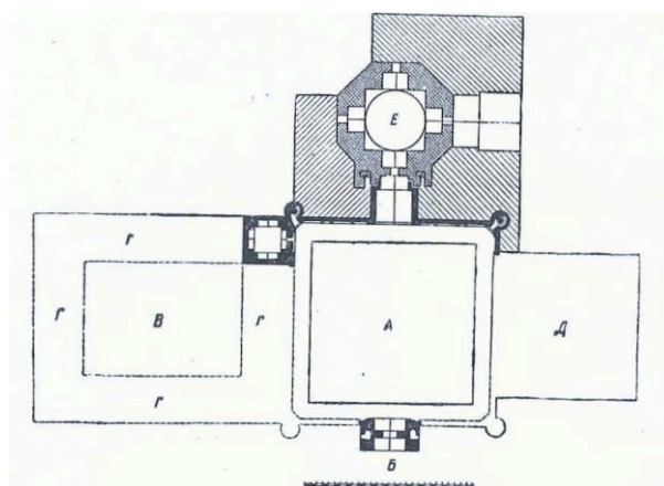
Рис. 14. Самарканд. План архитектурного комплекса Гур-Эмир Л—двор; Б—входной портал; В—двор медресе; Г—медресе; Д—хонака; Е— мавзолей Гур-Эмир
