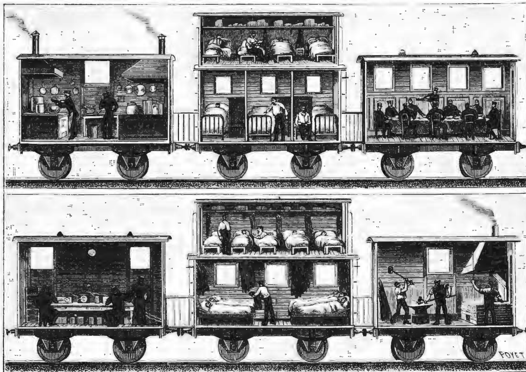
Занаспійская желѣзная дорога. Разрѣзъ важнѣйшихъ вагоновъ.
