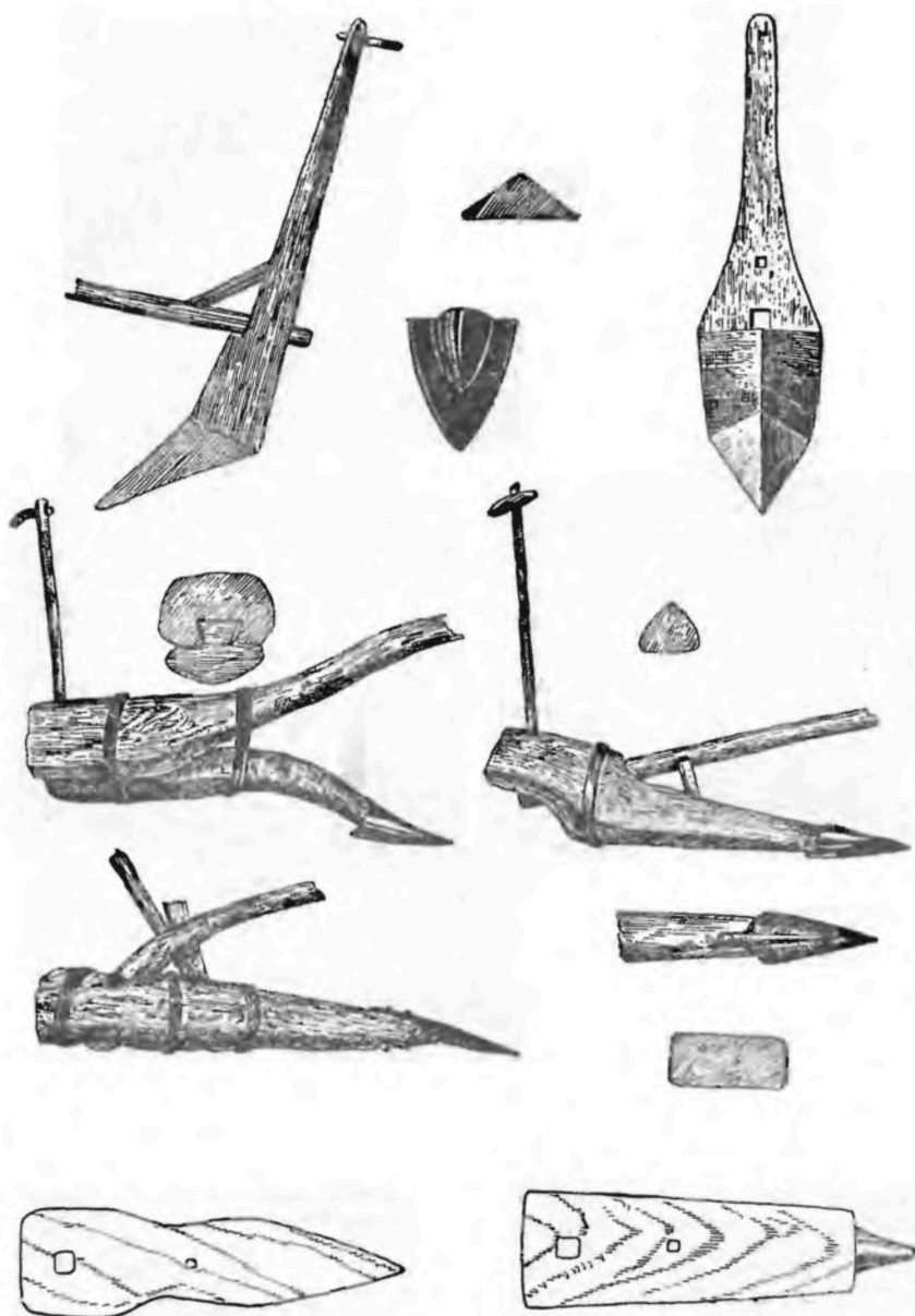
Рис. 3. Деревянные плуги из Афганистана начала XX в.
