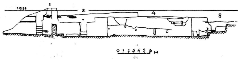
Рис. 23. Дворец. Разрез 3—В через помещения 8, 4, 2 и 3
