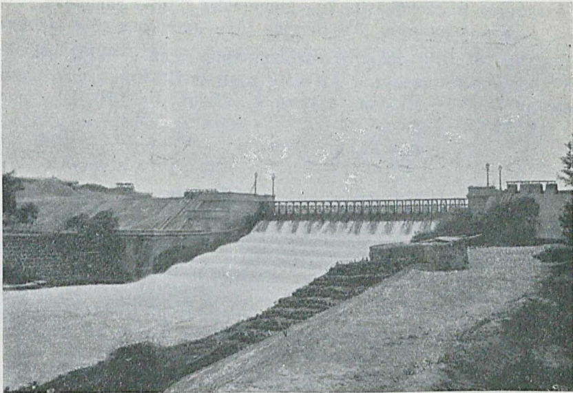
Мургабъ. Гиндукушская плотина.
