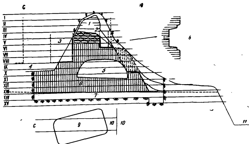
Рис. 3. Разрез крепостной стены древнего Кеша. I—XV—стратиграфические ярусы. 1—пахса XVIII в., 2—натки, 3—внутристенный коридор, 4—современный уровень, 5—камера, 6—пахсовый цоколь, 7—материк, 8—оформленные наружного фаса стены, 9—камера в плане, 10—откос цоколя, 11—уровень воды.
