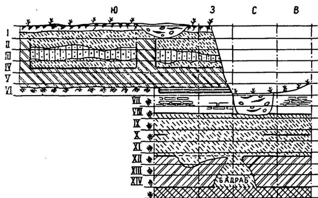
Рис. 1. Развертка стен шурфа № 4 в крепостной стене древнего Кеша. I—XIV — стратиграфические ярусы.
