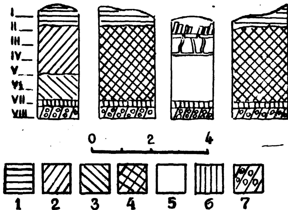
Рис. 14. Галатeпa. Шурф 2: 1—твёрдое заполнение; 2—кирпичная стена; 3—забутовка; 4—завал кирпича и пахсы; 5—пахсовая стена; 6—лёсс; 7—гравий
