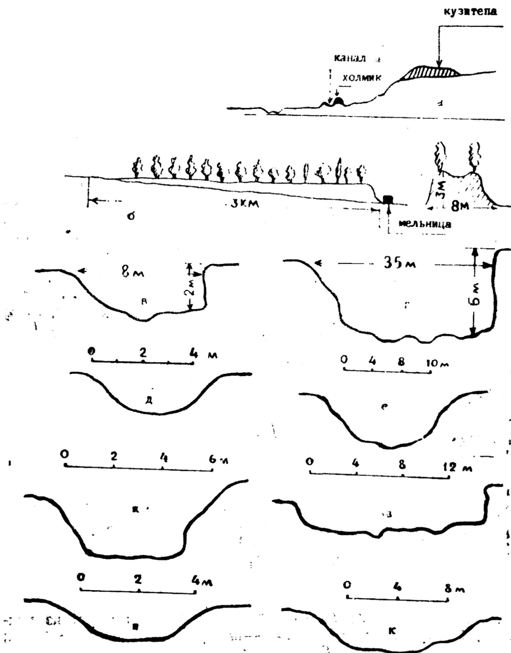
Рис. 5. Профили каналов: а—канал к западу от Кузитапа; б—продольный профиль Кипчакарыка; в—канал к северу от Кузитапа; г—канал к юго-западу от Кузитапа; д, е—каналы севернее селения Калининбад; ж—канал в районе Галатепе; з—канал у Кулудатепе; и—канал у тепа-1; к—канал в районе Галатепе
