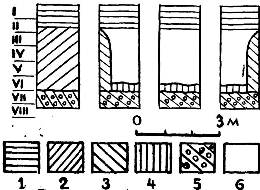
Рис. 13. Кулulatesа. Шурф 5: 1—рыхлый слой; 2—кирпичная стена; 3—приставная стена; 4—зольник; 5—гравий; 6—завал кирпича и пахсы
