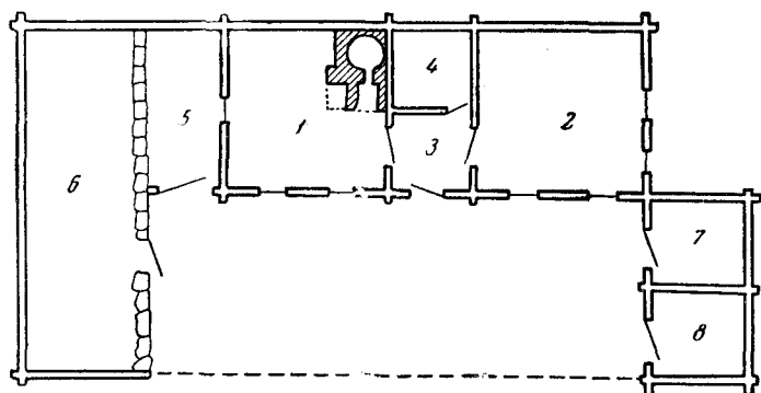
Рис. 1. Покособразная планировка шведской усадьбы: 1 — жилое помещение, 2 — чистое помещение, 3 — прихожая, 4 — каморка, кладовая, 5 — сарай, 6 — хлев, 7, 8 — амбары
