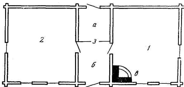
Рис. 5. План норвежского крестьянского дома: 1 — жилое помещение с отопительной системой (в), 2 — чистое помещение, 3 — прихожая (а), каморка (б)
