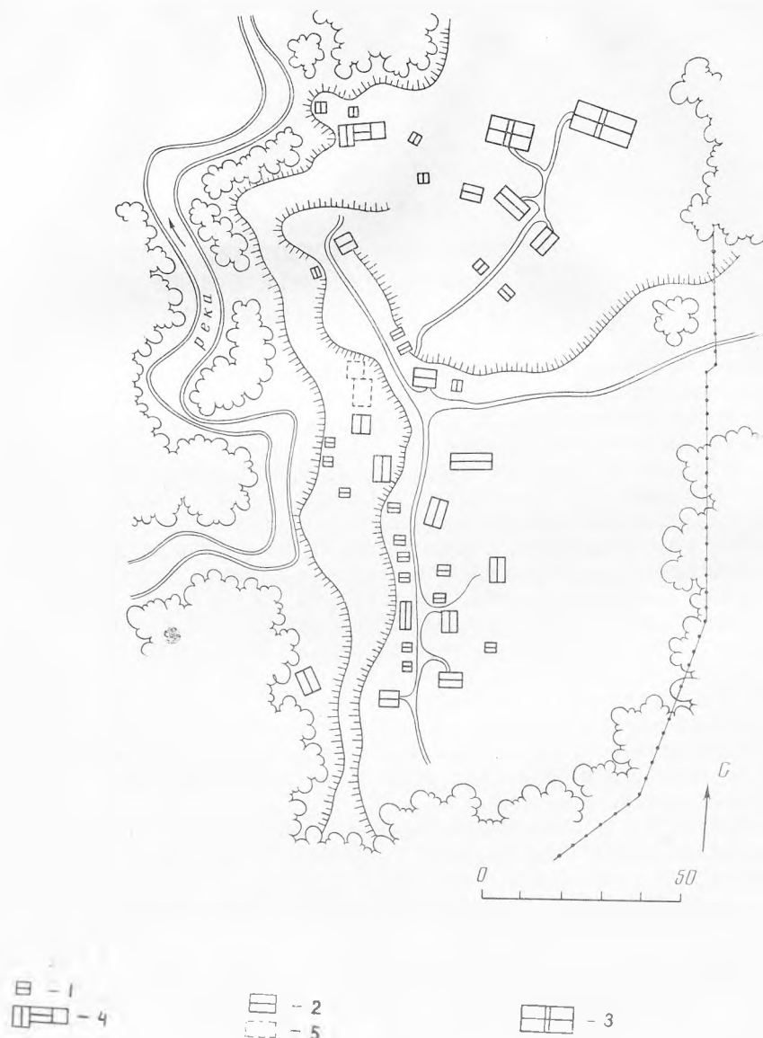
Рис. 1. Планировка сезонного поселения Хорнемская (р. Пинега): 1 — амбар; 2 — жилой дом; 3 — скотный двор; 4 — Г-образная связь дома и двора; 5 — не сохранившиеся постройки
