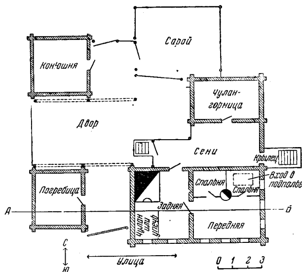
Рис. 6. План и разрез дома Ф. П. Елистратова, построенного в 1924 г. (с. Сосновый Солонец Куйбышевской обл.)
