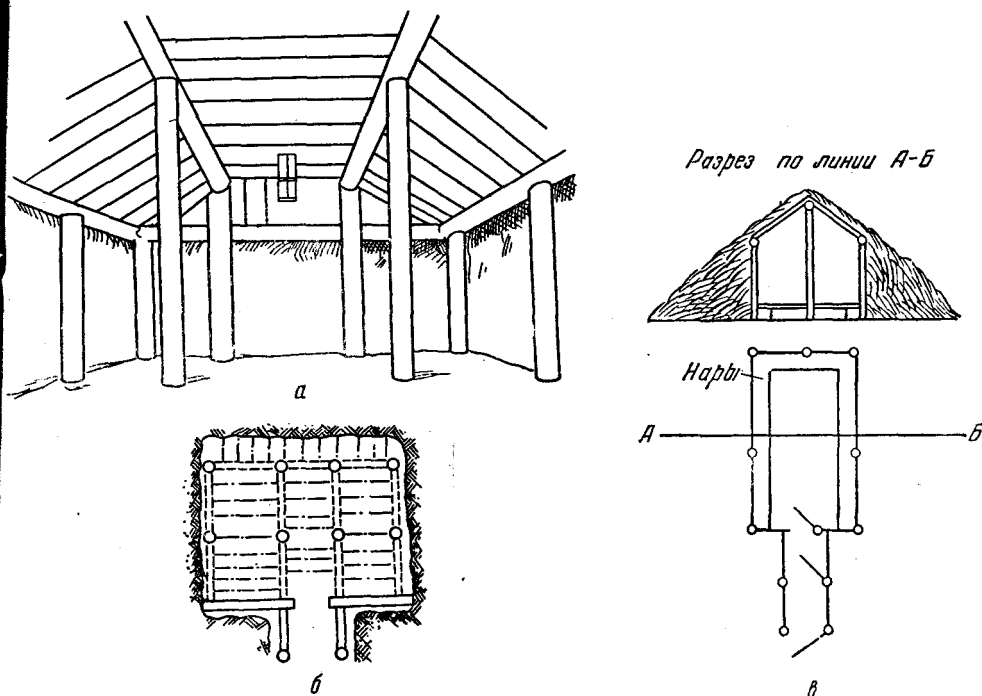
Рис. 7. Омшаники (дер. Вислая Дубрава Николо-Черемшанского р-на Ульяновской обл.): а, б — внутреннее устройство и план; в — разрез и план
