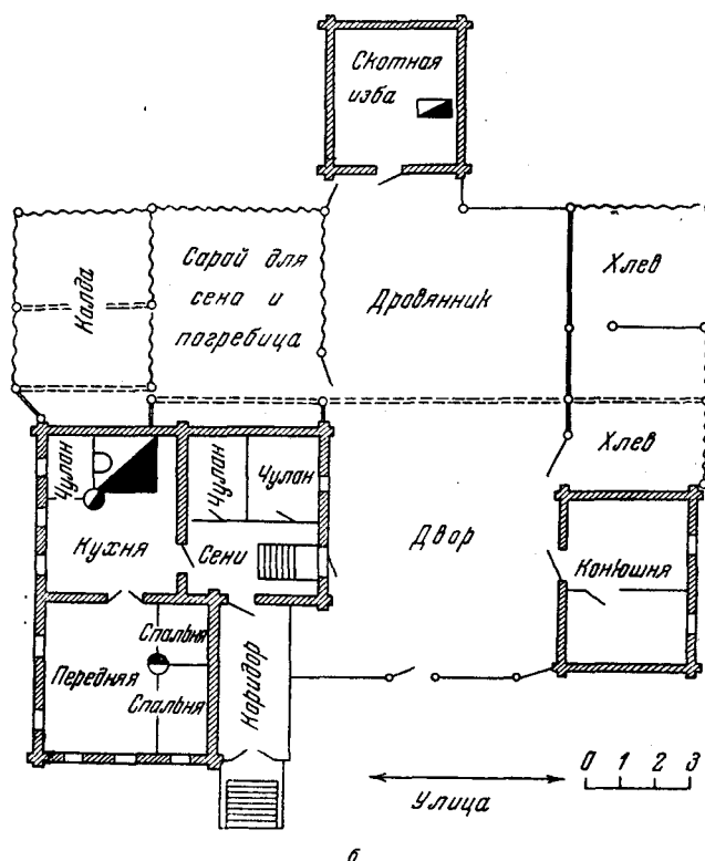
Рис. 3. Дом Ф. М. Пенькова, построенный в 1950—1951 гг: а — общий вид; б — план (д. Вислая Дубрава Николо-Черемшанского р-на Ульяновской обл.)
