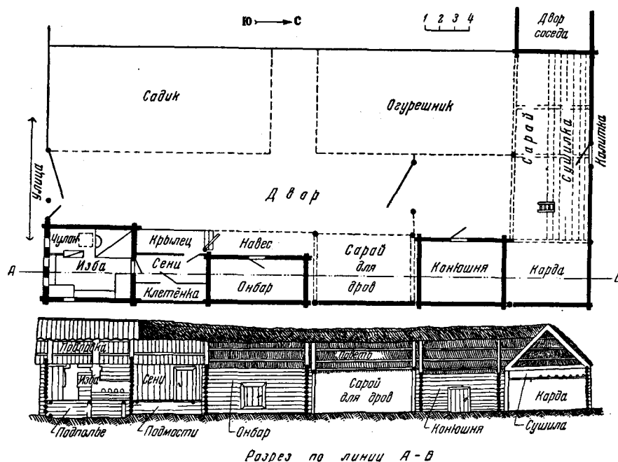
Рис. 4. План и разрез дома с двором В. Ф. Миронова, постройки 1926 г. (д. Кольцовка Вурнарского р-на Чувашской АССР)
