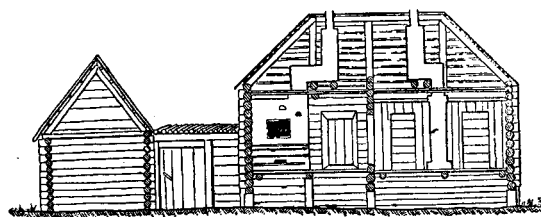
Разрез по линии А-Б
