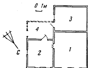
Рис. 3. Дом в селении Гермаб; а — внешний вид, б — план; 1, 2 — жилые комнаты, 3 — «коридор», 4 — веранда
