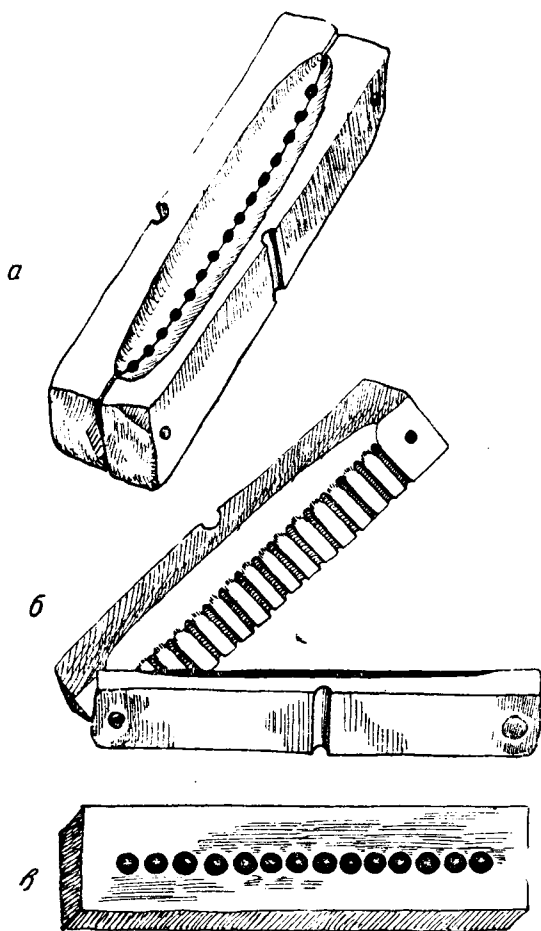
Рис. 4. а — общий вид литниковой системы: деревянный разъемный брусочек с общей литниковой чашей и 15-литниковыми каналцами; б — то же в раздвинутом виде; в — металлическая форма в виде пластинки с чашеобразными углублениями, являющимися формочками для отливки выпуклых свинцовых бляшек (см. рис. 2, е)
