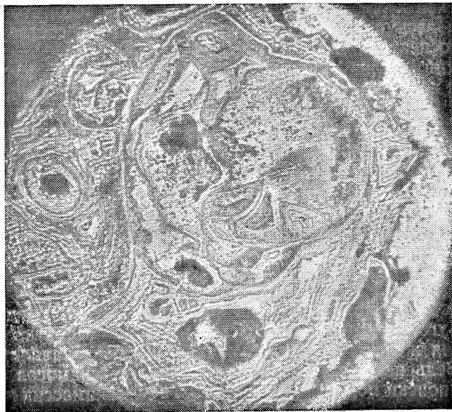
Рис. 2. Микроструктура окарины \text{Fe}_2\text{O}_3 при увеличении 100
