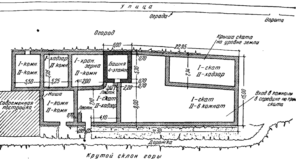
Рис. 1. План галуана Икаевых, Сев. Осетия, Архонское ущелье, сел. Архон. Обмер архит. С. С. Кригер и Н. Ф. Такоевой, 1947 г.
