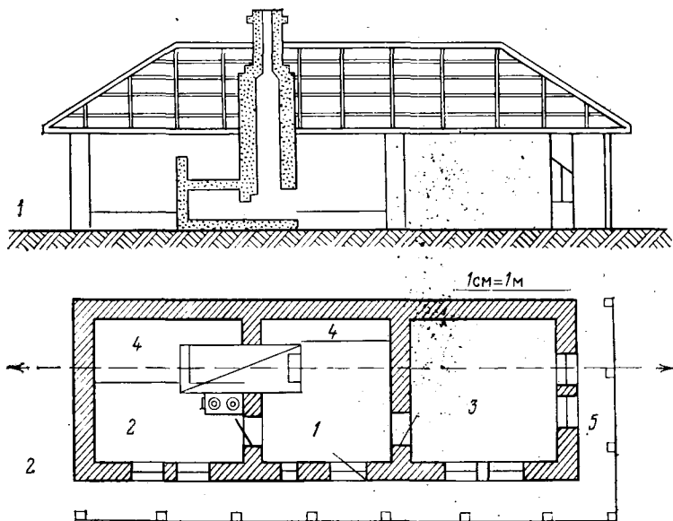
Рис. 4. Внутреннее устройство дома, конца XIX — начала XX в. в с. Жовтнево Болградского р-на Одесской обл. (разрез и план): 1 — помещение типа сеней, где находятся устье печи, очаг и прямой дымоход над ними; 2 — жилая комната, куда выходит корпус печи; 3 — парадная комната; 4 — глинобитное возвышение «пат»; 5 — открытая галерея. Чертеж В. И. Агафонова, 1969 г.
