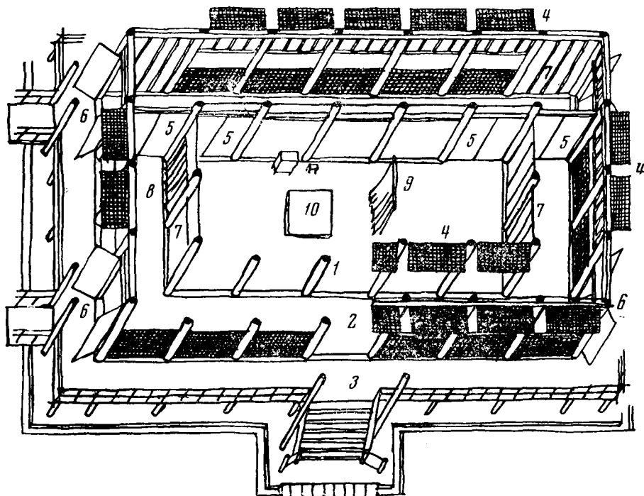
Рис. 7. Здание типа синдзэн: 1—мойя; 2—коридор хисаси; 3—терраса суноко; 4—подъемные и съемные перегородки ситомидо; 5—раздвижные двери; 6—двухстворчатые двери; 7—бамбуковый занавес сударэ; 8—занавес из ткани; 9—переносная ширма кито; 10—маты татами
