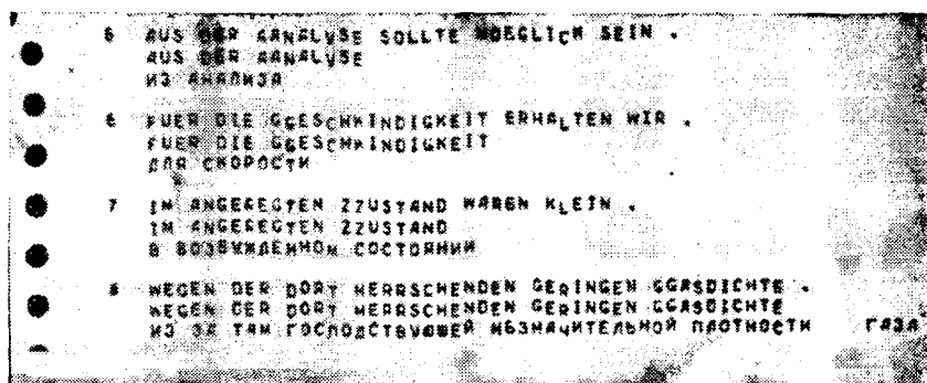
Рис. 11. Перевод на ЭВМ «Минск-22» немецких именных групп с помощью обращения к типовому контексту. Авторы программы А. В. Зубов и А. Н. Шарада (минская группа «Статистика речи»)
