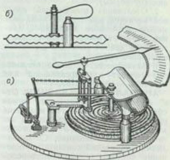
Механизм анероида. а — общий вид, б — вертикальный разрез коробки.
