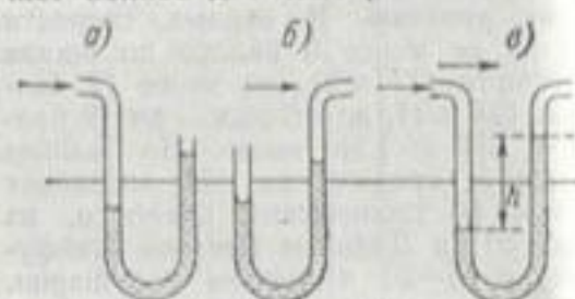
Трубка Пито.
