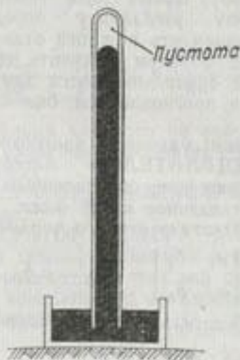
Опыт Торричелли. Принцип ртутного барометра.
