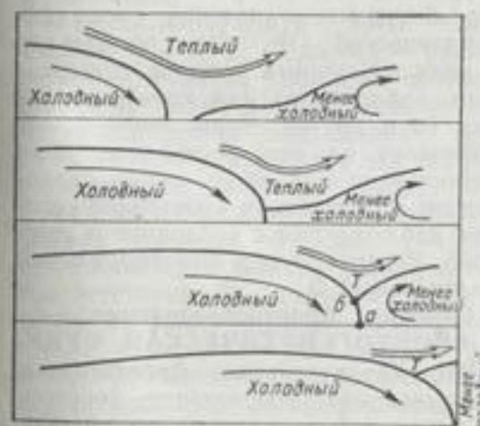
Образование холодного фронта окклюзии. а — нижний холодный фронт, б — верхний теплый фронт, аб — поверхность окклюзии.
