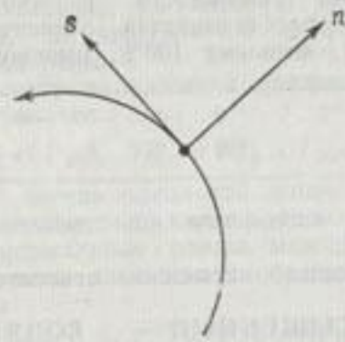
Натуральная система координат.
