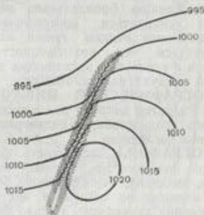
Орографические изобары (волнистые линии).
