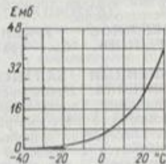
Зависимость упругости насыщения от температуры.
