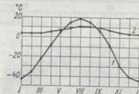
Годовой ход температуры воздуха под широтой 62^{\circ} в морском и континентальном климате. 1 — Якутск, 130^{\circ} в. д., 2 — Торсхавн, 7^{\circ} з. д.
