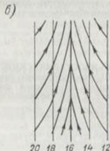
Изогоны ветра и соответствующие им линии тока. Числами указано направление ветра на каждой изогоне (32 — север, 16 — юг). Линии тока сходятся к точке (а) и к линии (б).
