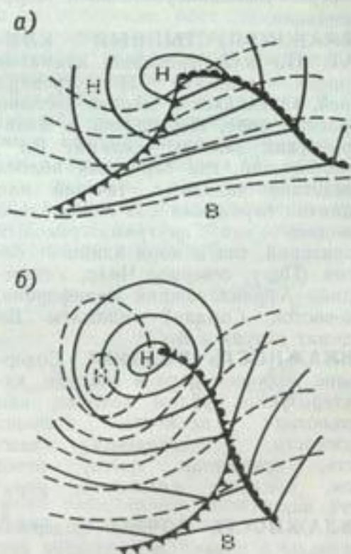
Фронты и изобары во внетропическом циклоне у земной поверхности и в верхней тропосфере. а — молодой циклон, б — окклюзированный циклон.
