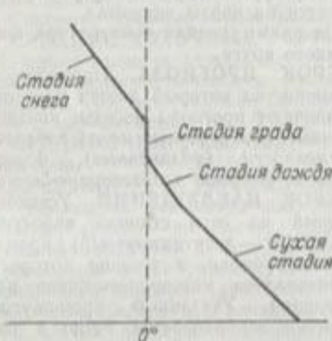
Стадии адиабатического процесса.
