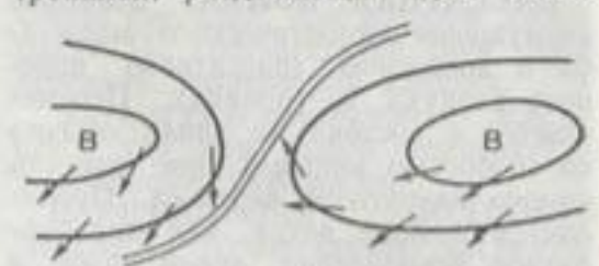
Пассатный фронт.
