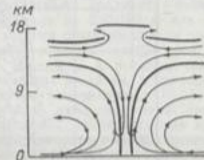
Вертикальная циркуляция в тропическом циклоне. Жирные линии — тропопаузы и граница глаза бури.
