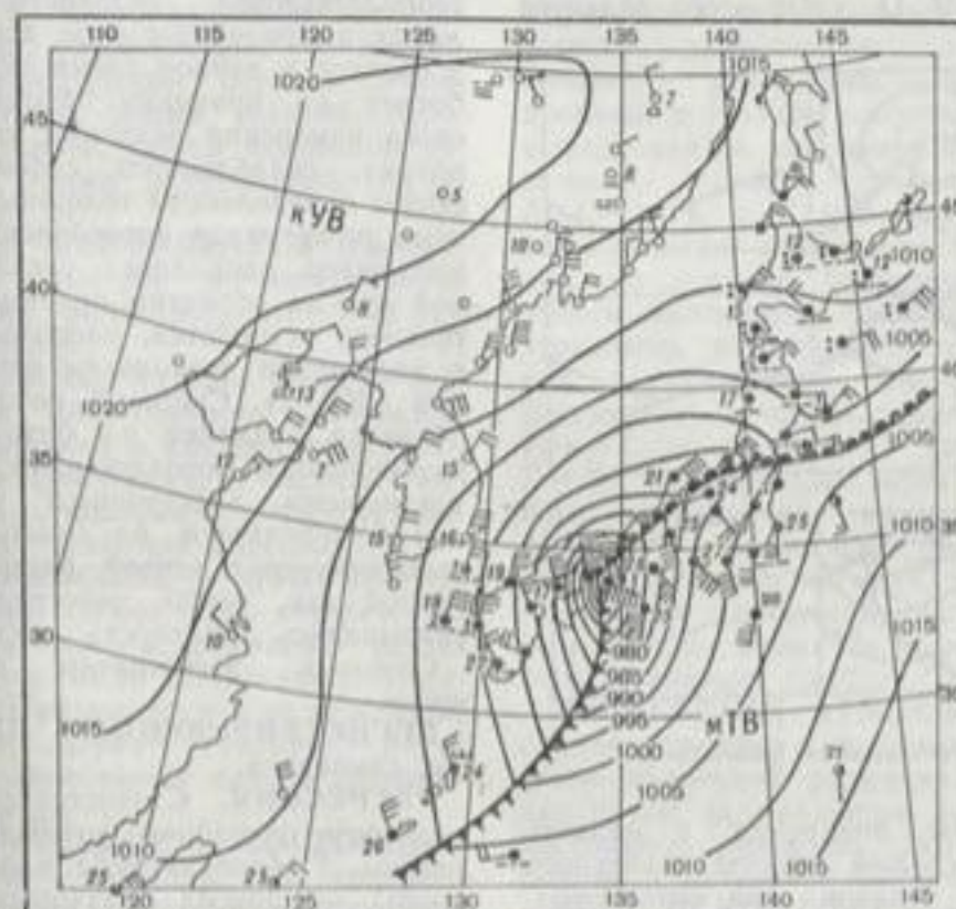
Регенерации тайфуна. 21 сентября 1934 г., утро.
