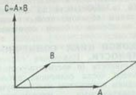
Векторное произведение.
