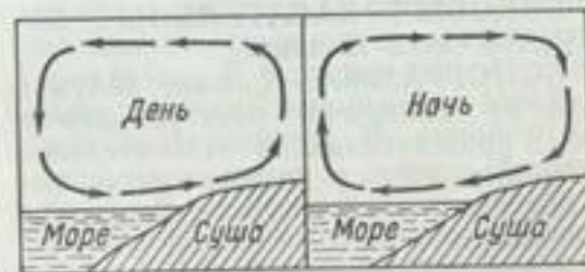
Схема бризов.
