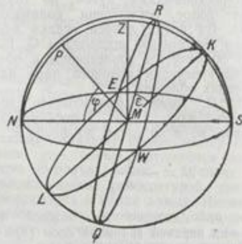
Основные точки и круги небесной сферы.
