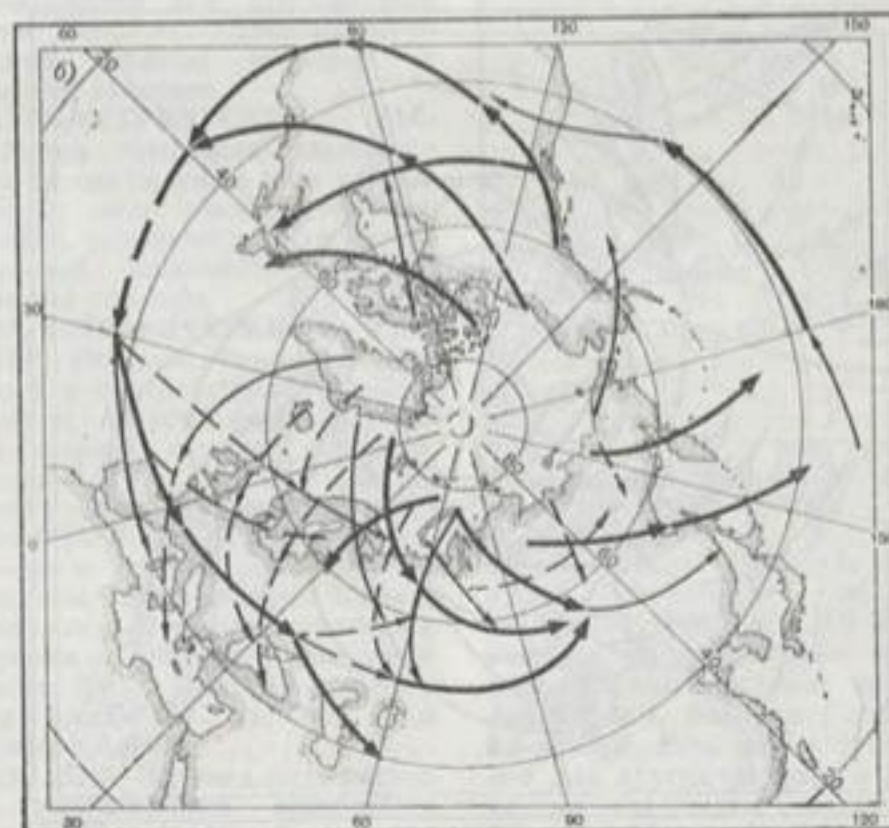
Пути антициклонов в северном полушарии в январе (а) и в июле (б).
