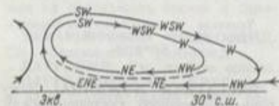
Пассатная циркуляция. Основное и верхнее пассатные течения, пассатная инверсия (прерывистая линия), антипассаты. Буквы — направления ветра.
