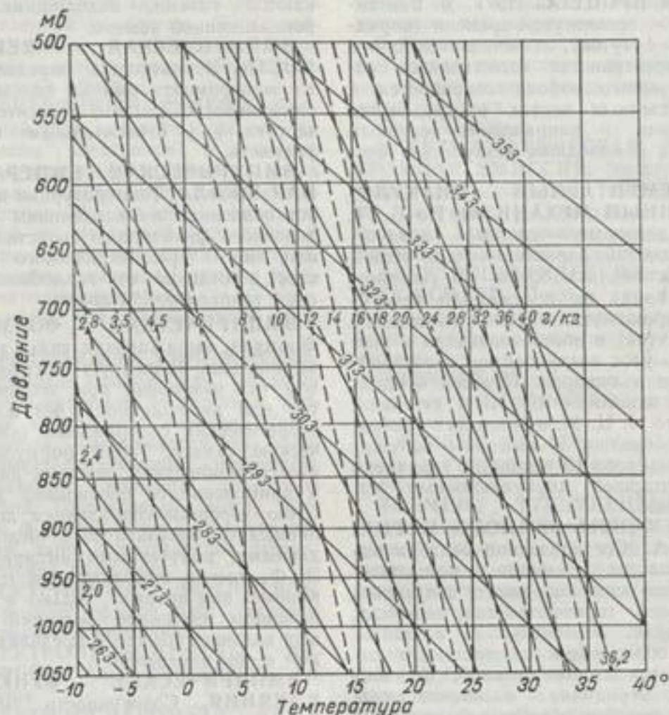
Эмаграмма.
