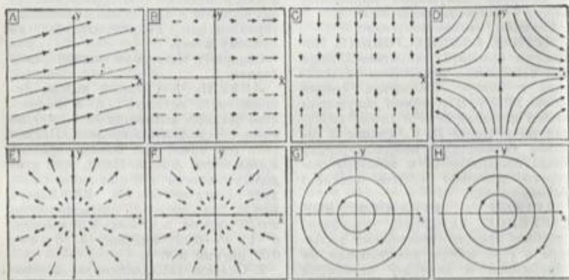
Составляющие линейного поля движения.
