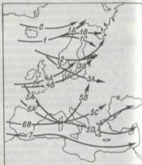
Основные пути циклонов в Европе по Ван-Беберу.
