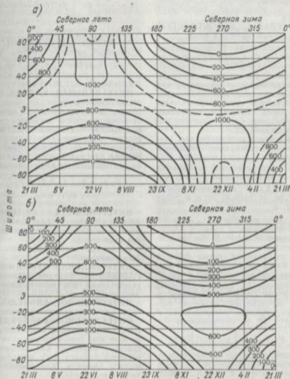
Инсоляция (в кал/см²) земной (горизонтальной) поверхности за сутки в отсутствие атмосферы (а) и при коэффициенте прозрачности 0,7 (б).
