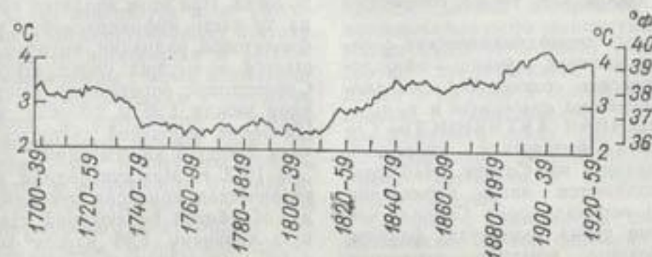
Современное потепление. Вековой ход температуры в центральной Англии в январе по 40-летним скользящим средним.
