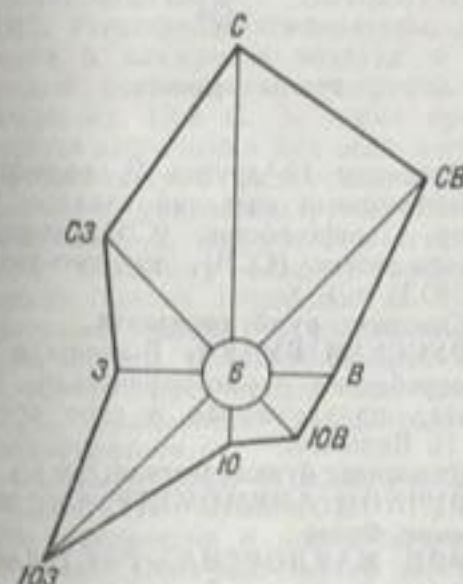
Роза ветров.
