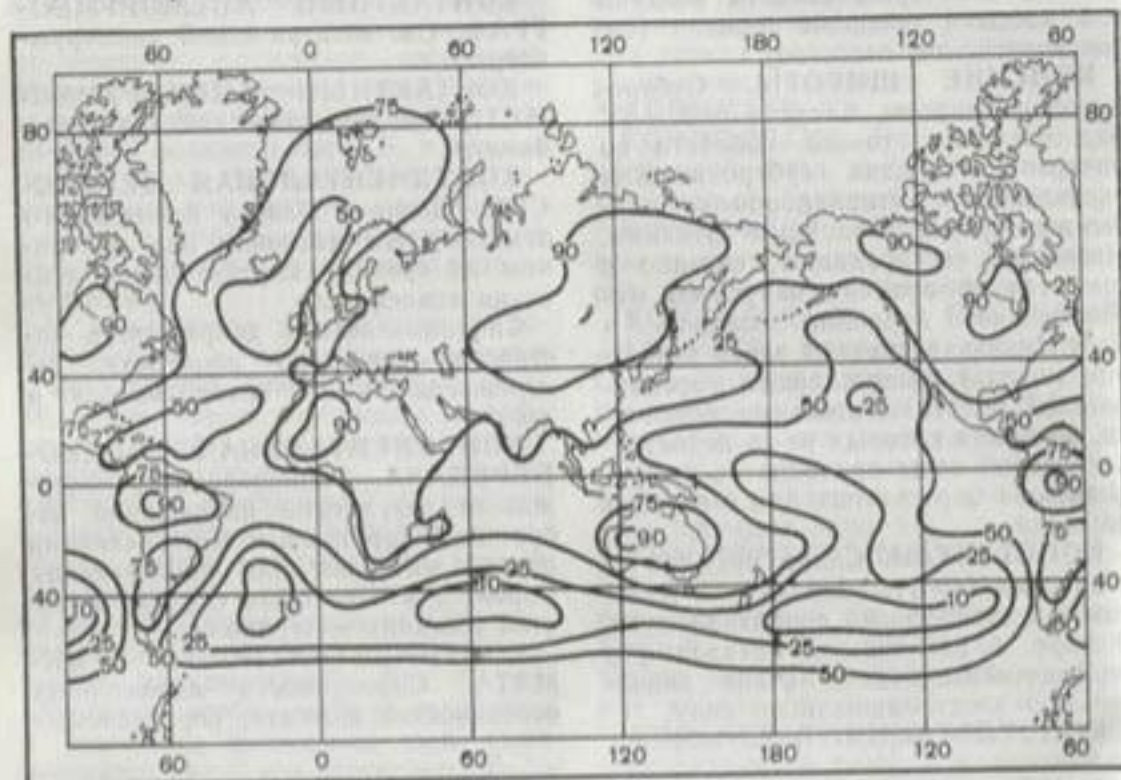
Распределение индекса континентальности С. П. Хромова по земному шару.
