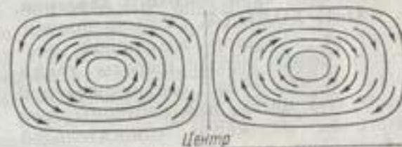
Ячейки конвекции. Линии тока в вертикальном разрезе.
