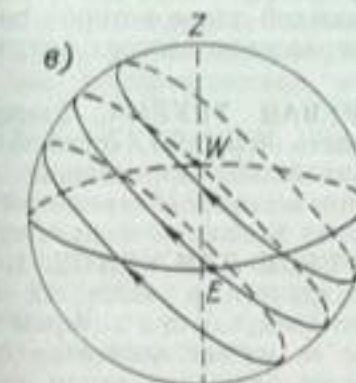
Видимое движение солнца. Суточное движение солнца на экваторе (а), внутри тропиков (б) и в умеренных широтах (в) в дни солнцестояний (крайние траектории) и равноденствий (средние траектории). Z — зенит, W, E — точки запада и востока.
