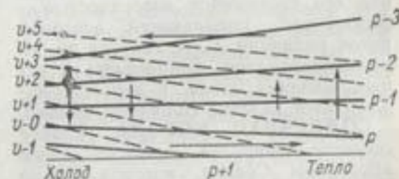
Изобаро-изостерические солениды. Стрелками указано направление связанной с ними циркуляции.
