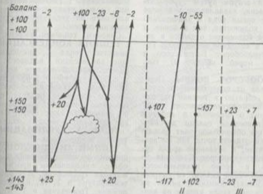
Тепловой баланс Земли, атмосферы и земной поверхности. I — коротковолновая радиация, II — длинноволновая радиация, III — перераспределение.
