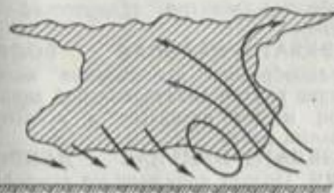
Движение воздуха при шквале.
