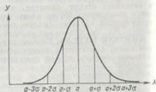
Нормальная кривая распределения.
