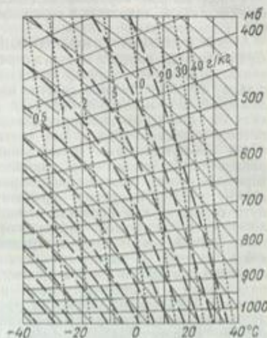
Аэрограмма. Сплошные наклонные линии — сухие адибаты, пунктирные — влажные адибаты, пунктирные — изогаммы удельной влажности для состояния насыщения.
