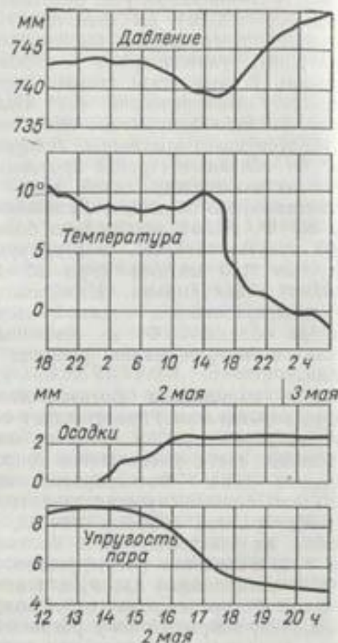
Изменение метеорологических элементов при прохождении холодного фронта в Москве 1—2 мая 1929 г.
