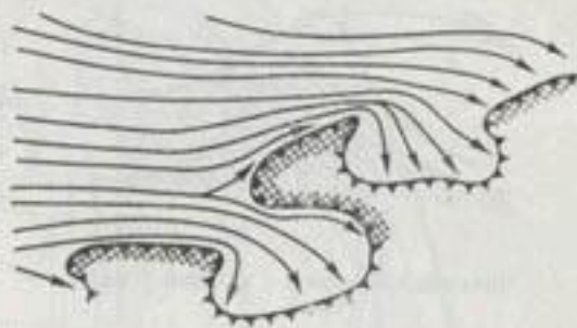
Орографическая окклюзия. Линии тока в холодном воздухе и холодный фронт у орографических препятствий.
