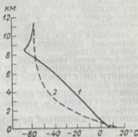
Теоретическое распределение температуры с высотой. 1 — при конвективном равновесии в тропосфере и лучистом в стратосфере, 2 — при лучистом равновесии.
