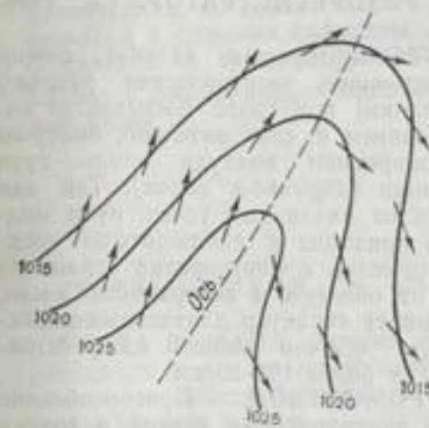
Гребень. Стрелки — приземный ветер.
