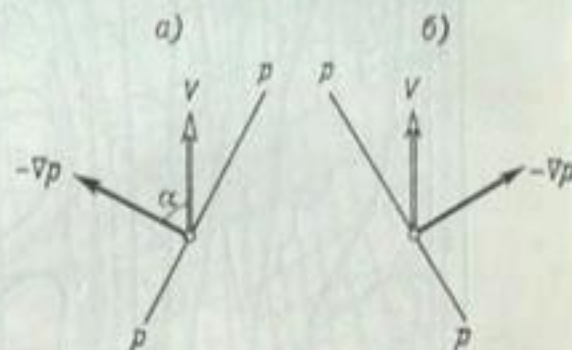
Барический закон ветра.
