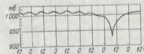
Запись барографа при прохождении тропического циклона.
