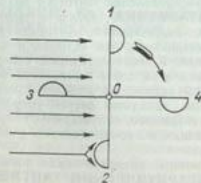
Анемометрические полушария. Схема, вид сверху. Стрелки — направление ветра, оперенная стрелка — направление вращения полушарий.
