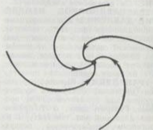
Точка сходимости.
