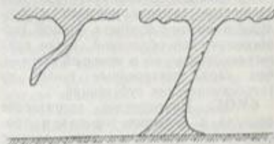
Смерч.
