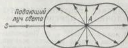
Индикатриса молекулярного рассеяния по Релею.
