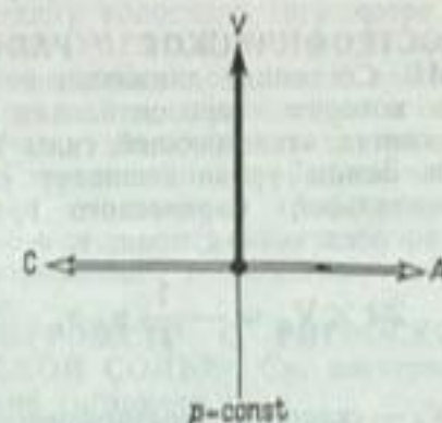
Геострофический ветер.
