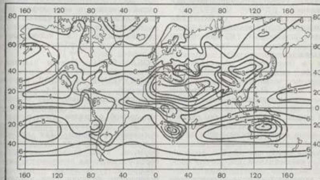
Средняя годовая облачность в десятых долях.
