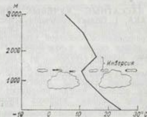
Типичное распределение температуры воздуха с высотой в зоне пассатов.
