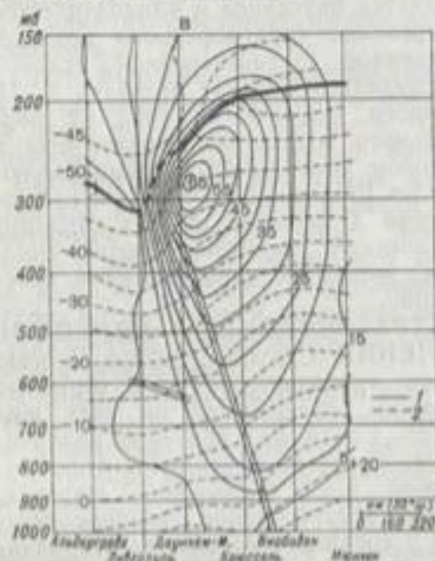
Струйное течение над полярным фронтом в Европе 18 июня 1963 г. 1 — изотопы в м/с, 2 — изотермы в градусах.
