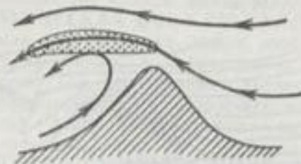
Чечевицеобразное облако над горой.
