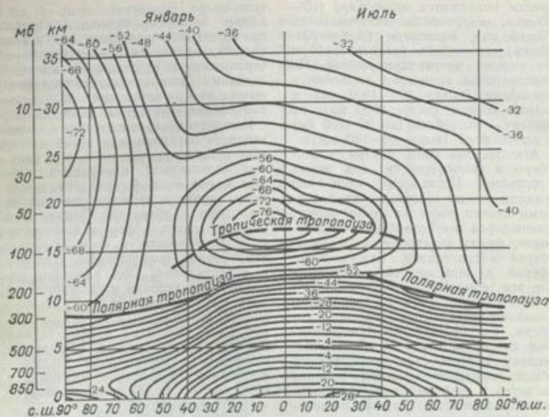
Среднее распределение температуры с высотой в северном полушарии зимой и летом. Жирная линия — тропопавза.
