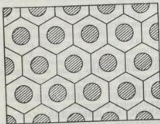
Схема ячеек Бенара.
