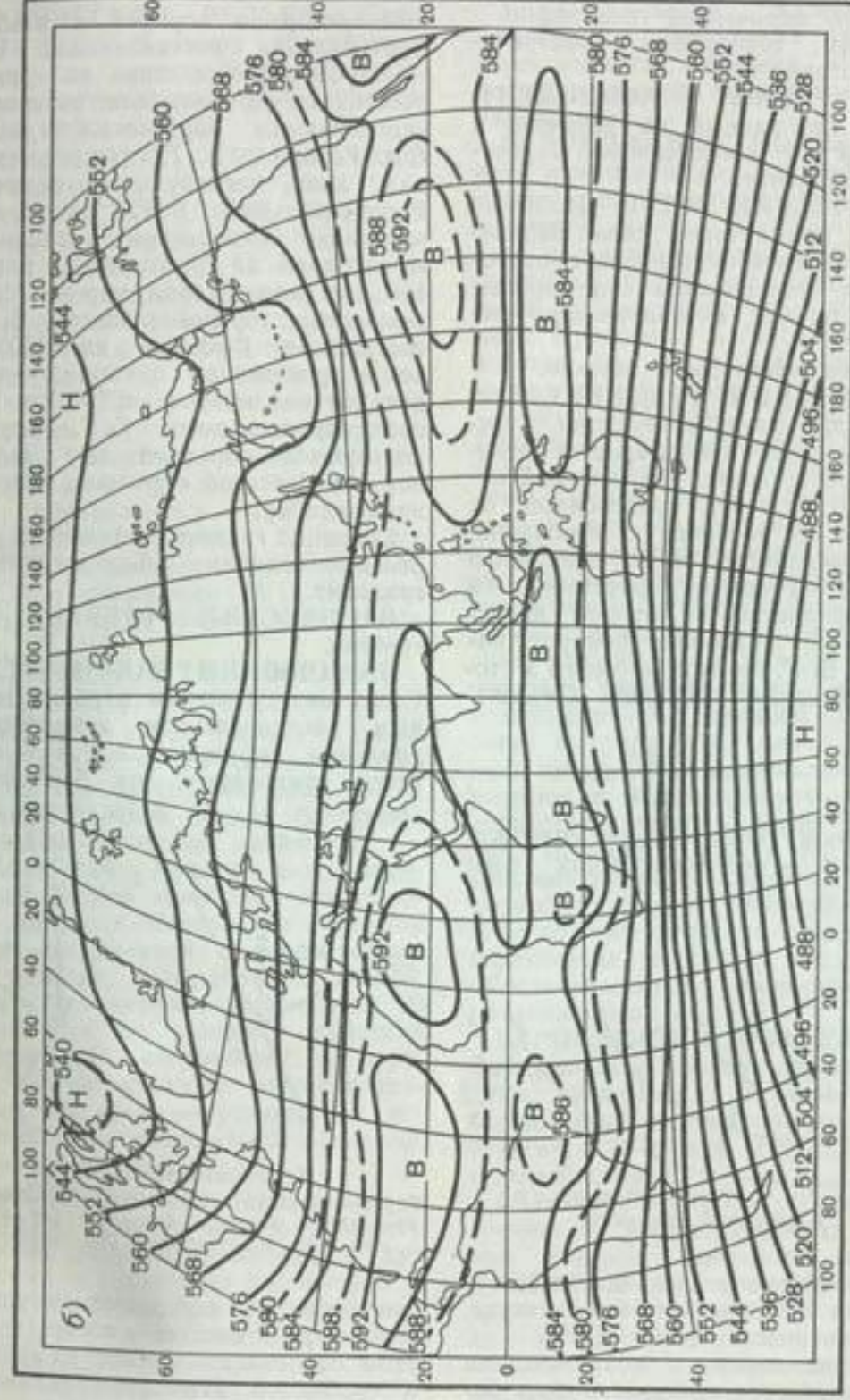
Многолетние средние карты абсолютной топографии поверхности 500 мб за декабрь (а) и за июль — август (б). Высоты в геопотенциальных декаметрах.
