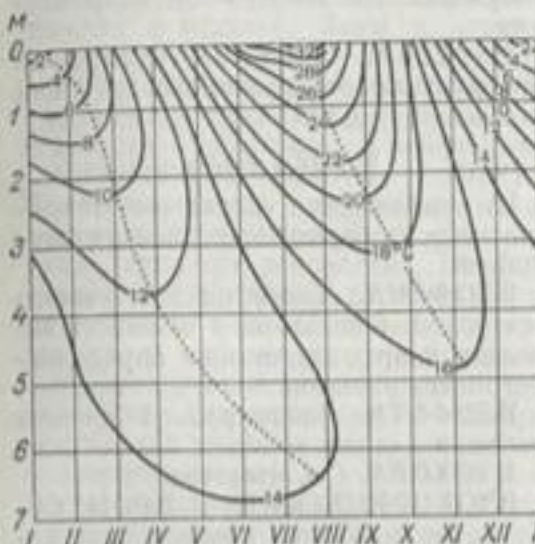
Изовагеты температуры почвы в Тбилиси
