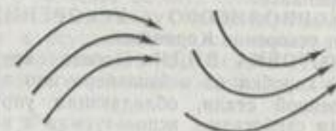
Конфлюэнция.
