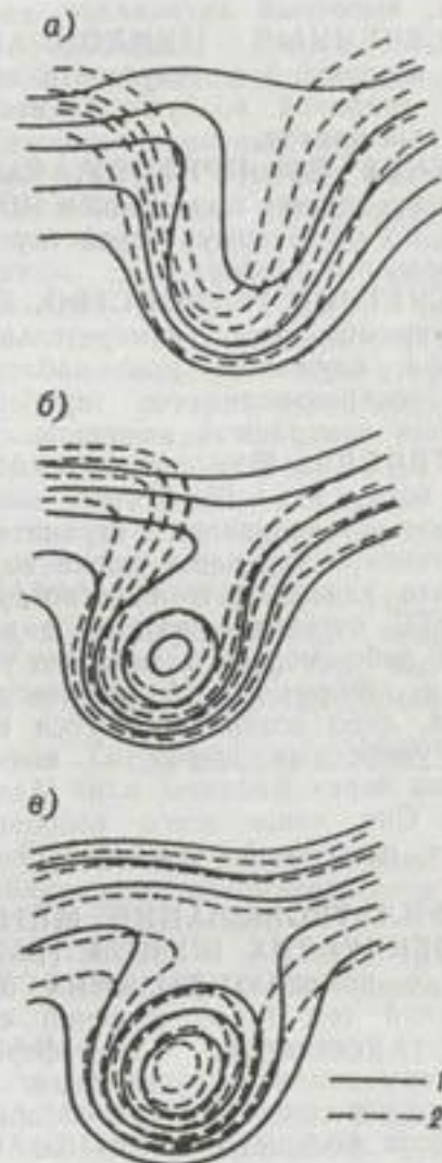
Образование высокого холодного циклона в результате отсечения.
