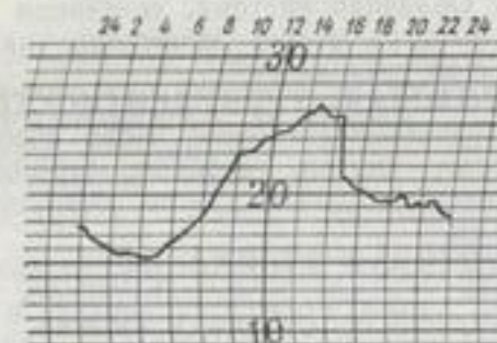
Грозный нос и ход температуры при грозе
