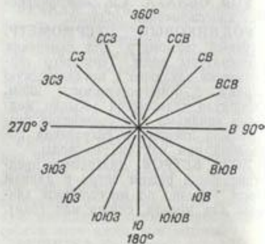
Румбы горизонта.
