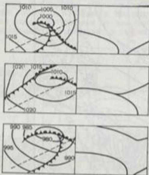
Регенерация циклона.
