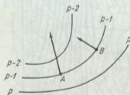
Барический градиент.
