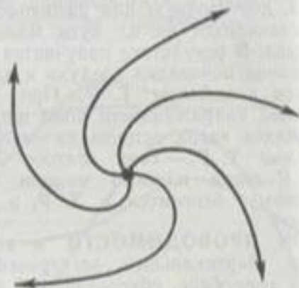
Точка расходимости.
