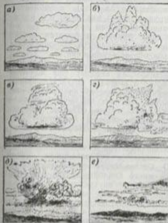
Облака конвекции.
