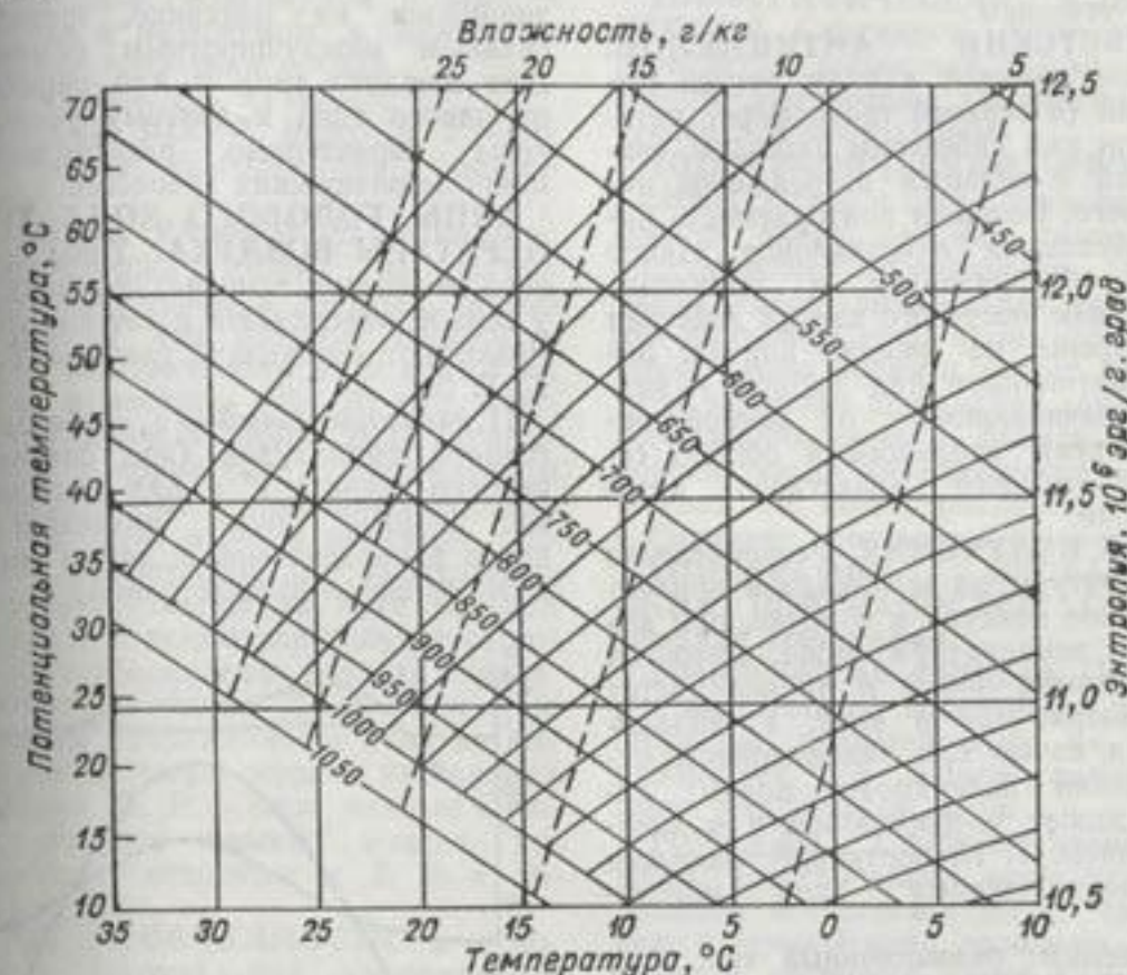
Тетраграмма.
