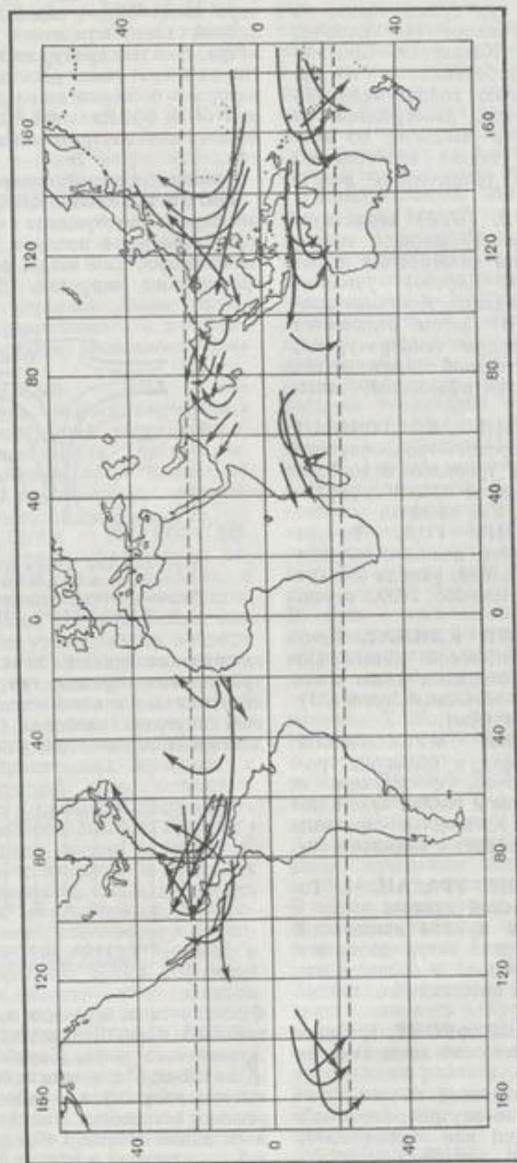
Основные пути тропических циклонов.
