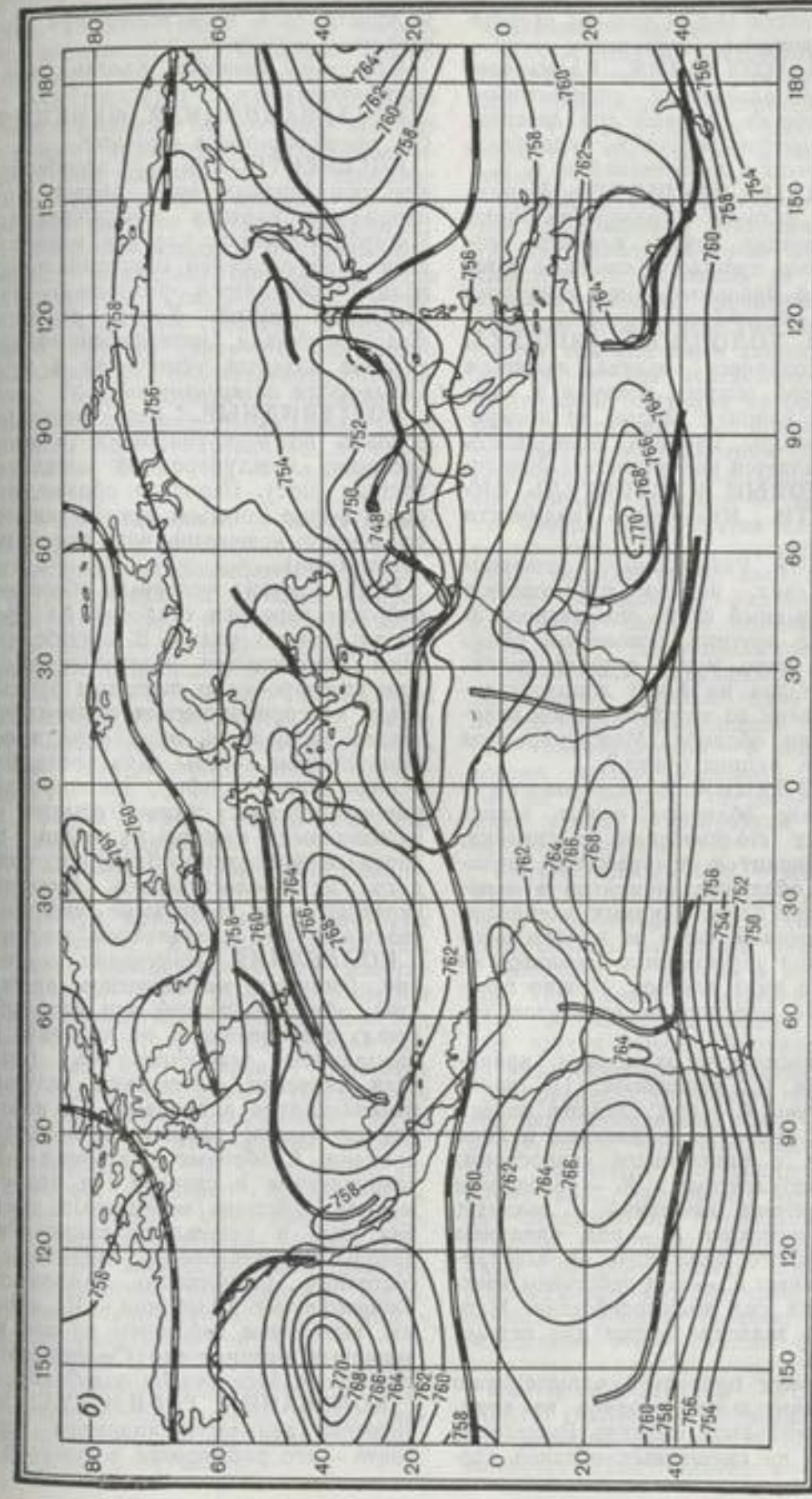
Климатологические фронты по С. П. Хромову в январе (а) и в июле (б). 1 — арктический, 2 — полярный, 3 — пассатный, 4 — тропический (антропогенная зона конвергенции).
