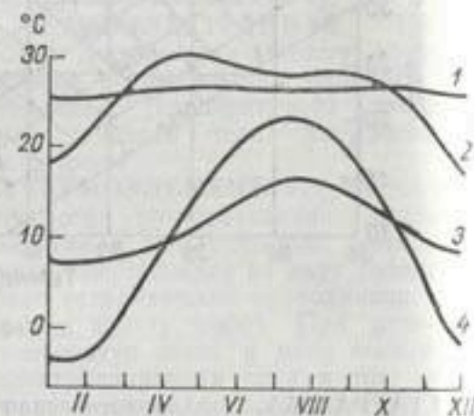
Некоторые типы годового хода температуры воздуха.
