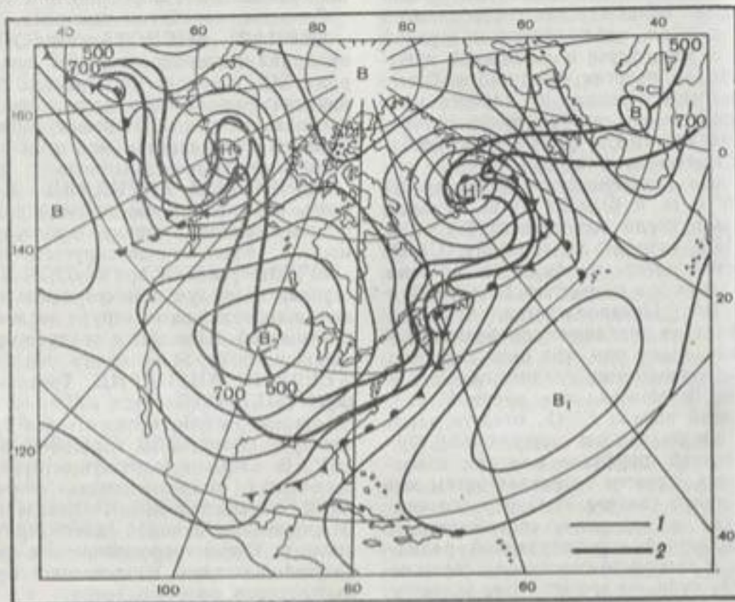
Две серии циклонов на синоптической карте. 1 — изобары на уровне моря, 2 — положение полярного фронта на изобарических поверхностях 700 и 500 мб, линии с орнаментом — фронты на земной поверхности, H1 — центральный циклон, B1 — субтропический антициклон, B2 — заключительный антициклон.
