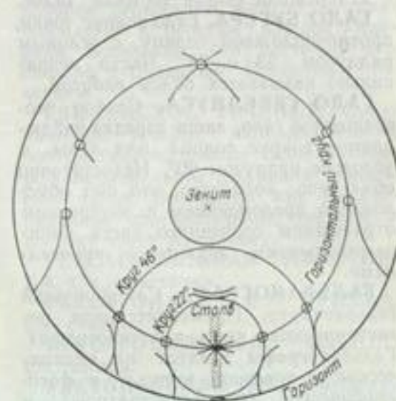
Основные формы гало.
