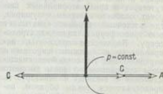
Антибарический ветер.
