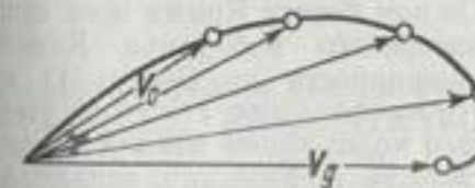
Спираль Экмана.
