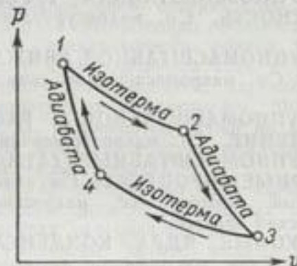
Круговой процесс Карно.
