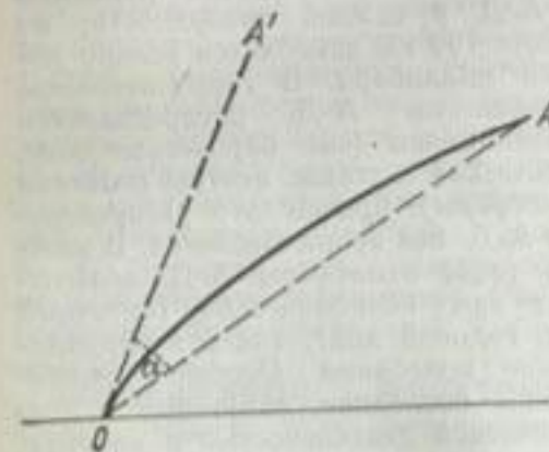
Атмосферная рефракция. Сплошная линия АО — путь луча от предмета к наблюдателю; прямая ОА — истинное направление на предмет; ОА' — направление, в котором виден предмет; \alpha — угол рефракции.
