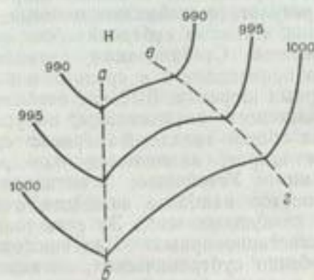
Антициклоническая кривизна изобар (между линиями а и б).
