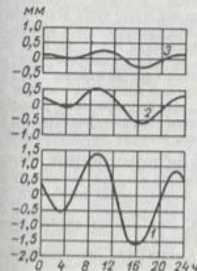
Суточный ход атмосферного давления. 1 — Сингапур, 2 — Париж, 3 — Упсала.
