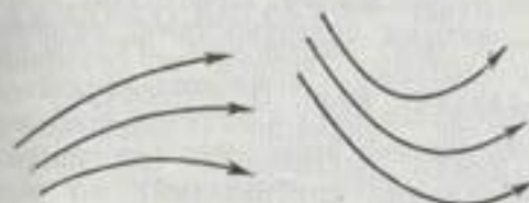
Дифлюэнция.
