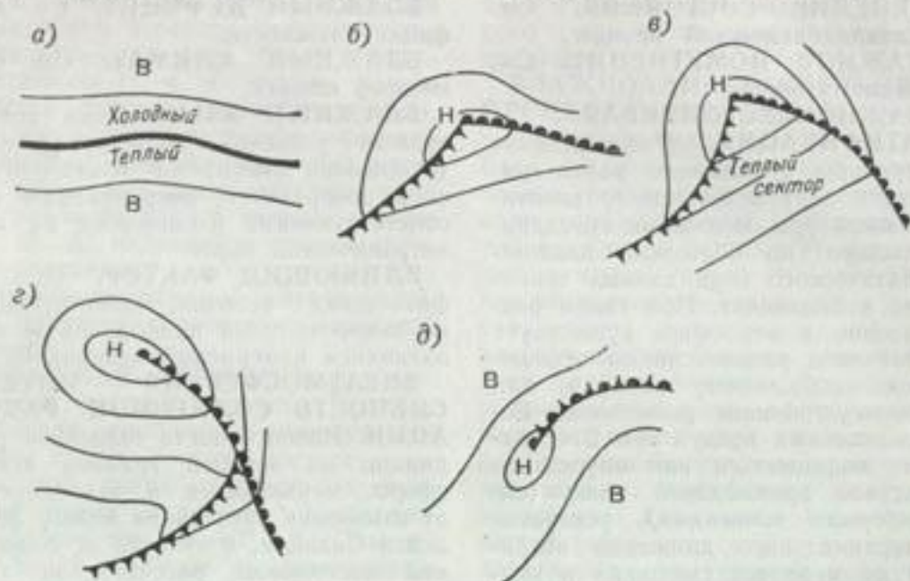
Развитие внетропического циклона на фронте. Тонкие линии — изобары; а — волна; б, в — молодой циклон; г, д — окклюзированный циклон.
