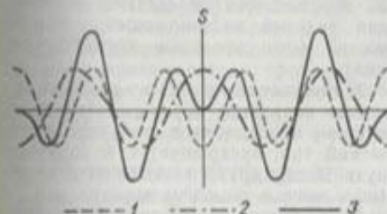
Точка симметрии.
