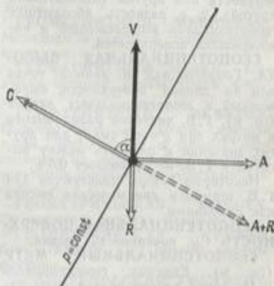
Геотриптический ветер. G — сила барического градиента, A — отклоняющая сила вращения Земли, R — сила трения, V — скорость ветра.
