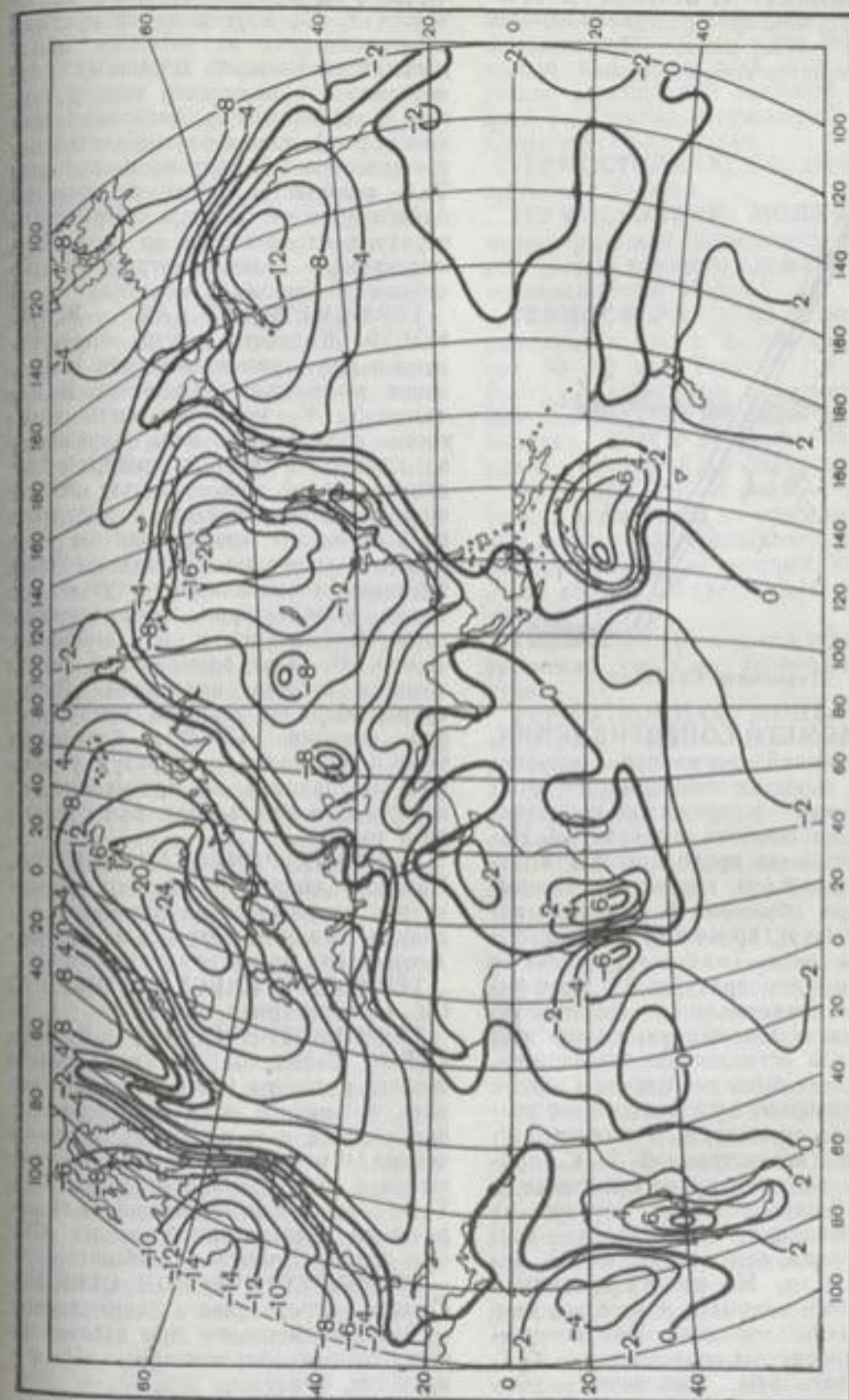
Термозвездочки кивары на уровне моря. Разности между средней температурой места и средней температурой широтного круга в январе за многолетний период.
