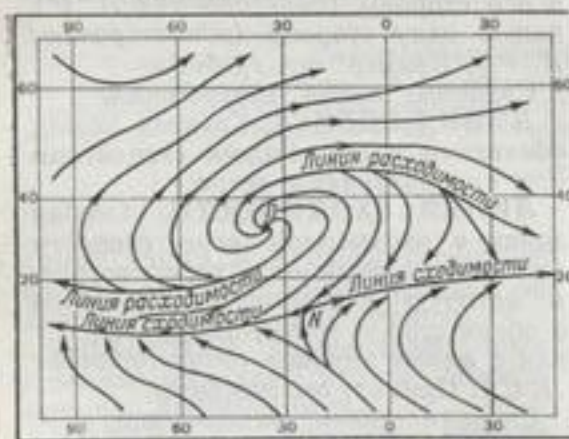
Линии тока. Схематизированное поле преобладающих ветров в области азорского антициклона в июле. D — точка расхождимости, N — нейтральная точка.
