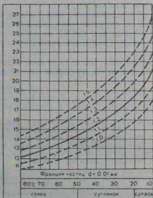
Рис. 5. График определения нормативных расстояний между дренами в зависимости от глубины их закладки и механического состава связных почв (по данным Ц. Н. Шкинника)
