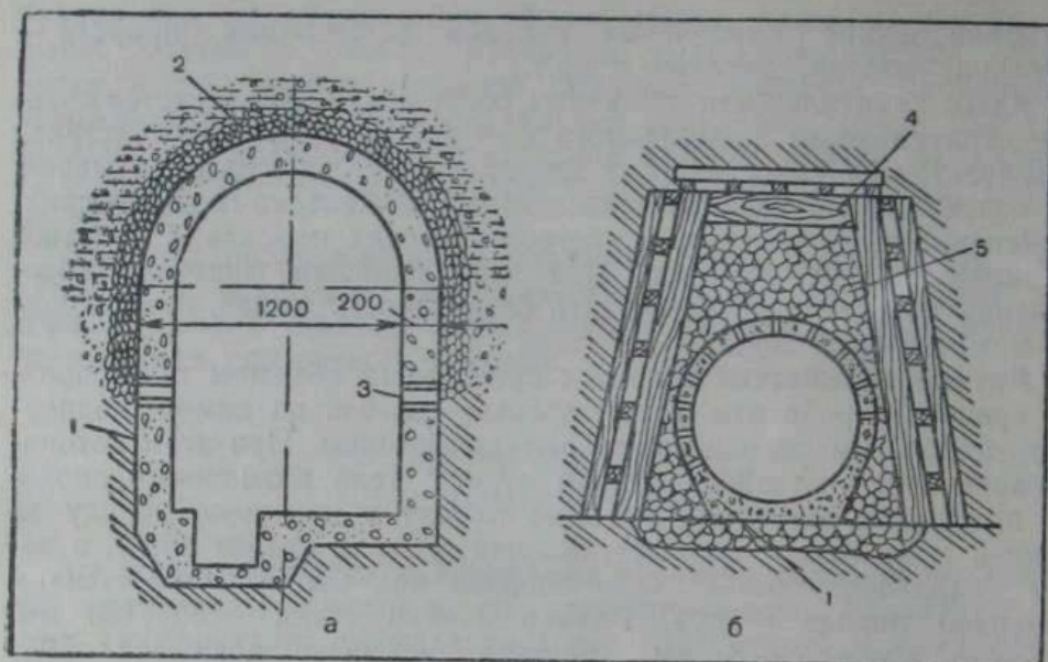
Рис. 55. Поперечные сечения дренажных штолен:
