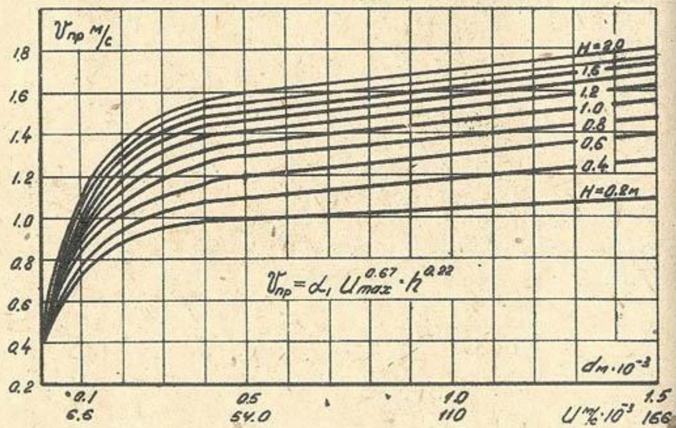
Рис.3. Кривые зависимости V_{кр} = f(W_{max}) для разных глубин потока.
