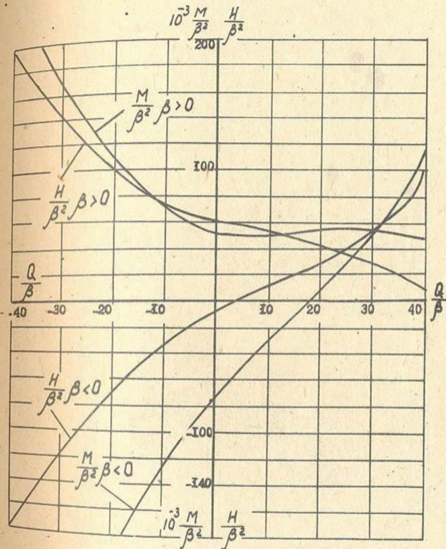
Рис. 1. Насос В 24 25/40-1
