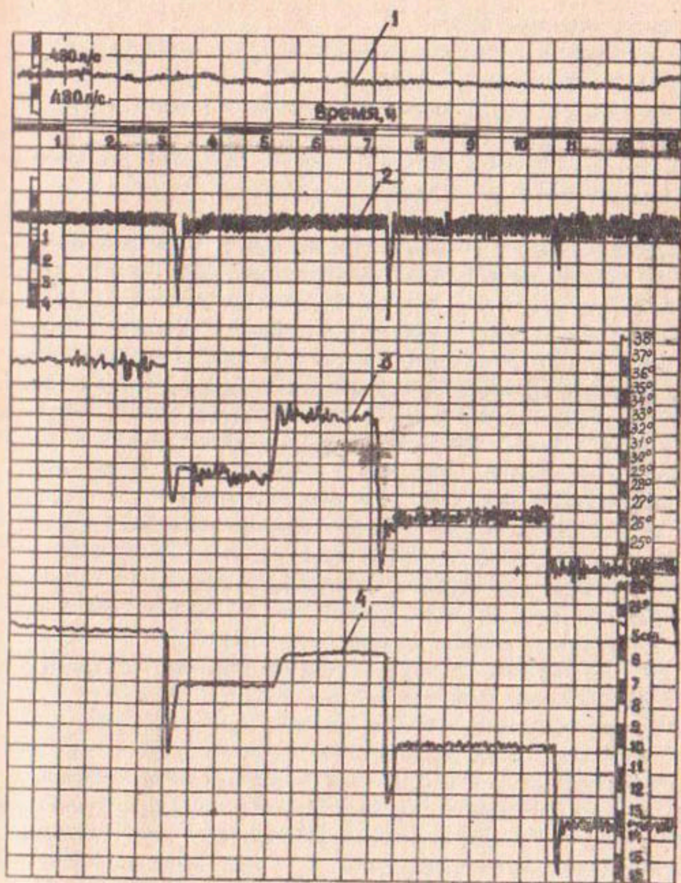
Рис.3. Диаграмма колебаний горизонтов воды верхнего и нижнего бьефов и изменений угла открытия затвора во времени: 1- колебания подаваемого на модельную установку расхода; 2- изменение уровня воды в верхнем бьефе; 3- изменение уровня воды в нижнем бьефе; 4- изменение угла открытия затвора
