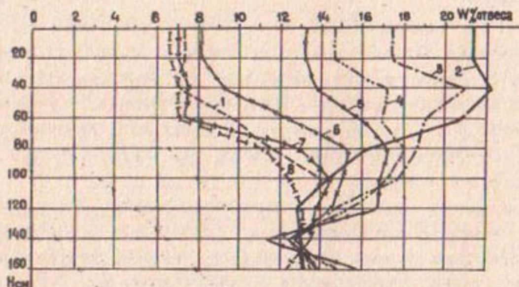
Рис.2. Динамика влажности почвогрунтов в межполивной период 1 - перед поливом; 2 - первый день после полива; 3 - третий день после полива; 4 - пятый день после полива; 5 - седьмой день после полива; 6 - десятый день после полива; 7 - пятнадцатый день после полива; 8 - двадцатый день после полива
