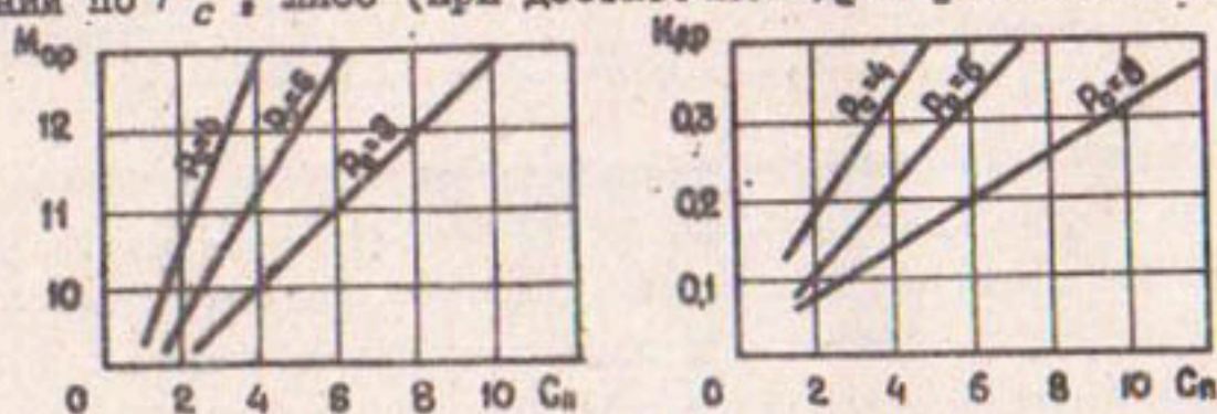
Рис. 2. Зависимость оросительной нормы ( M_{ор} тыс. м 3 /га) и доли дренажного стока ( K_{др} ) от минерализации поливной воды ( C_{II} г/л)
