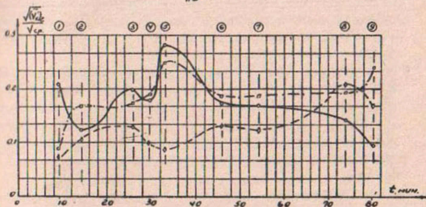
Рис.3 "а" – график изменения локальных осредненных скоростей в участках I–9 хронограммы осредненных скоростей русла динамического равновесия (рис.2); "б" – график изменения интенсивностей турбулентности потока в участках I–9 хронограммы осредненных скоростей русла динамического равновесия (рис.2). Условные обозначения те же, что и в рис.1 и 2.
