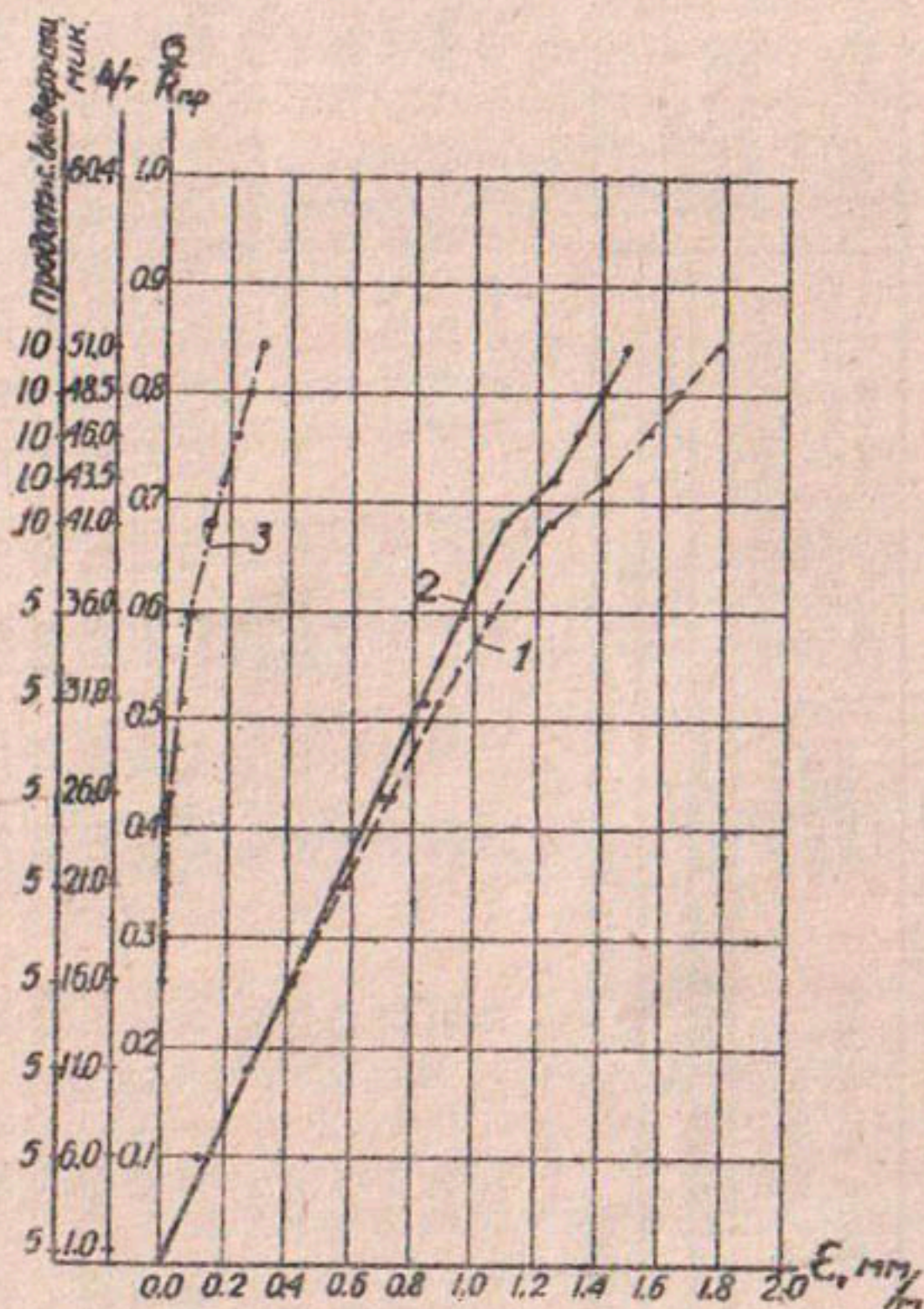
Рис.3 График зависимости средних деформаций ядра К-12 от нагрузки (Ядро испытано 14.01 67 г. в возрасте 25 месяцев, N_p = 60,4 т, R_{\sigma} = 526 кг/см 2 , R_{\kappa\psi} = 700 кг/см 2 , \gamma_6 = 2,31 при \sigma = 0,5 R_{\sigma p} = 263 кг/см 2 , \epsilon = 0,82 мм/м, = 321000 ): 1- деформации полные; 2- упругие; 3 - пластические.
