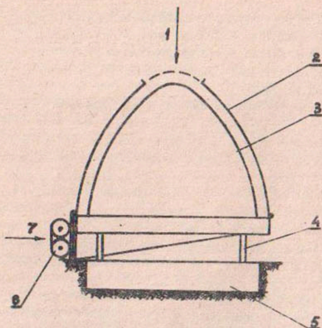
Рис. I Схема стенда с поперечной горизонтально направленной вибрацией формы:
