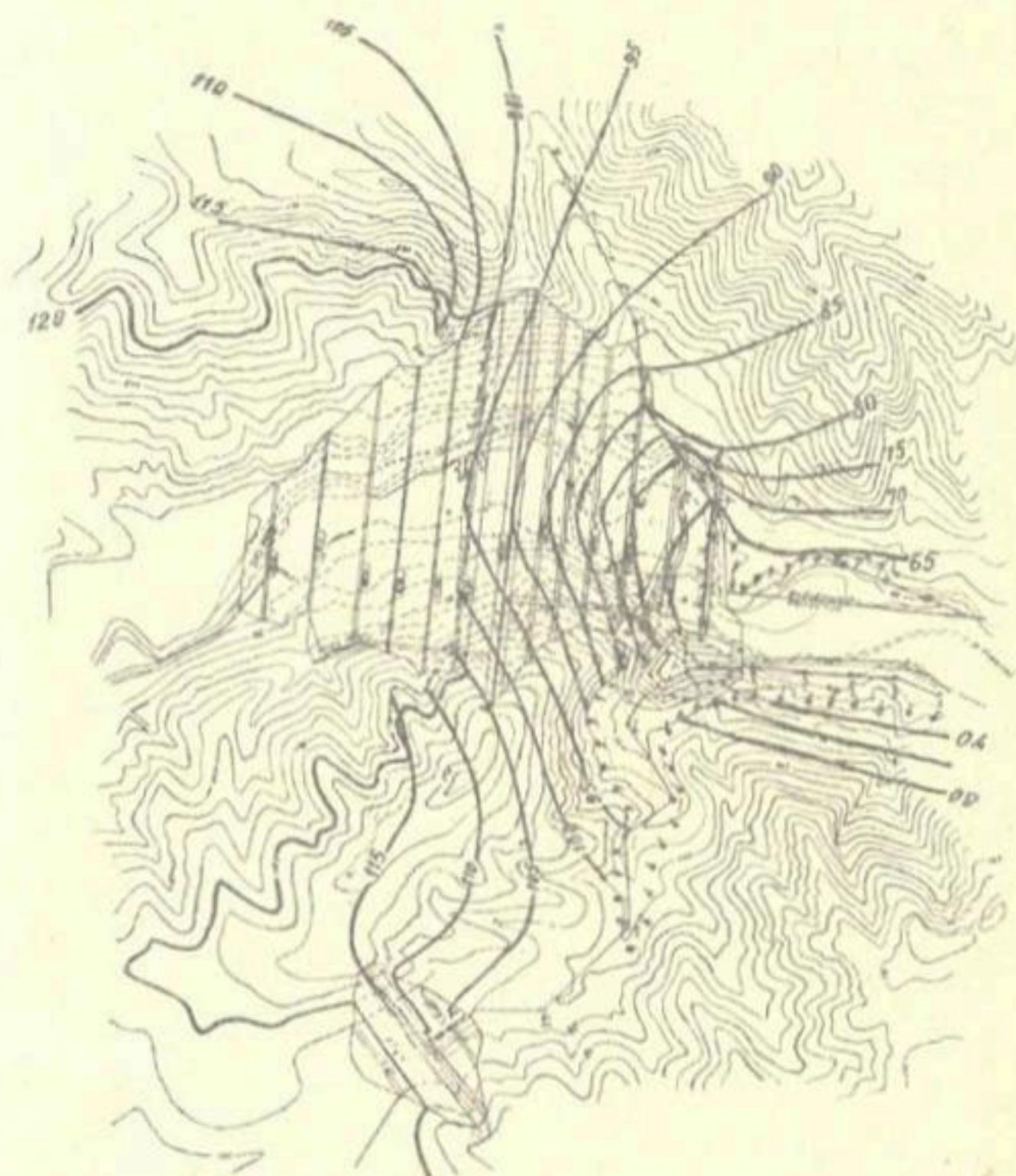
Рис.2.План плотины Каркиданского водохранилища с гидро-изогипсами на 10.V.1968г.
