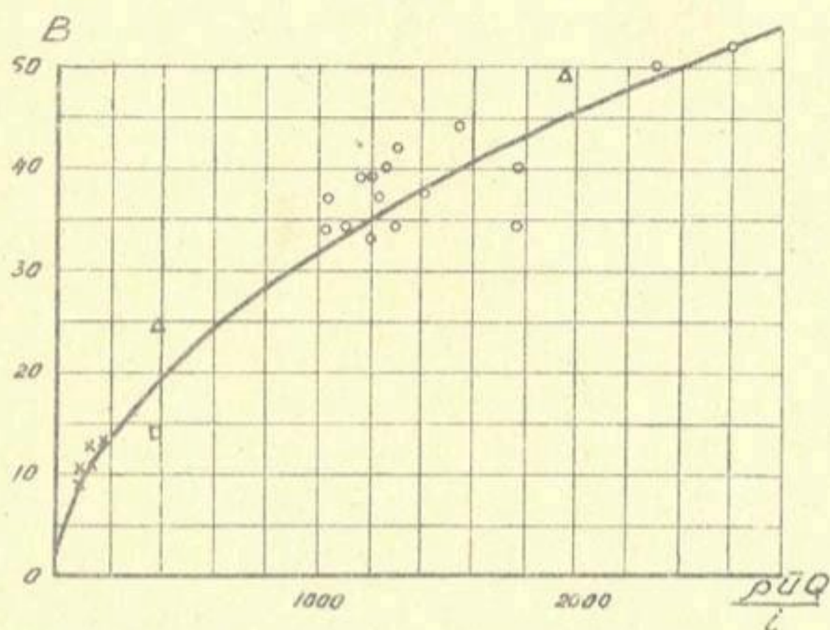
Рис. 4. График зависимости B = f\left(\frac{Q}{\gamma} \cdot \rho l\right)
