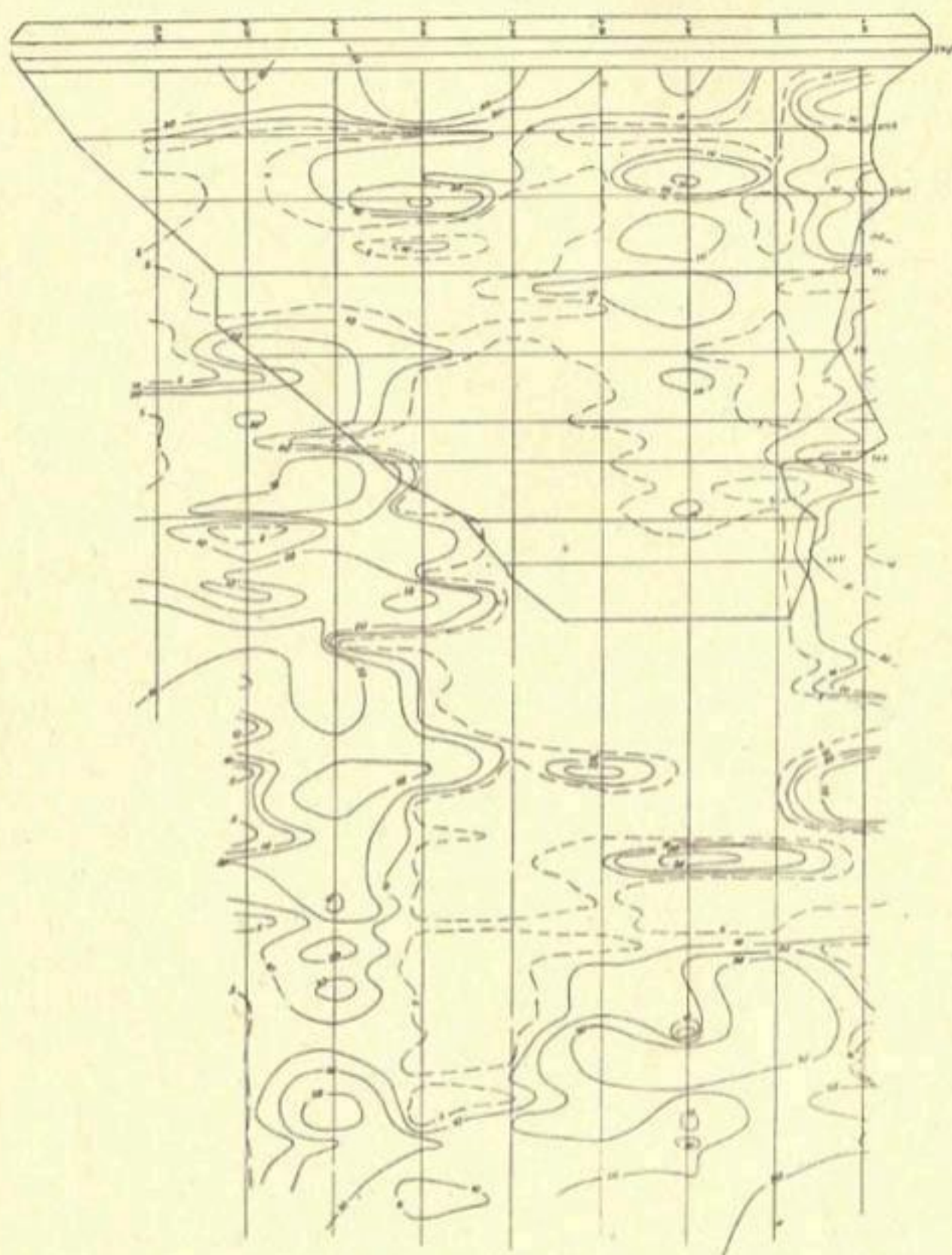
Рис. 7. Карта скоростей придонных течений в мм/сек на Каркиданском водохранилище при ГВВ 120м, май 1968г.
