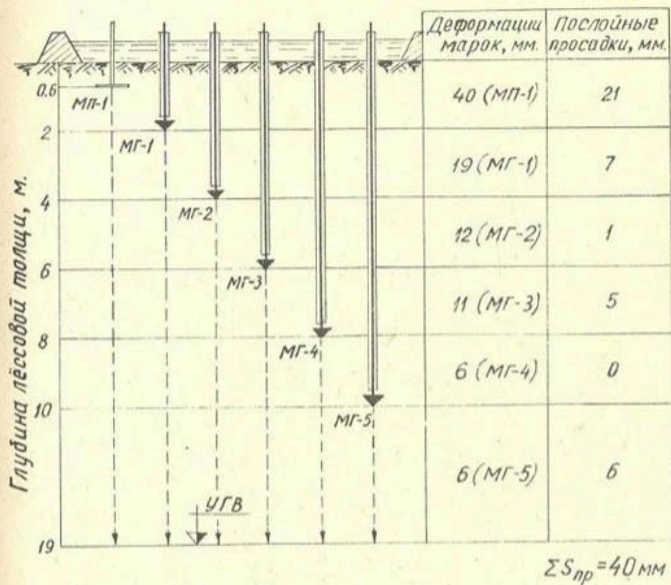
Рис. I. Величина осадок глубинных и поверхностных марок.
