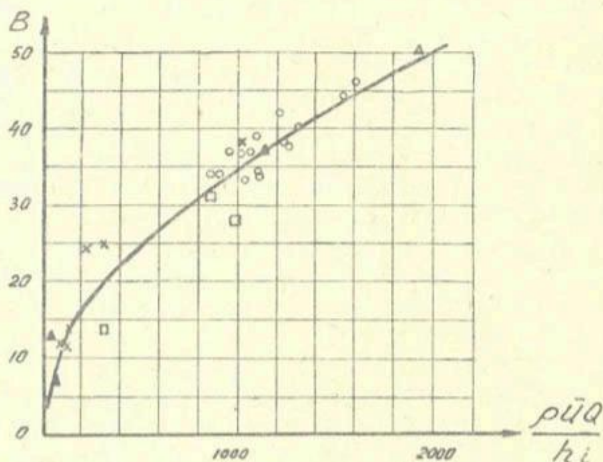
Рис. 5. График зависимости B = f\left(\frac{\rho \bar{u} Q}{h_i}\right) ○ — спрямление к-ла им. Ленина; × — " " Боз-яб и Боз-яб ГКИ 64г; △ — канал им. Ленина ГКИ и 30; ▲ — каналы Кенегес и Кулабад; □ — канал Кегейли.
