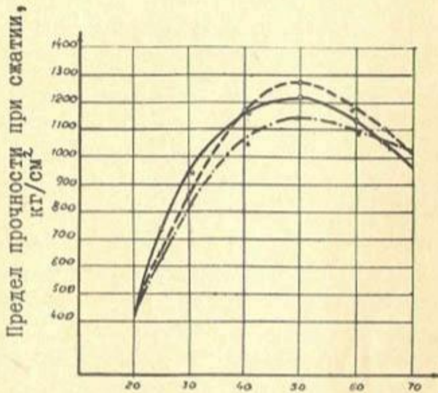
Рис.2.Изменение прочности полимербетона на различных смолах в зависимости от количества отвердителя бензолсульфокислоты: _____ смола ФД-1; - - - смола ФД-2; - · - · - смола ФД-3.
