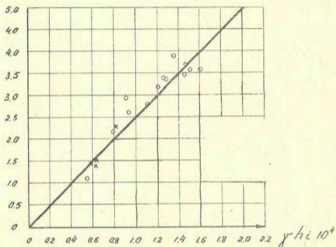
Рис. I. График зависимости нагрузки потока от \gamma h i o — спрямление к-да им. Ленина (1967г.); x — " " " Боз-яб (1967г.)
