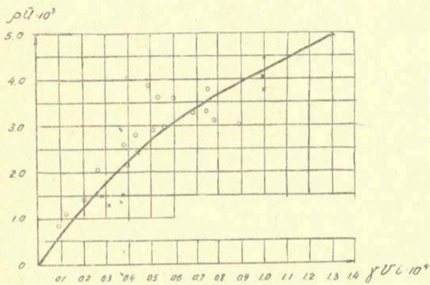
Рис.2. График зависимости нагрузки потока \rho \bar{g} от \gamma V \bar{g} o — спрямление к-да им.Ленина (1967г.); x — " " " " Боз-яб (1967г.).
