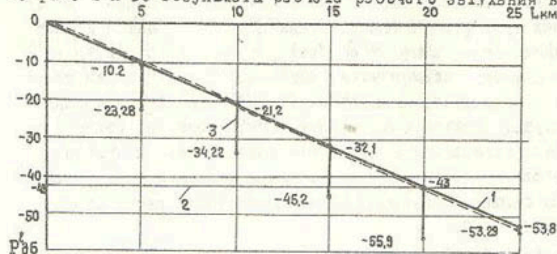
Рис. 2. Зависимость уровня приема сигналов ТУ ( P^L ) от длины цепи с пятью КП, включаемыми в цепь кабельной линии при согласованной нагрузке на конце ( R_n ) 600 Ом: 1 — собственное затухание цепи; 2 — допустимый уровень приема; 3 — затухание, вносимое высоким сопротивлением КП в режиме приема
