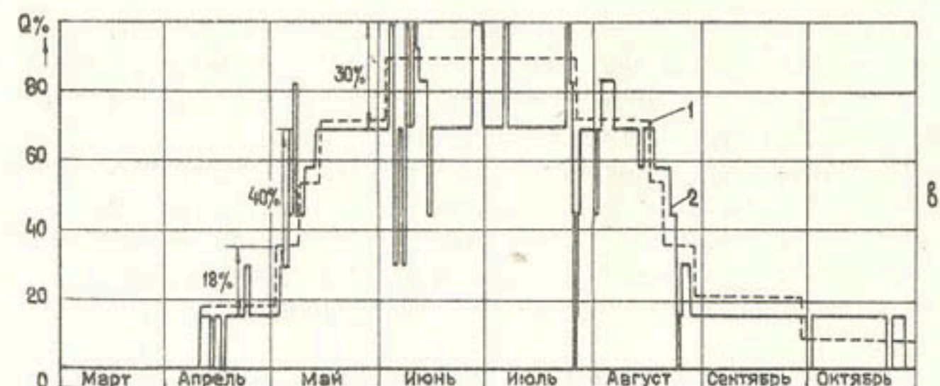
Рис. I. Графики водоподачи (1 — по плану; 2 — фактическая): а — в нижнем бьефе перегораживающего сооружения на ПК 923 Южного Голодноостепского магистрального канала; б — в голове Каршинского магистрального канала; в — в голове Джизакского магистрального канала ДМ-1
