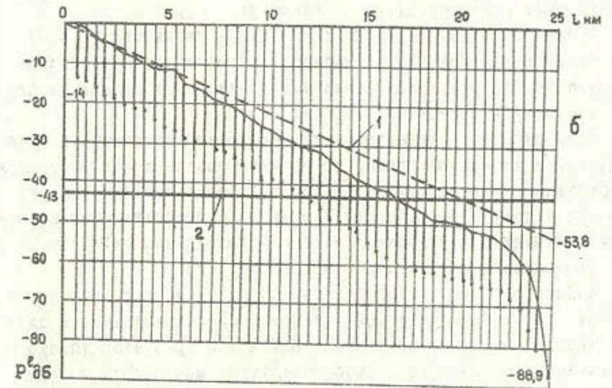
Рис. 3. Зависимость уровня приема сигналов ТУ ( P^L ) от числа КП, включаемых в цепь кабельной линии, при отсутствии согласующего сопротивления R_n (а — при 10 равномерно подключенных КП; б — при 50 равномерно подключенных КП): 1 — собственное затухание цепи; 2 — допустимый уровень приема
