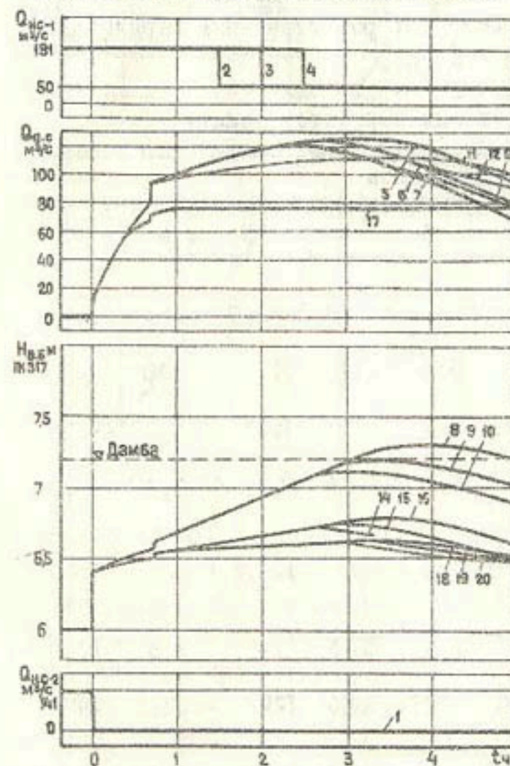
Рис. 5. Переходные режимы в в.б. на пк 317 ДМ-I при 100%-ном отключении НС-2 ( \Delta Q_k = -141 м³/с), работа аварийного автоматического водосброса различной пропускной способности ( Q_{в.с. макс} = 141; 110; 77 м³/с) и оперативном отключении НС-I на \Delta Q_n = -141 м³/с через \Delta t = 1,5; 2; 2,5 ч
