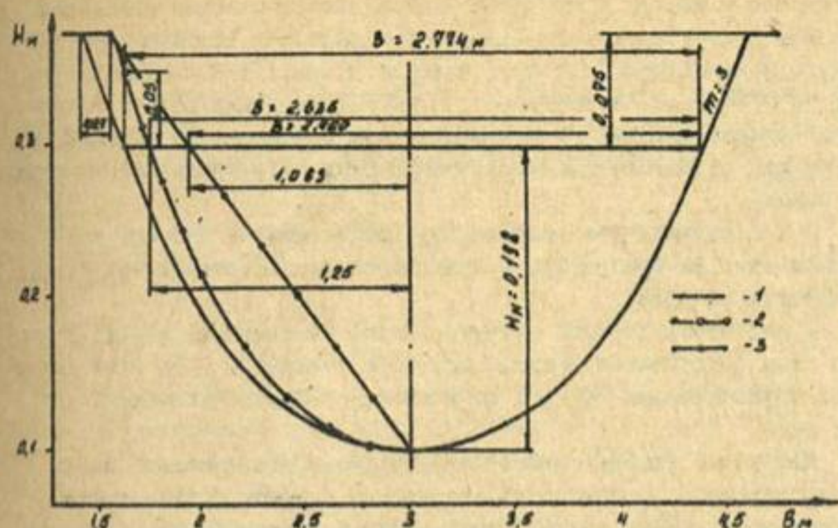
Рис. 1. Поперечное сечение русла в отворе установления выпуклости: 1 – поперечное сечение русла; 2 – I тип выпуклости; 3 – II тип выпуклости.
