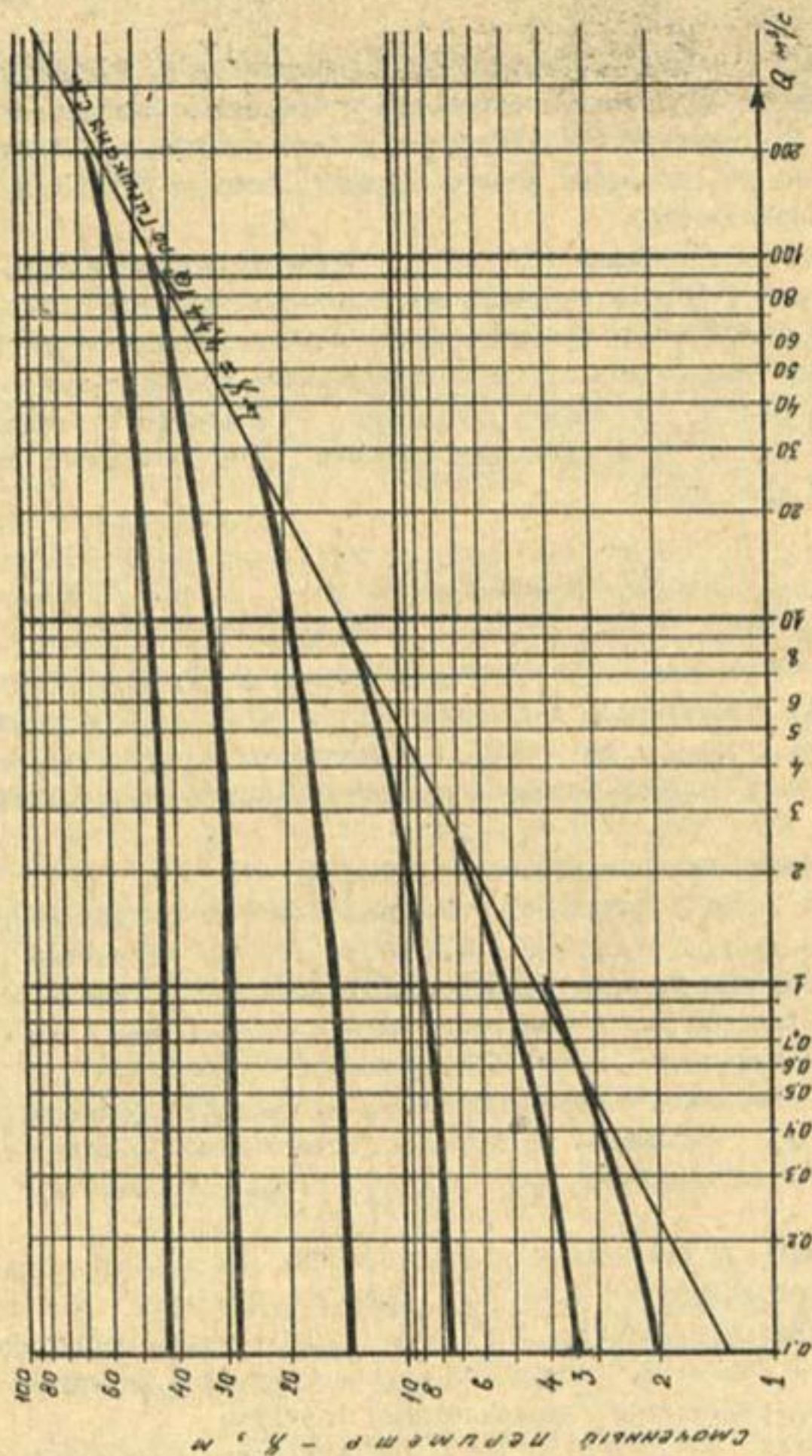
Рис. I. Зависимости смоченного периметра от проходящих по каналу расходов для каналов с максимальными расходами 200; 100; 30; 10; 2,5 и 1 \text{м}^3/\text{с} .
