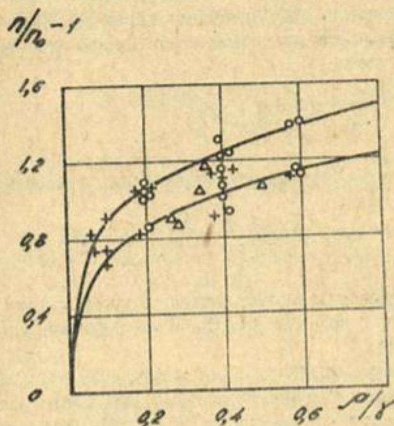
Рис.3. График изменения коэффициента шероховатости от относительного количества наносов в потоке.
