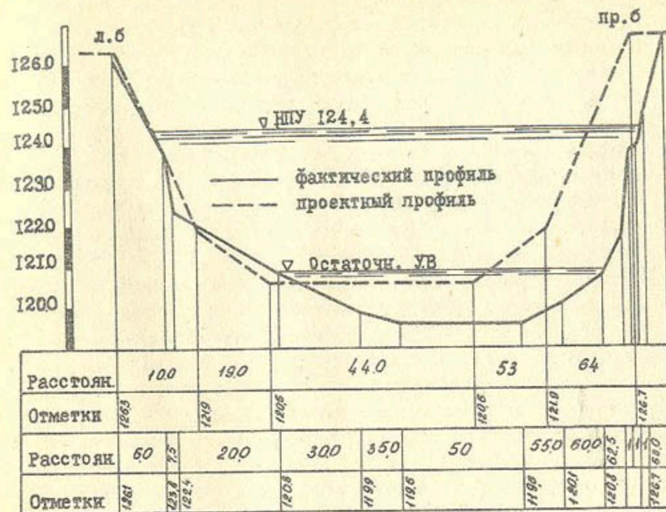
Рис. I. Поперечный профиль русла ЛМК на ПК 391
