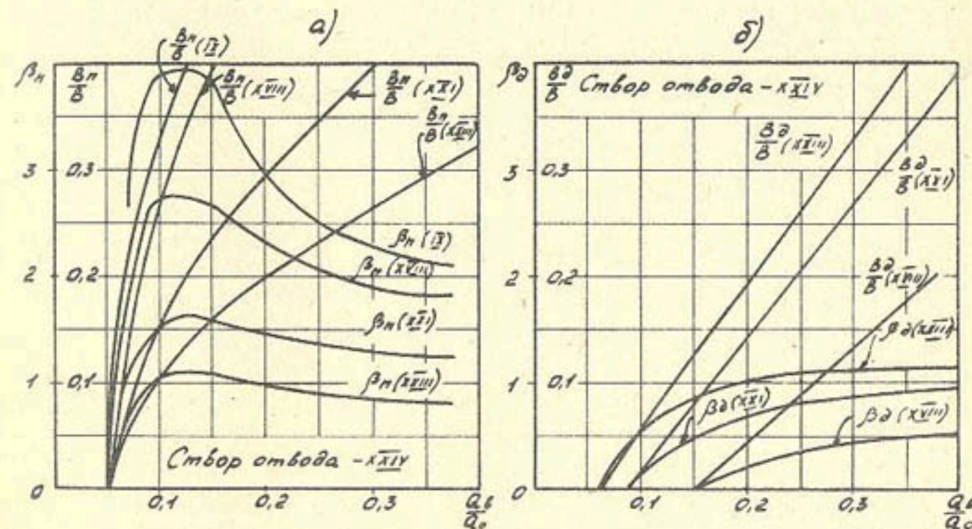
Рис. 6. Графики \frac{B_n}{B} , \beta_n , \frac{B_d}{B} и \beta_d при расположении водоприемника в ХХІУ створе (75°).
