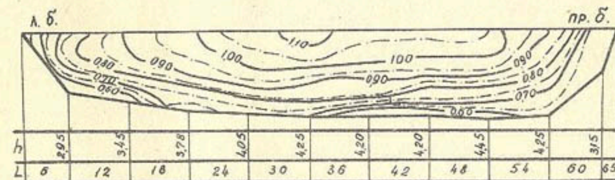
Рис. 3. Поперечный профиль и поле скоростей в основном русле ниже входа в ЛМК-8 ( Q = 171 \text{ м}^3/\text{сек} )
