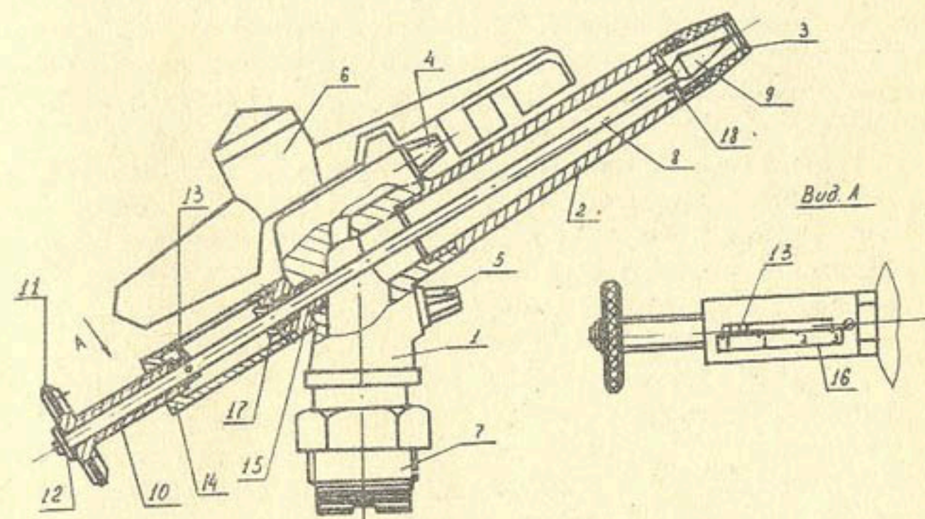
Рис. I. Дождеватель с регулируемым выходным сечением сопла (ДР-I):
