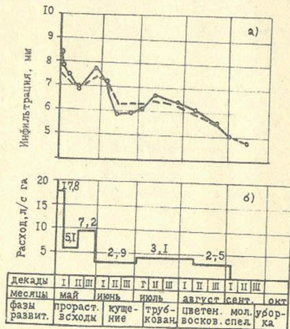
Рис.2. Гидромуль водоподачи (б) и инфильтрация воды из чеков (а), — — — — — расчетные по формуле (20), о о о — опытные по данным эксперимента.
