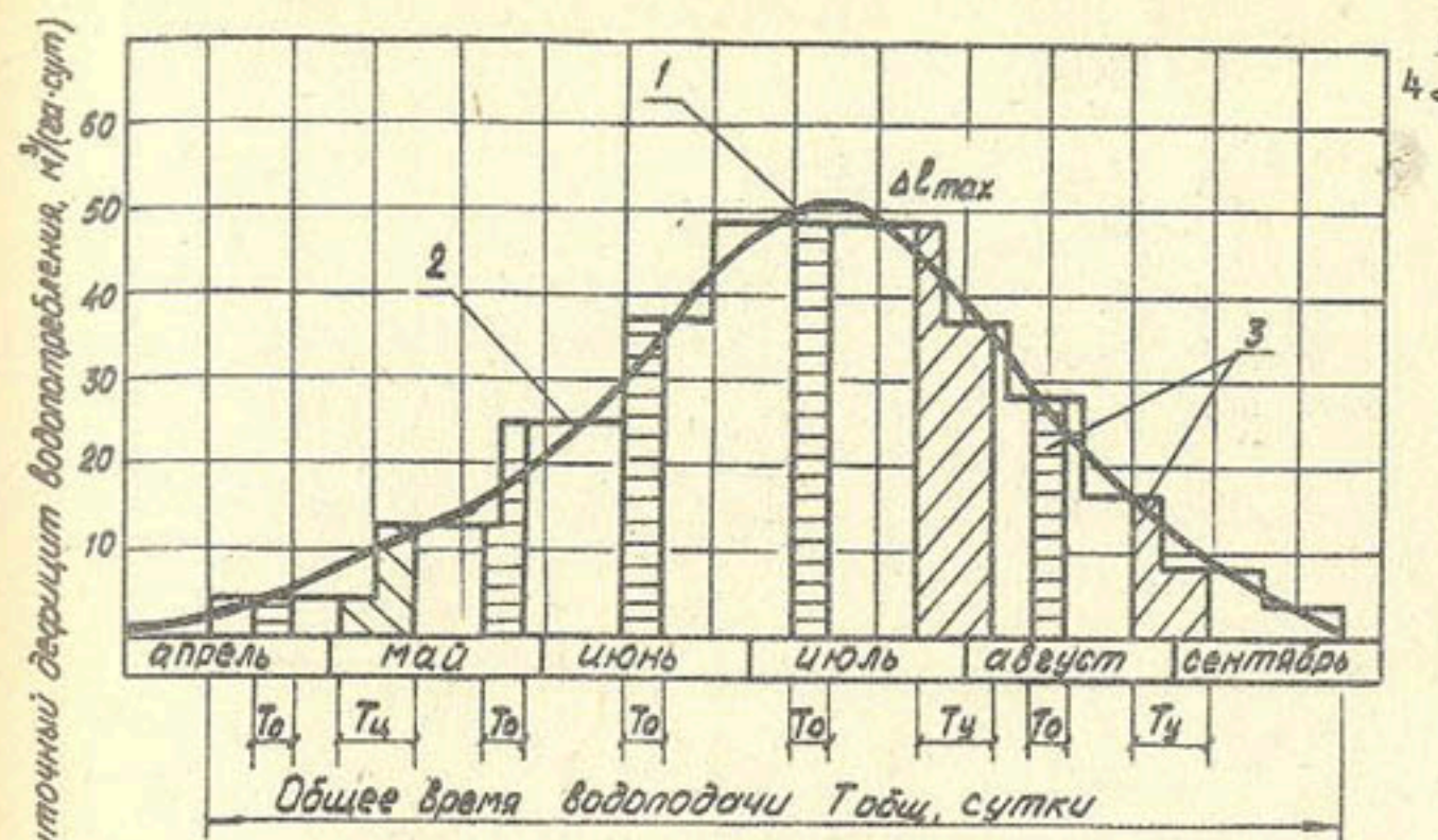
Рис. 1. Зависимость между водопотреблением яблоневого сада и водоподачей при синхронно-импульсном дождевании:
