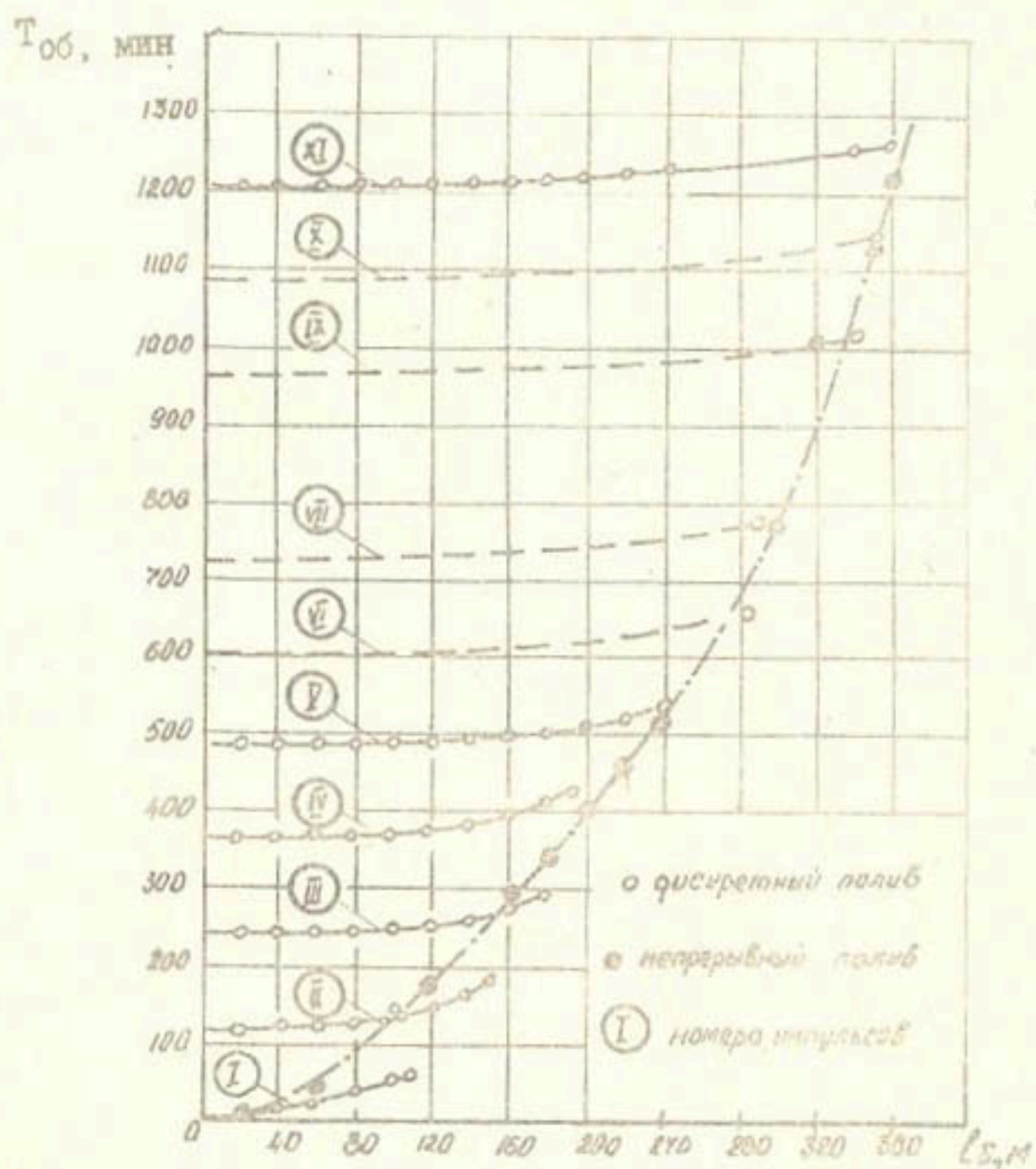
Рис.2. Кривые добегаания при непрерывном и дискретном поливе струей q_0 = 0,74 л/с.
