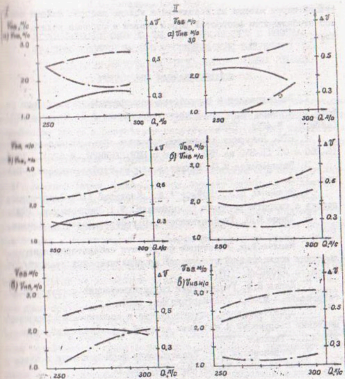
Рис. 8 Графики зависимости абсолютных скоростей в крайних точках со стороны нижнего (т.12) и верхнего (2.2) бьефов от расхода и градиента скорости \Delta V = \frac{V_{max} - V_{min}}{V_{cp}} I- без вставок; II- со вставкой; а) без щитов; б) со щитом справа; в) со щитом слева;
