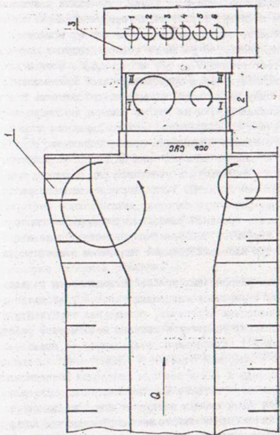
Рис. 2 Схема образования вихревых зон в подводящем тракте НС-1 КМК: 1 - подводящий канал; 2 - обтекатель; 3 - здание НС.
