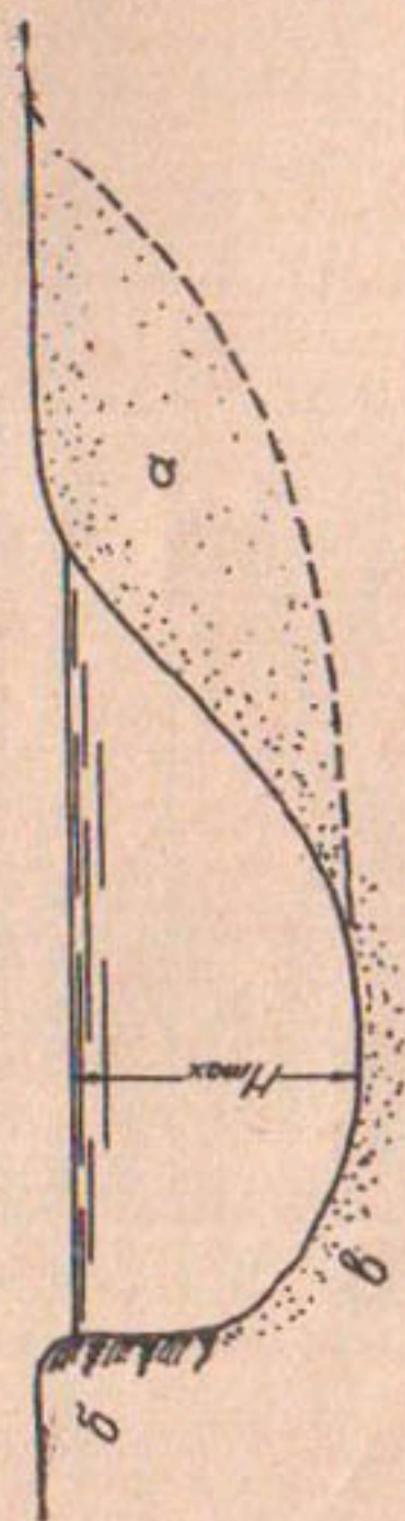
Рис. 5 Схема поперечного сечения русла при девиации III го типа; а - зона отложения; б - глинистый грунт; в - песчаные грунты.
