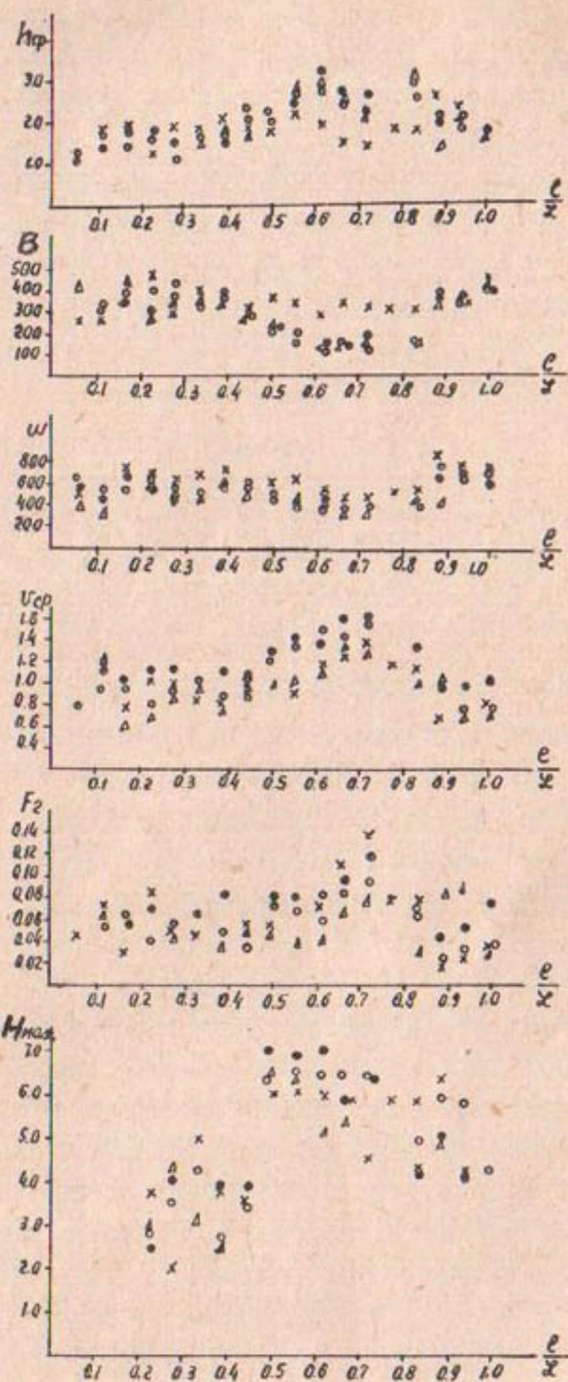
Рис. 3 Графики зависимости h_{cp}, B, \omega, v_{cp}, F_2, H_{max} = f\left(\frac{l}{L}\right)
