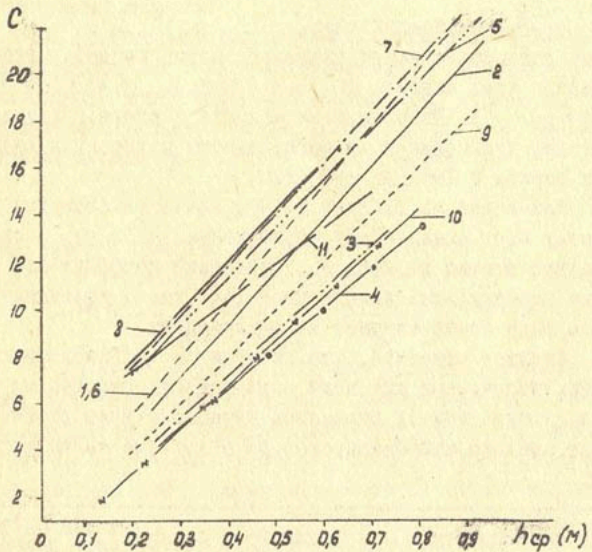
Рис.2. График зависимости C = f(h_{cp}) с 1952
