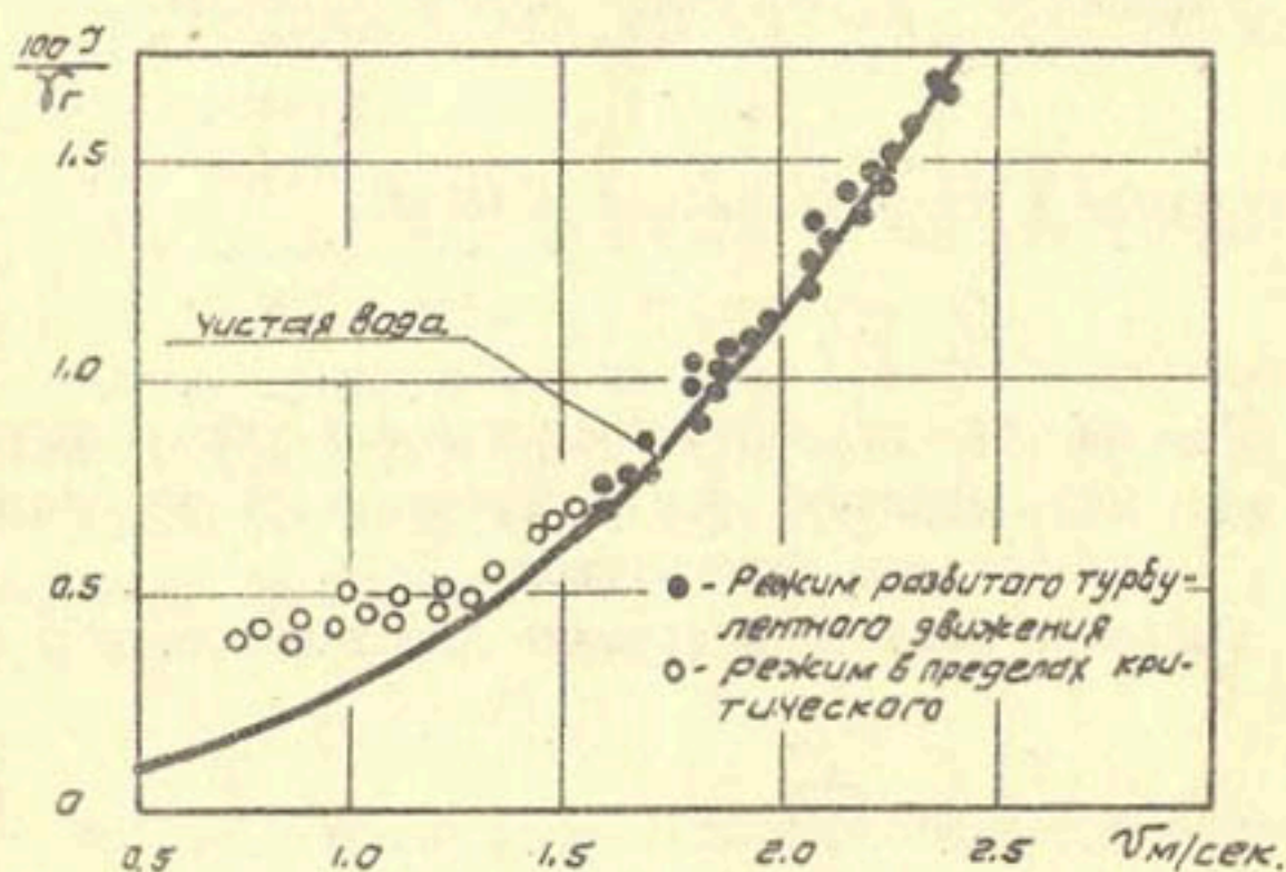
Рис. I. Зависимость гидравлического уклона (приведенного к воде) от скорости движения гидро-смеси; диаметр трубопровода D=200\text{мм} , d_{\text{ср}}=0,047\text{мм} , \gamma_r=2,65 \text{ т/м}^3
