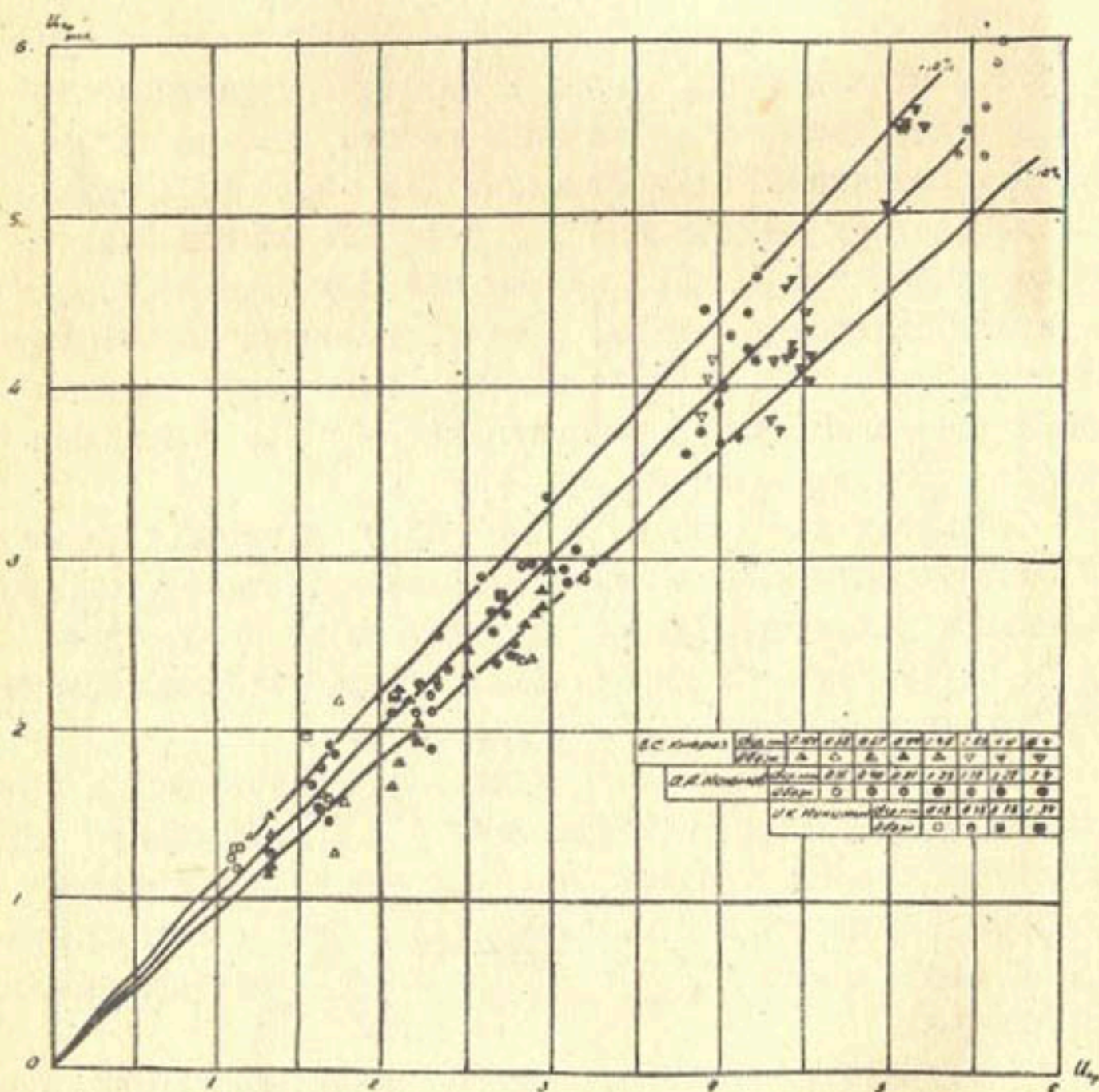
Рис.4. Результаты сопоставления величины U_{ж} по формуле (8) с опытными значениями.
