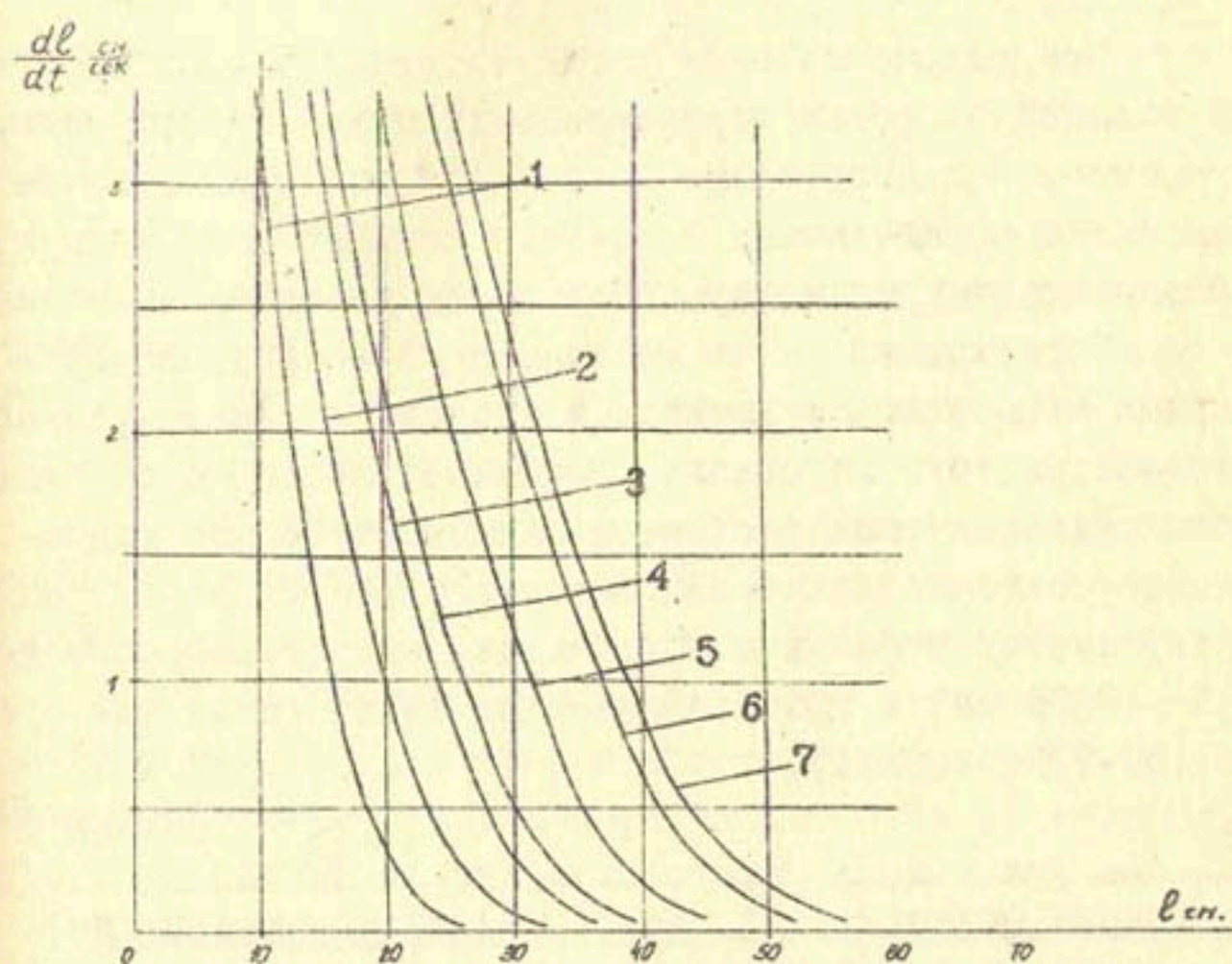
Рис.8. Зависимость длины воронки размыва от скорости перемещения насадки вдоль ее продольной оси (условия те же, что и для рис.7).
