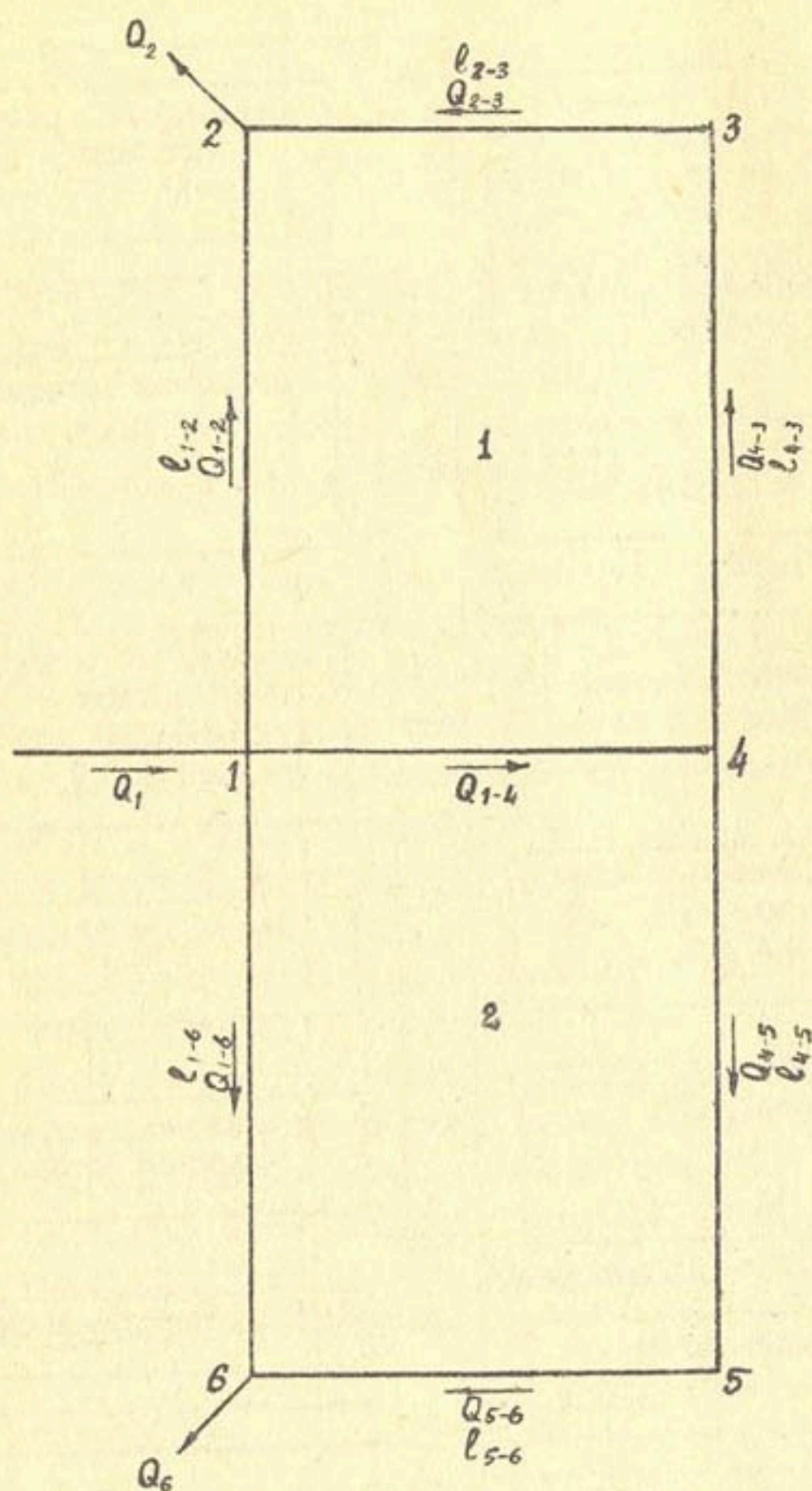
Рис. 2. Расчетная схема сети из параллельно закольцованных трубопроводов.
