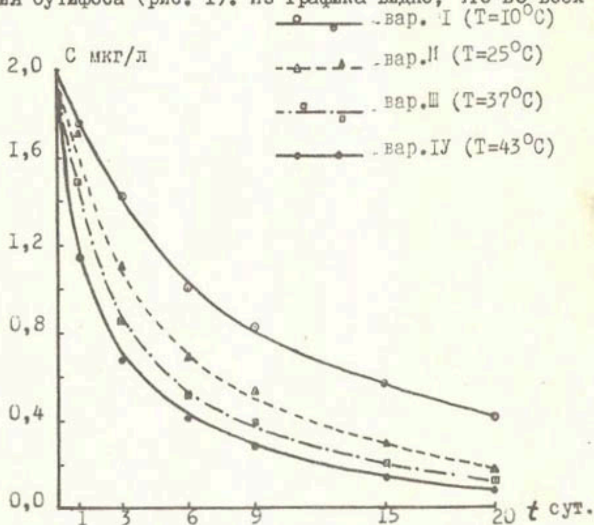
Рис. 1. Кинетические кривые разложения бутифоса в воде ( \rho\text{H} = 6 ).
