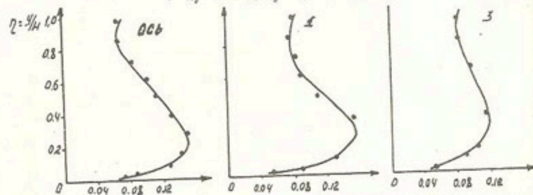
Рис.2. Графики распределения значений интенсивности турбулентности ( \zeta_u/\bar{u}_b ) по глубине потока при U/U_0 = 1,1 в опыте 2 ( H_{cp} = 0,30 м, \beta_{cp} = 20 , H_{m0} = 0,427 м).
