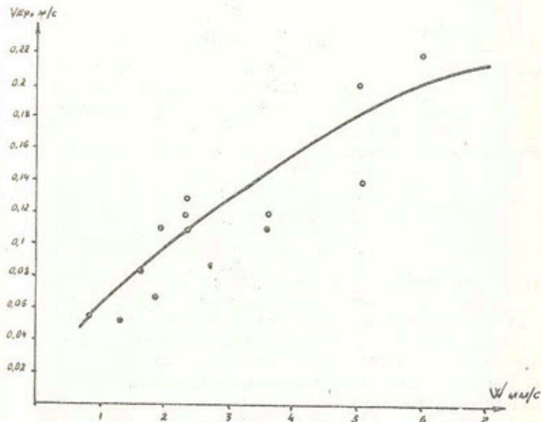
Рис. 2. График зависимости V_{кр} от гидравлической крупности W : о — для керамических дренажей; * — для пластмассовых дренажей.
