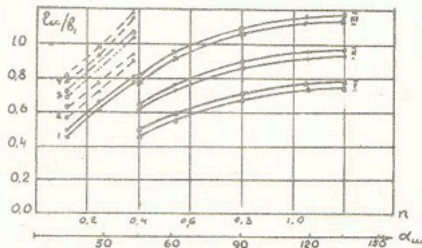
Рис. 2. Графики зависимостей l_{cc}/b_1 = f(n) l_{cc}/b_1 = f(\alpha_w) .
