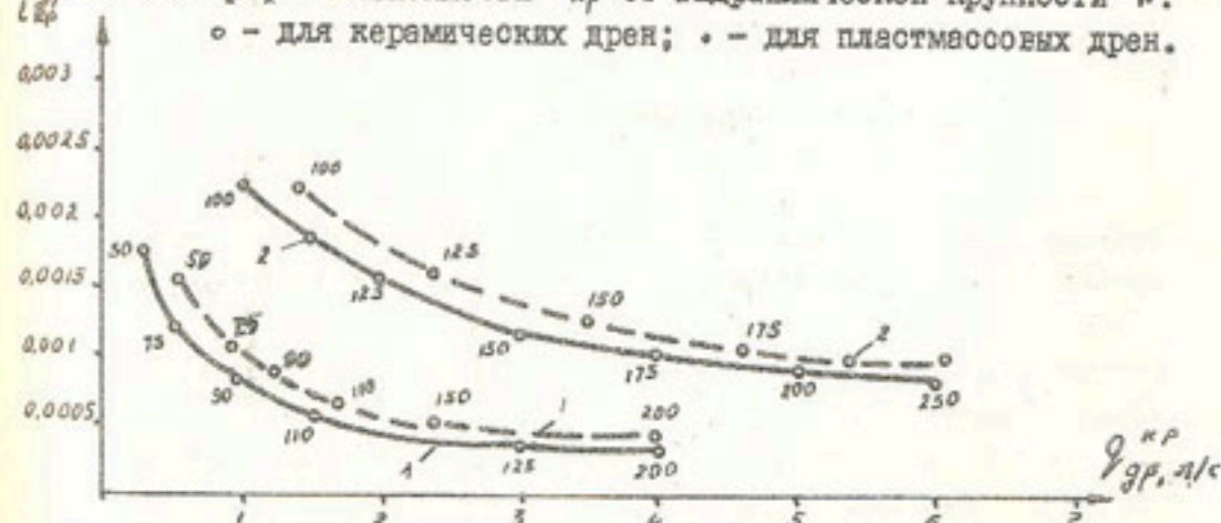
Рис. 3. График зависимости i_{кр} от q_{др} при W = 3,0 мм/с (1 — пластмассовый дренаж с искусственным или комбинированным фильтром) и 8,0 мм/с (2 — керамический дренаж) (числа у линий — диаметры труб).
