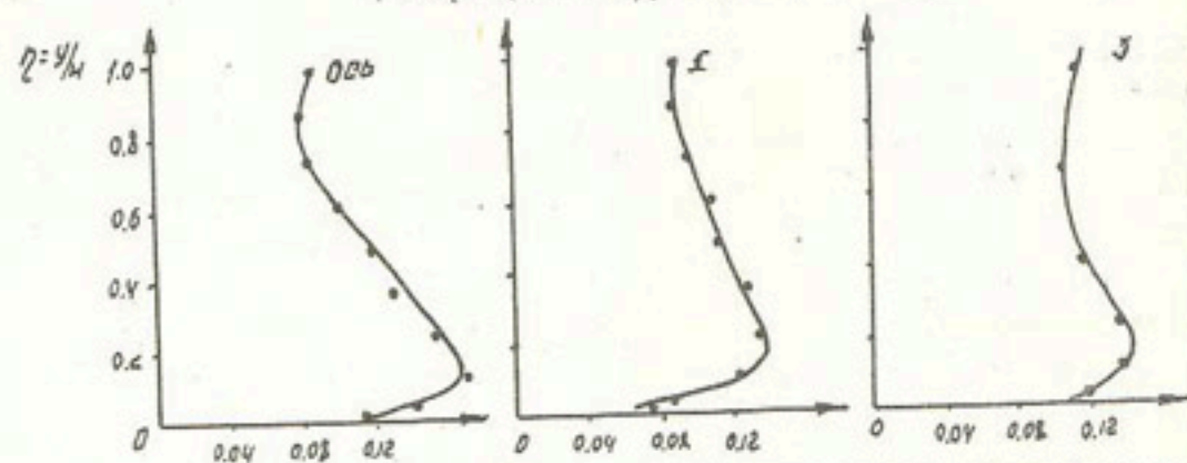
Рис.3. Графики распределения значений интенсивности турбулентности (продольной составляющей \zeta_u/\bar{u}_b ) по глубине потока при U/U_{crit} и грядовой форме дна в конце опыта 2.
