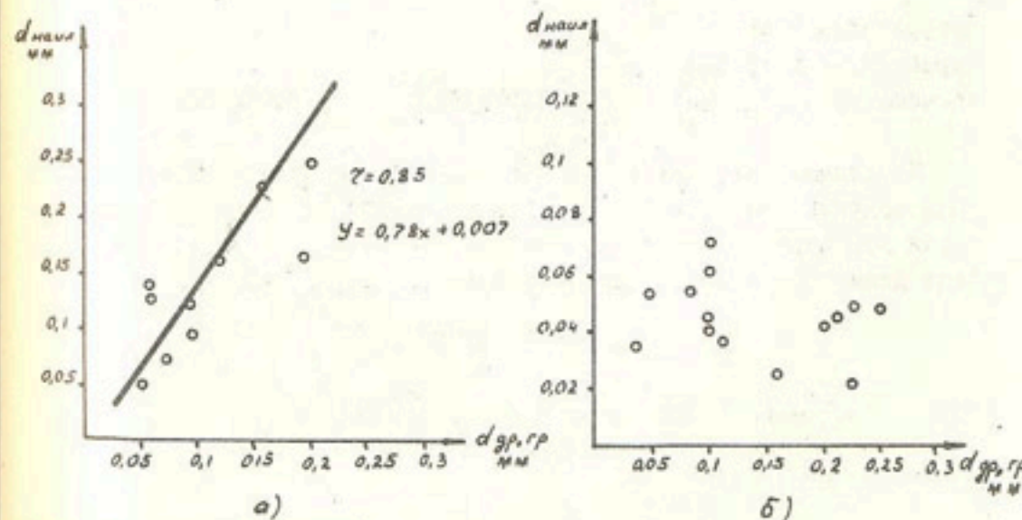
Рис.1. График зависимости средневзвешенного диаметра частиц наилок от средневзвешенного диаметра частиц дренажного грунта: а – для керамических дрен; б – для пластмассовых дрен с искусственным и комбинированным фильтром.
