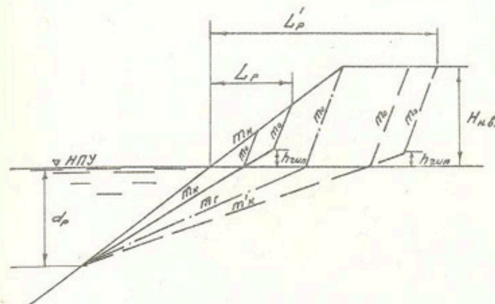
Рис.1. Расчетная схема размыва откоса из несвязного грунта ветровыми волнами при постоянном уровне воды.
