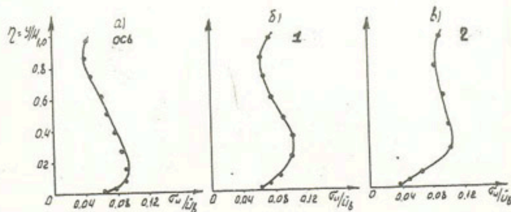
Рис.1. Графики распределения значений интенсивности турбулентности ( \zeta_u/\bar{u}_b ) по глубине потока при U/U_0 = 1,1 в опыте I ( H_{cp} = 0,30 м, \beta_{cp} = 20 , H_{m0} = 0,413 м).
