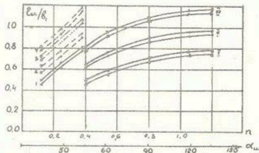
Рис. 2. Графики зависимостей l_{cc}/b_1 = f(n) l_{cc}/b_1 = f(\alpha) .
