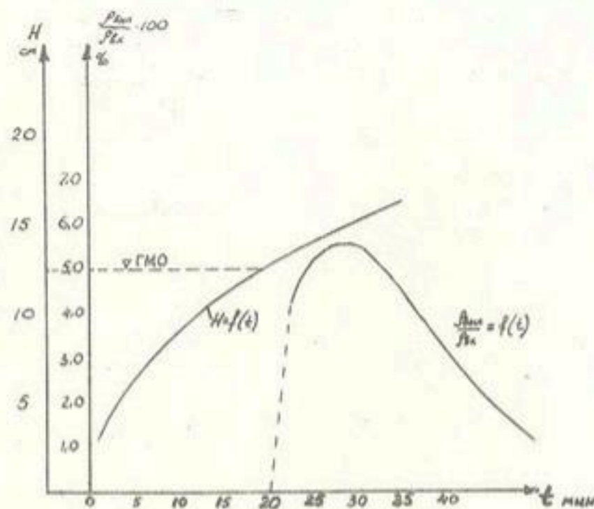
Рис.3. Графики h=f(t) и \frac{P_{\text{вых}}}{P_{\text{вх}}} \cdot 100 .
