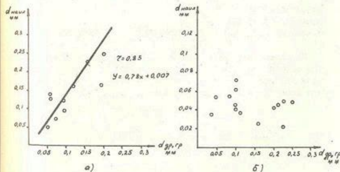
Рис.1. График зависимости средневзвешенного диаметра частиц наилка от средневзвешенного диаметра частиц дренажного грунта: а — для керамических дрен; б — для пластмассовых дрен с искусственным и комбинированным фильтром.
