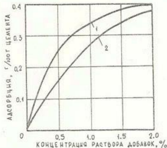
Рис. 3. Зависимость адсорбции от вида и количества добавки: 1 - С-1 Уз; 2 - ПШ.
