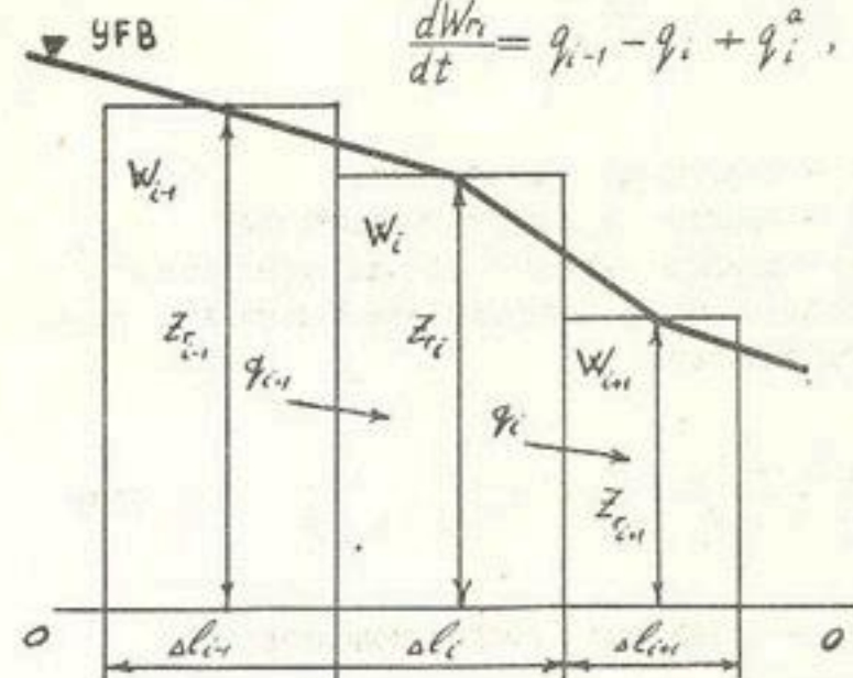
Рис.1. Схема грунтовых вод, представленная в виде последовательности элементов.
