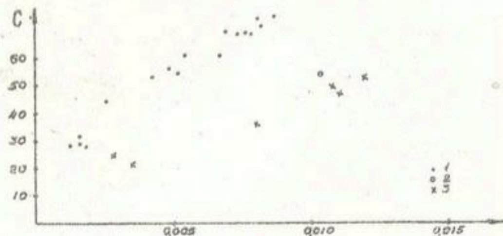
Рис. 2. График зависимости C=f(Fr) для отвора ПК 42: 1 – режим заливания; 2 – критический режим; 3 – режим размыва.
