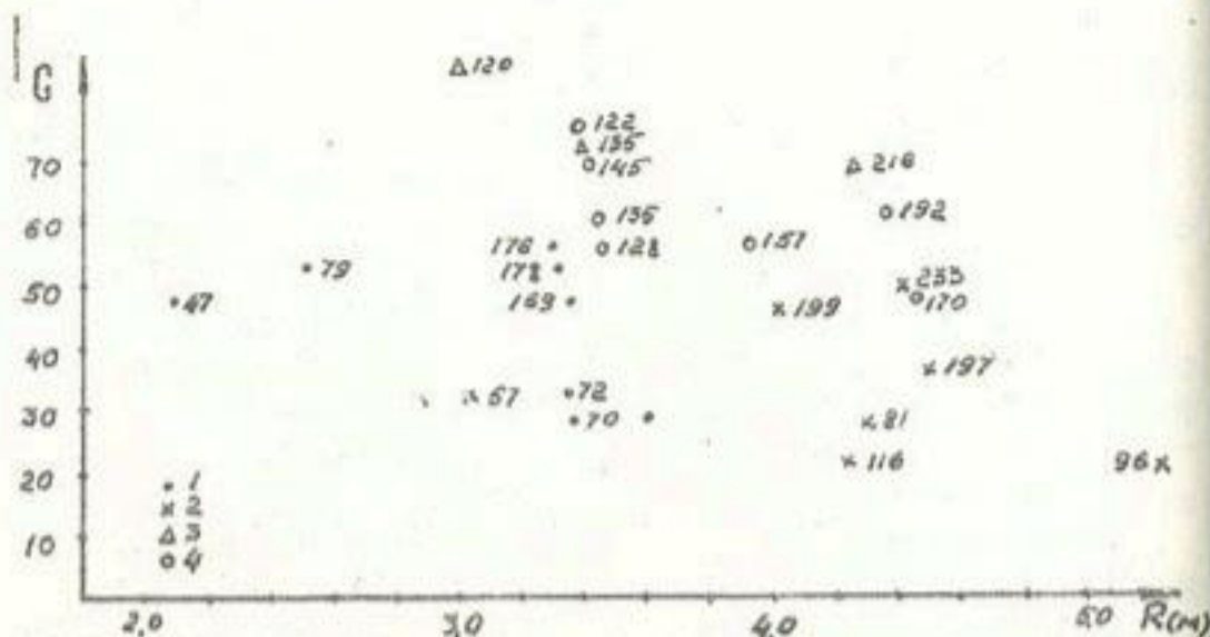
Рис. 1. График зависимости C=f(R) для отвора ПК 42: Измеренные данные: 1 – за 1976 г.; 2 – 1977 г.; 3 – 1983 г.; 4 – 1984 г. (цифры указывают измеренный расход).
