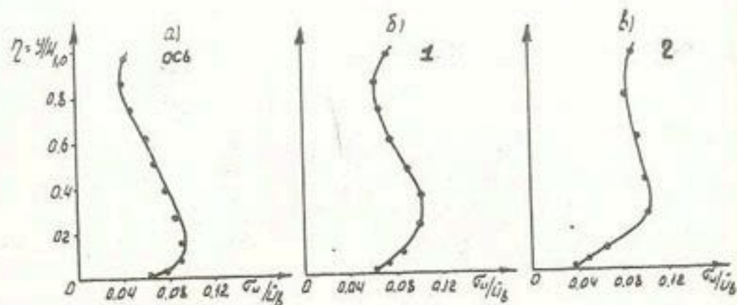
Рис.1. Графики распределения значений интенсивности турбулентности ( \zeta_u/u_b ) по глубине потока при U/U_0 = 1 в опыте I ( H_{cp} = 0,30 м, \beta_{cp} = 20 , H_{mo} = 0,427 м).
