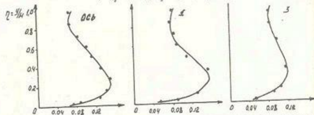
Рис.2. Графики распределения значений интенсивности турбулентности ( \zeta_u/u_b ) по глубине потока при U/U_0 = 1,1 в опыте 2 ( H_{cp} = 0,30 м, \beta_{cp} = 20 , H_{mo} = 0,427 м).
