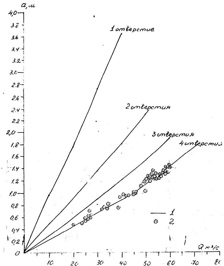
Рис. 5. График a = f(Q, n) ЛМК Казалинского гидроузла
