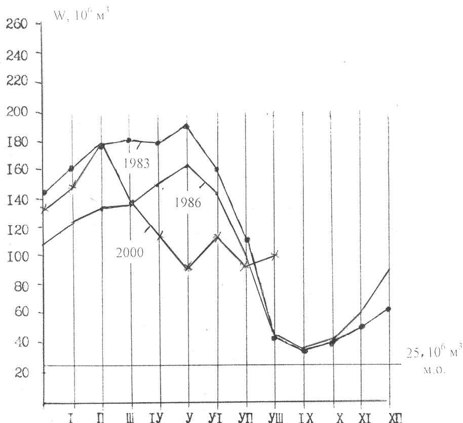
Рис. 1. График наполнения и сработки Ташкентского водохранилища для маловодных лет
