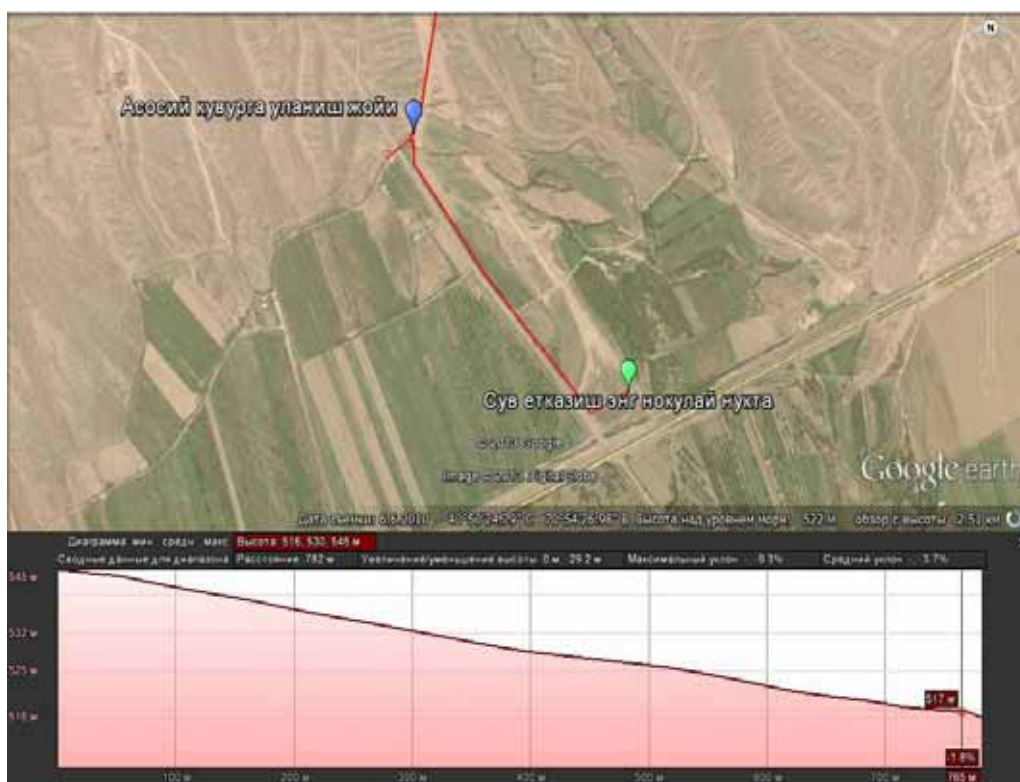
2 расм – Асосий кувурга уланиш жойи ва даланинг сув етказиб бериш энг ноқулай бўлган нуқтаси оралигида ер юзаси абсолют сатҳининг ўзгариши
