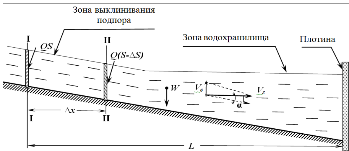
Рис. 1 - Схема расчета видоизменения мутности потока по длине водохранилища
