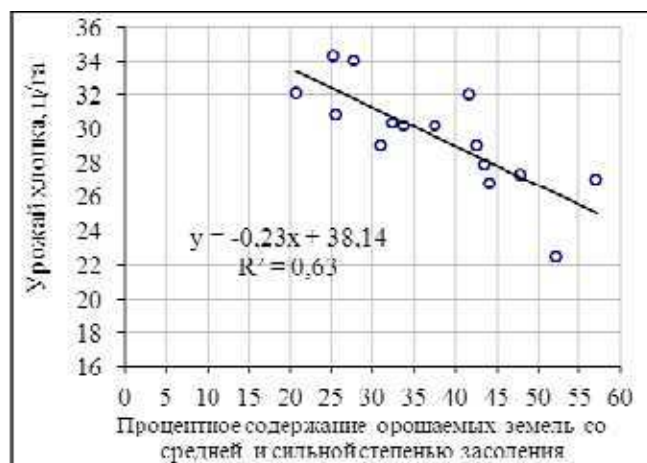
Рис. 8 - Степень влияния распространения засоления на орошаемых землях на урожайность хлопка (обобщённые данные Хазараспскому и Ханкинскому, районам)
