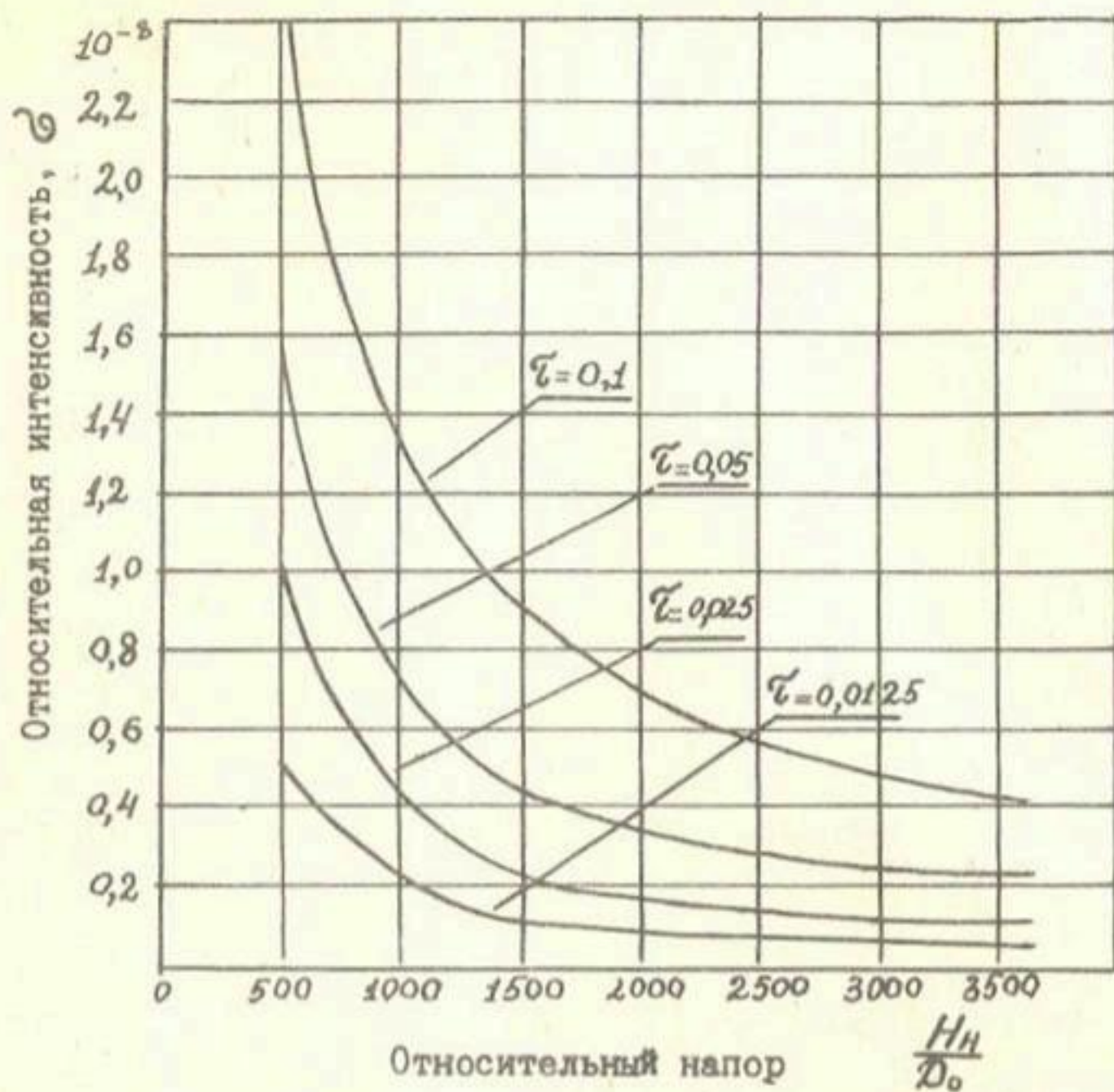
Рис. Зависимость относительной интенсивности от относительного напора
