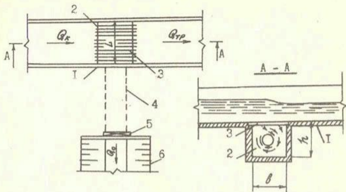
Рис. I Вододелитель-стабилизатор расхода: I - подводящий канал; 2 - водоприемная галерея (приемок); 3 - защитная решетка; 4 - труба; 5 - плоский затвор; 6 - отводящий канал
