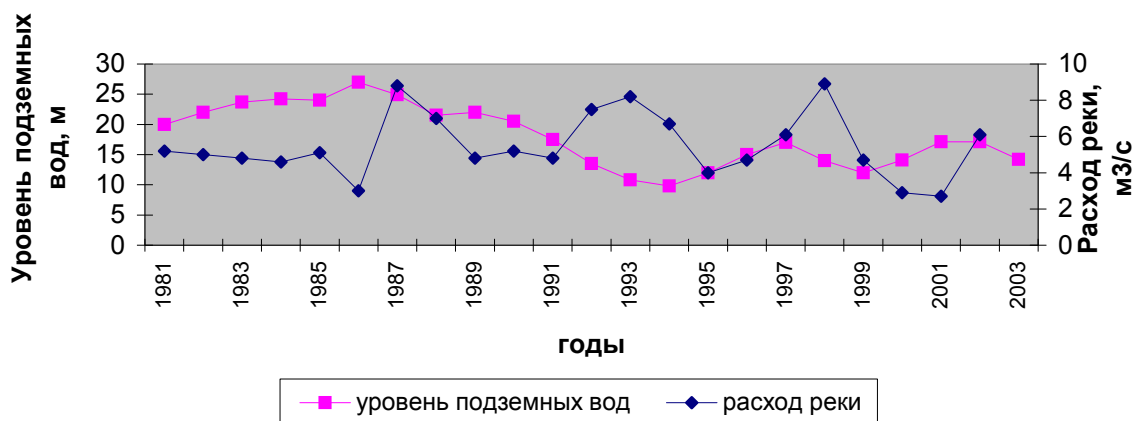
Рис. 1-Среднегодовые уровни подземных вод на линии ВУ-1 и расходы реки Яккабагдаря
