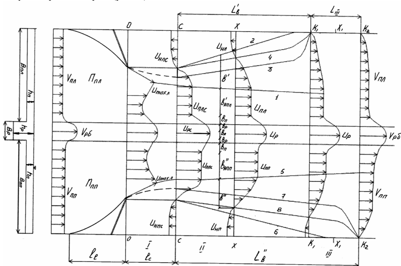
Рис. 1 - Схема растекания потока за поперечными пойменными дамбами ( n_{пл} \neq n_{рб} ), несимметричное растекания)
