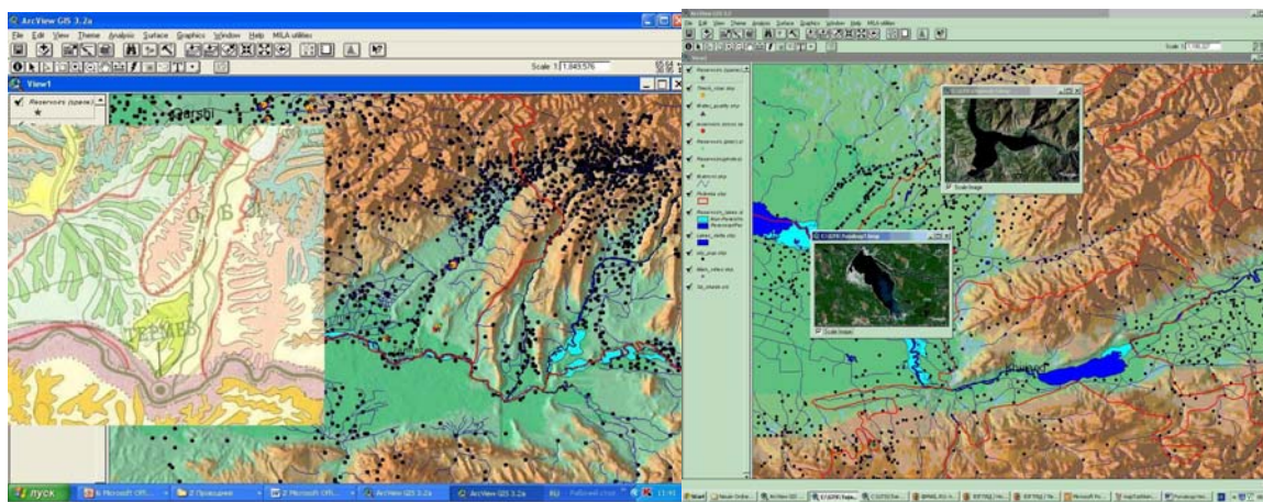
Рис. 2 - Выделение речных бассейнов Узбекистана и их частей методом «пластики рельефа» и ГИС-технологий.
