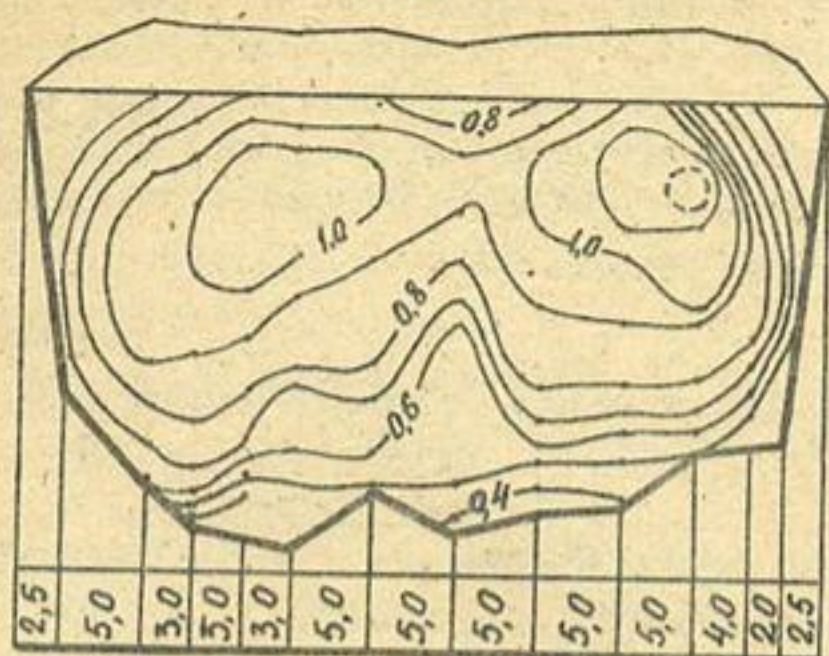
Рис. 1. Изотакхи в поперечном сечении оросительного канала: расход 91 \text{ м}^3/\text{с} , средняя скорость 0,8 \text{ м/с} . Вверху — эшора средних по глубине скоростей.
