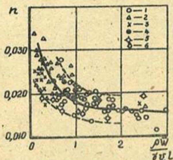
Рис.4. Зависимость n = f\left(\frac{\rho \bar{w}}{\gamma v_*^2 L}\right) 1,2,3,4,5,6 - то же, что и на рис.3.
