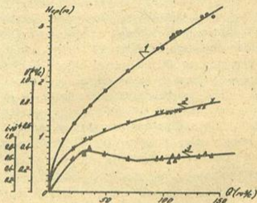
Рис. I Изменения средней скорости, средней глубины потока и уклона водной поверхности в Кызылкумском канале в створе ПК 70 в зависимости от расхода воды по измерениям (САНИИРИ, 1978 г):
