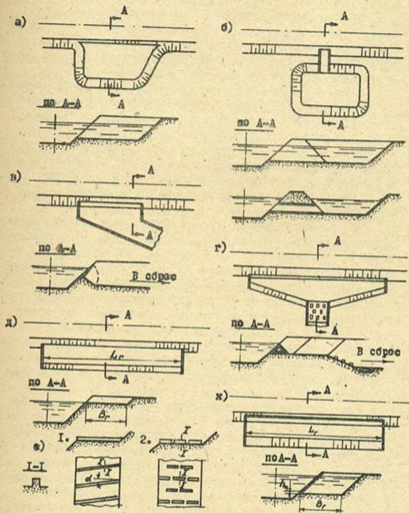
Рис. 2. Гасители положительных волн перемещения: а - боковые уширения; б - емкости, соединяемые с каналом: 1) протокой или 2) трубой; в - боковой водосбор с клапанным затвором; г - боковой водослив; д - гаситель бокового типа; е - то же, с дополнительными гасящими элементами: 1) стенками, 2) шашками; ж - гаситель щелевого типа.
