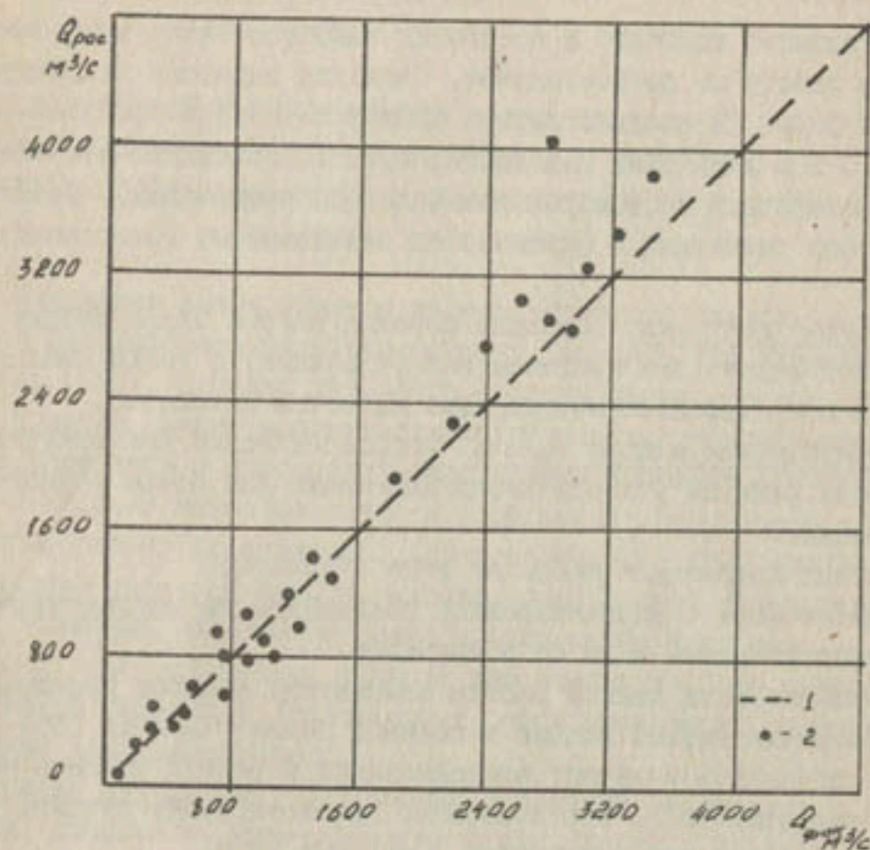
Рис. I. График соответствия расчетных и фактических расходов по створу Дарганата: 1-ось симметрии; 2-измеренные данные.
