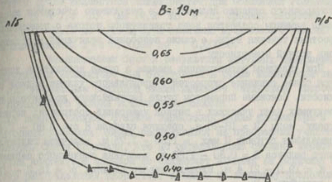
Рис.1. Изоганы скоростей в ств.1 Берунийского коллектора ( M_r = 1:150 , M_B = 1:25 ).
