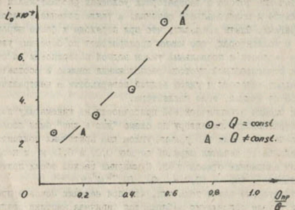
Рис. 4. График зависимости i_0 = f\left(\frac{Q_{np}}{Q}\right) .
