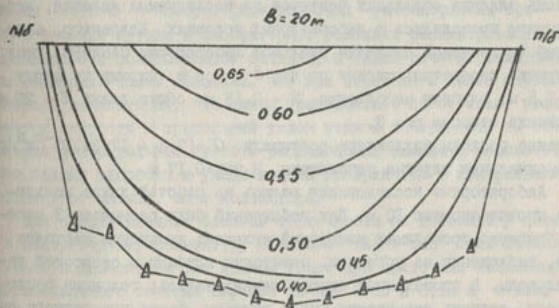
Рис.2. Изоганы скоростей в ств. Берунийского коллектора ( M_r = 1:150 , M_B = 1:25 ).
