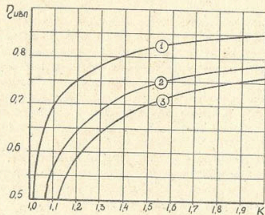
Рис. 2. Зависимость q_{изп} = f(K, \alpha) при водопроницаемости почвогрунтов: 1 - сильной, 2 - повышенной, 3 - средней.
