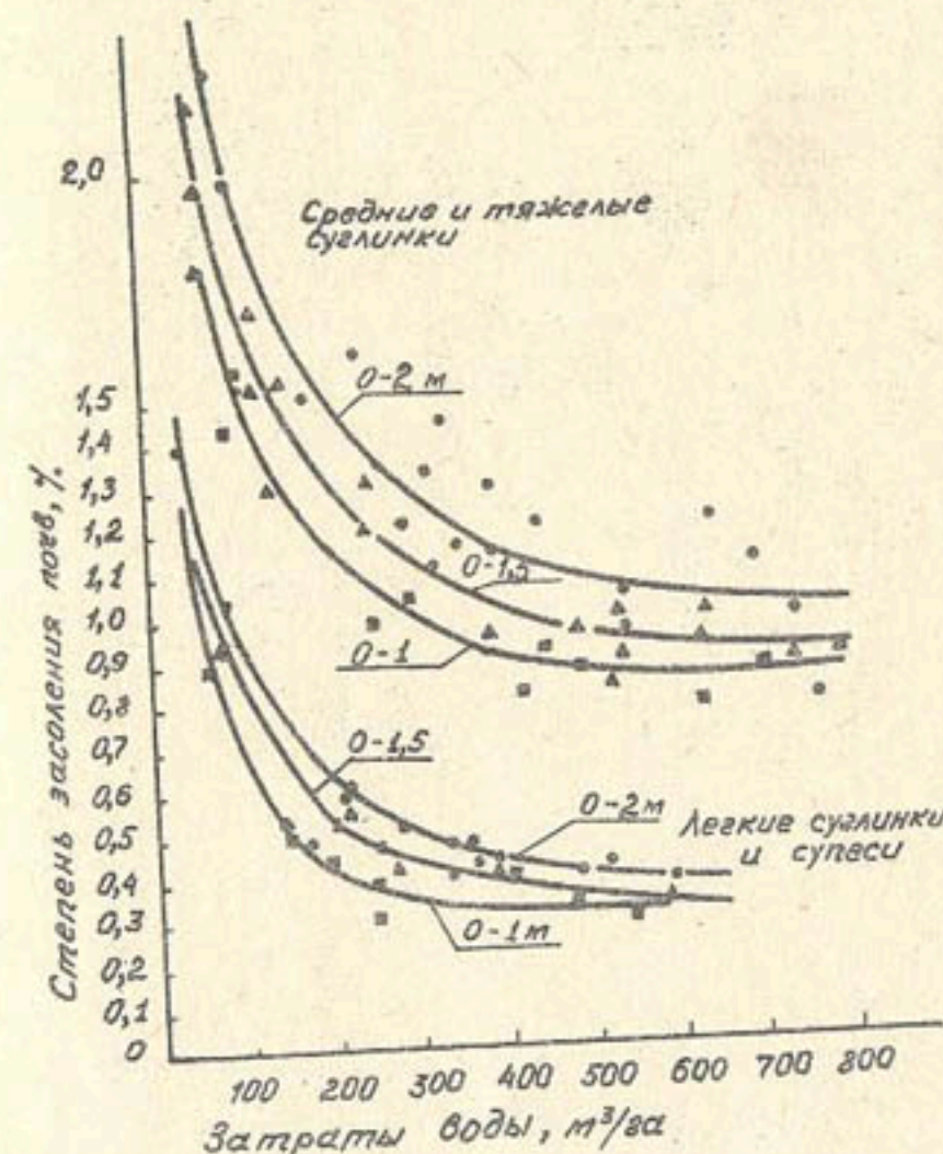
Рис. I. Затраты оросительной воды для выноса I т солей при различном их исходном содержании.
