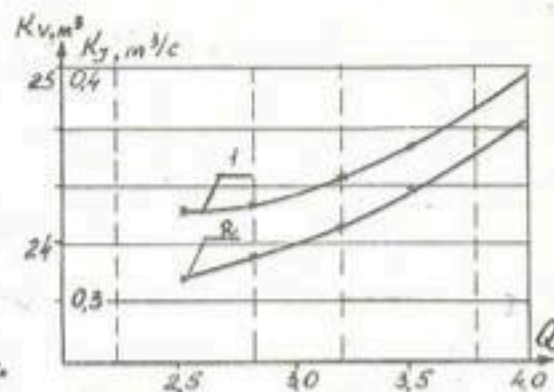
Рис.2. Зависимости коэффициентов K_v (1) и K_y (2) от водоподдачи для расходомера УЗР-В на НА №3 НС №1 ГИМК.
