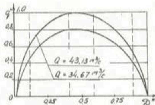
Рис.4. Эпюры удельных расходов, снятые на НА №4 ГНС ( D_{тр.} = 3600 мм).
