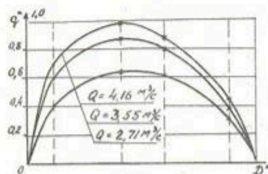
Рис.1. Эпюры удельных расходов, снятые на НА №3 НС №1 ГИМК при 100с осреднения.
