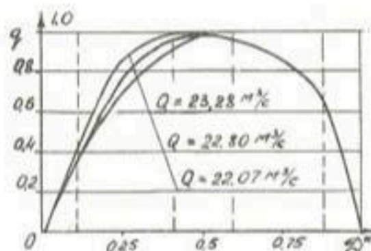
Рис.3. Эпюры удельных расходов, снятые на НА №1 ГНС ( D_{тр.} = 2400 мм).
