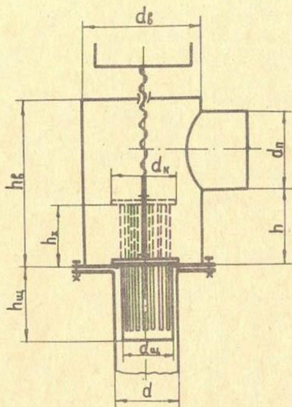
Рис.2. Вентиль с иглой
