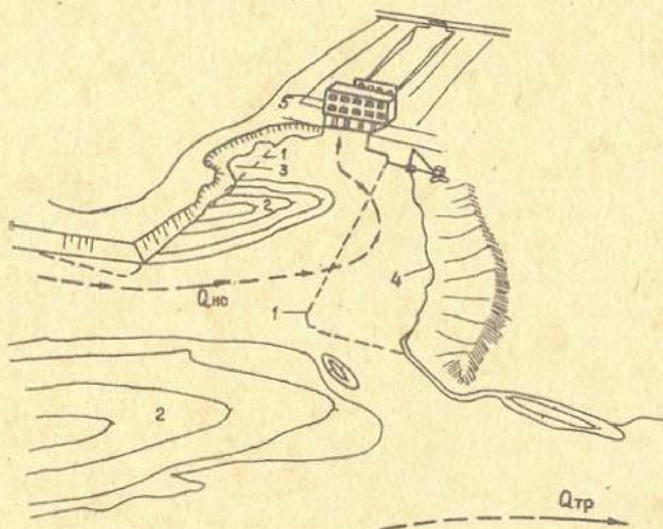
Рис. 2. Схема изменения прямолинейного русла отводящего канала к сырдарьинской насосной станции № 3: 1 - первоначальные границы русла отводящего канала; 2 - участки неравномерного отложения наносов; 3 - зона размыва дамбы канала; 4 - криволинейное русло отводящего канала, сформировавшееся при эксплуатации НС; 5 - насосная станция
