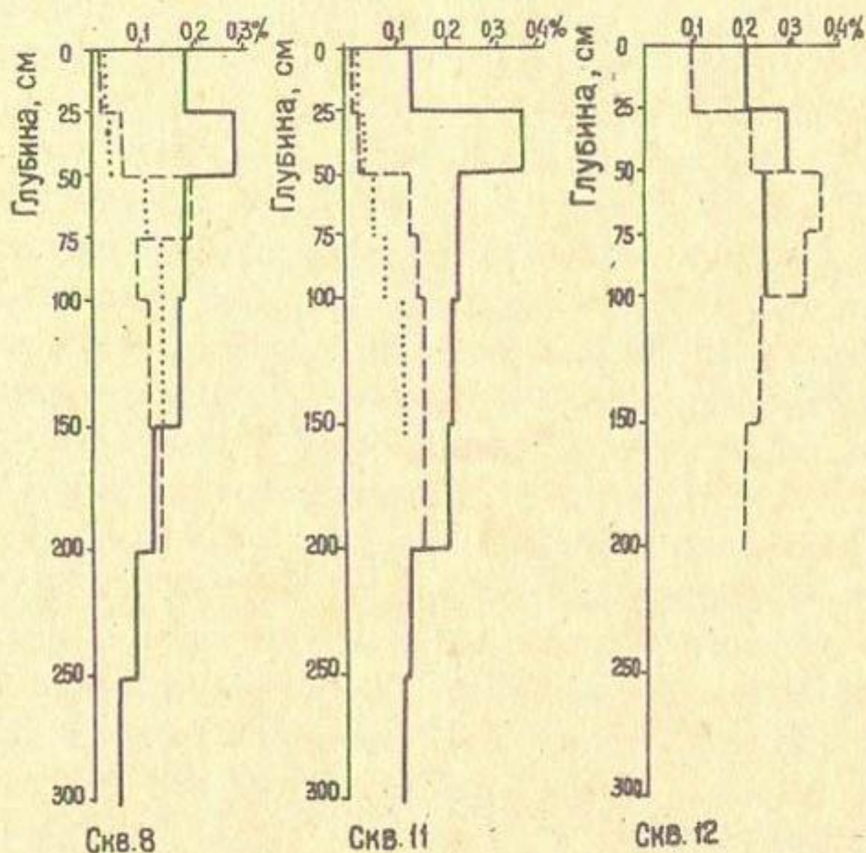
Рис. 1. Распределение хлора по профилю почвы: — исходное содержание; — — — содержание после подачи 5000 \text{ м}^3/\text{га} ; .... содержание после подачи 10000 \text{ м}^3/\text{га}
