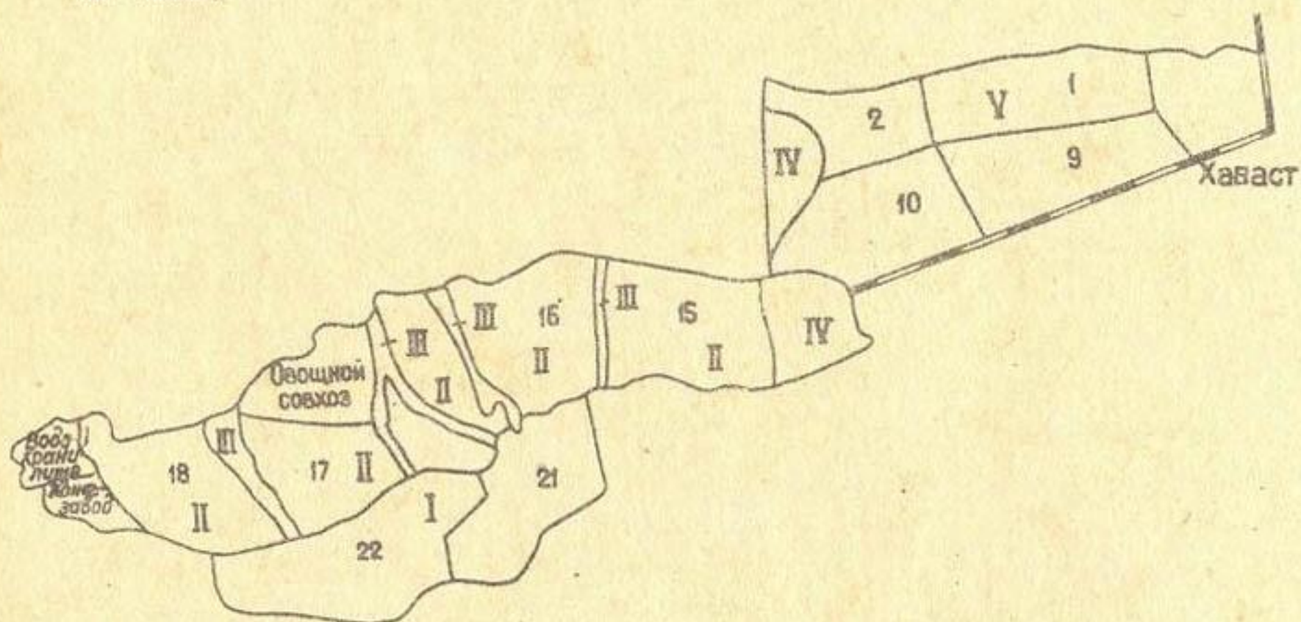
Схема литолого-геоморфологического районирования: [1/2] номер и границы совхоза; [I/II] номер и границы литолого-геоморфологического района
