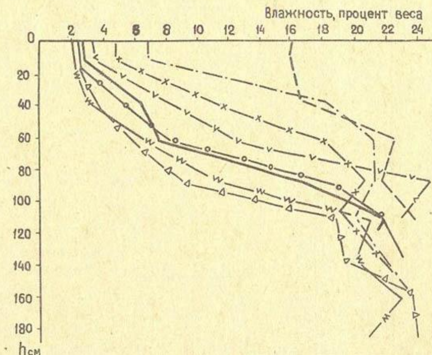
Рис. I. Динамика влажности почвогрунтов в точке 7 после второго полива по бороздам: — в первый день; --- на третий день; —х— на шестой день; —V— на десятый день; —O— на пятнадцатый день; —W— на двадцать первый день; —Δ— на двадцать четвертый день; — исходная влажность
