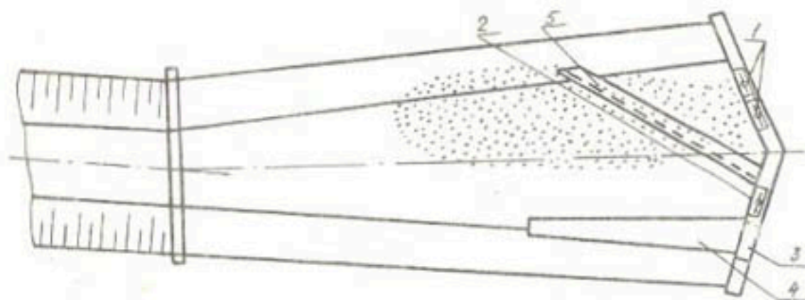
Рис. I. Водораспределительный узел до переустройства.
