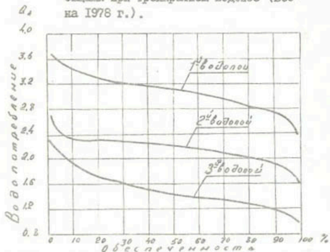
Рис.4. Кривые обеспеченности расходов воды овцами при трехкратном водоопое (ле- то 1978 г.).
