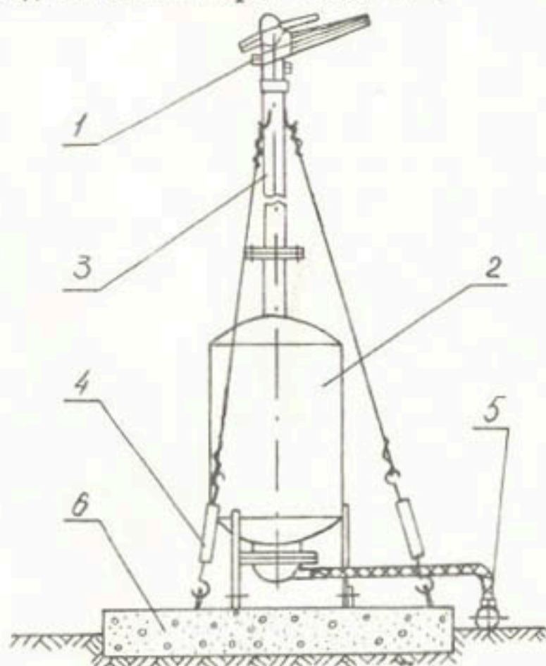
Рис.2. Импульсный дождеватель для надкоронового полива плодовых деревьев: 1-дождевательный аппарат "Роса-3"; 2-пневмогидроаккумулятор; 3-водовыводная труба; 4-растяжки; 5-поливной трубопровод; 6-железобетонная плита.
