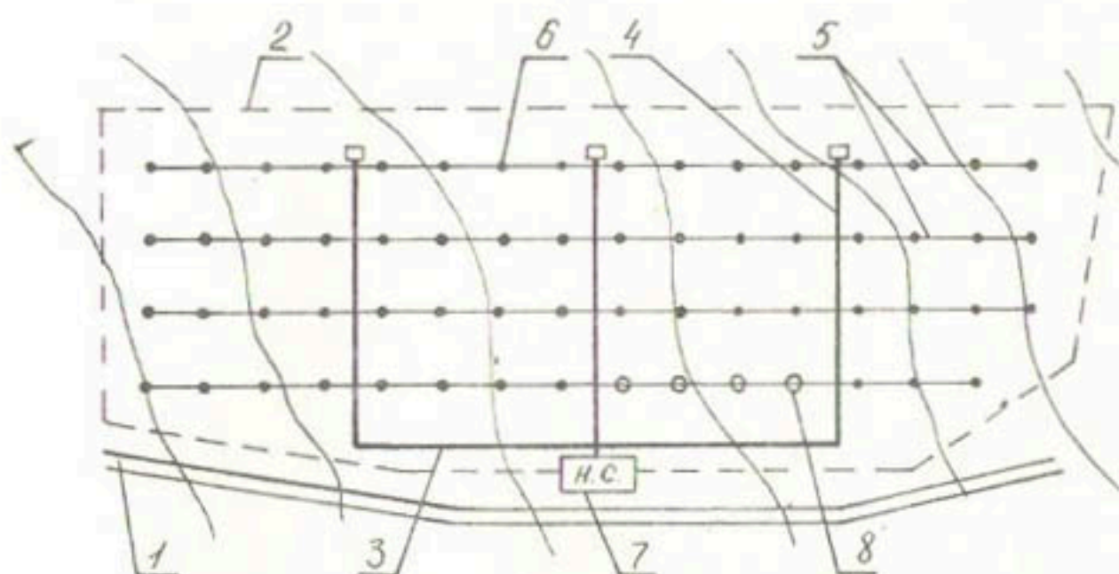
Рис.1. Схема системы в плодвинсовхозе им.Джамбула Джамбулской области: 1-лотковый распределитель; 2-граница орошаемого поля; 3,4,5-магистральные распределительный и поливной трубопроводы; 6-импульсный дождеватель; 7-насосная станция; 8-дождевательный аппарат "Роса-3".
