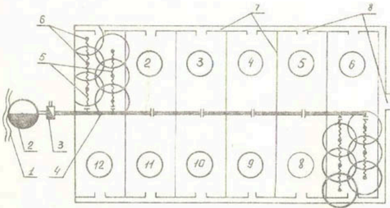
Рис. 1. Технологическая схема полива загонов культурного пастбища ирригационным комплектом с ПИДП:
