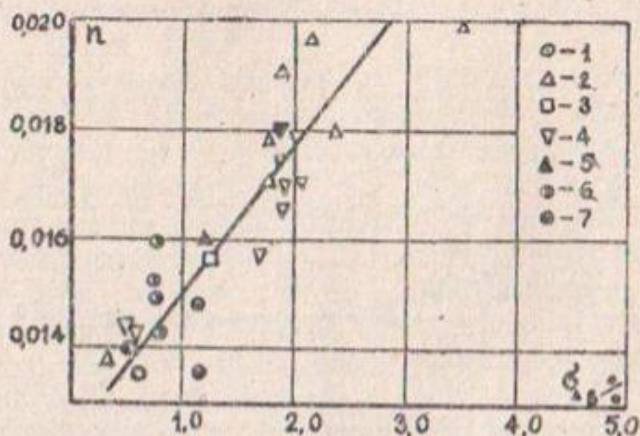
Рис.3. Зависимость коэффициента шероховатости от неравномерности ширины оборного канала из Г-образных блоков
