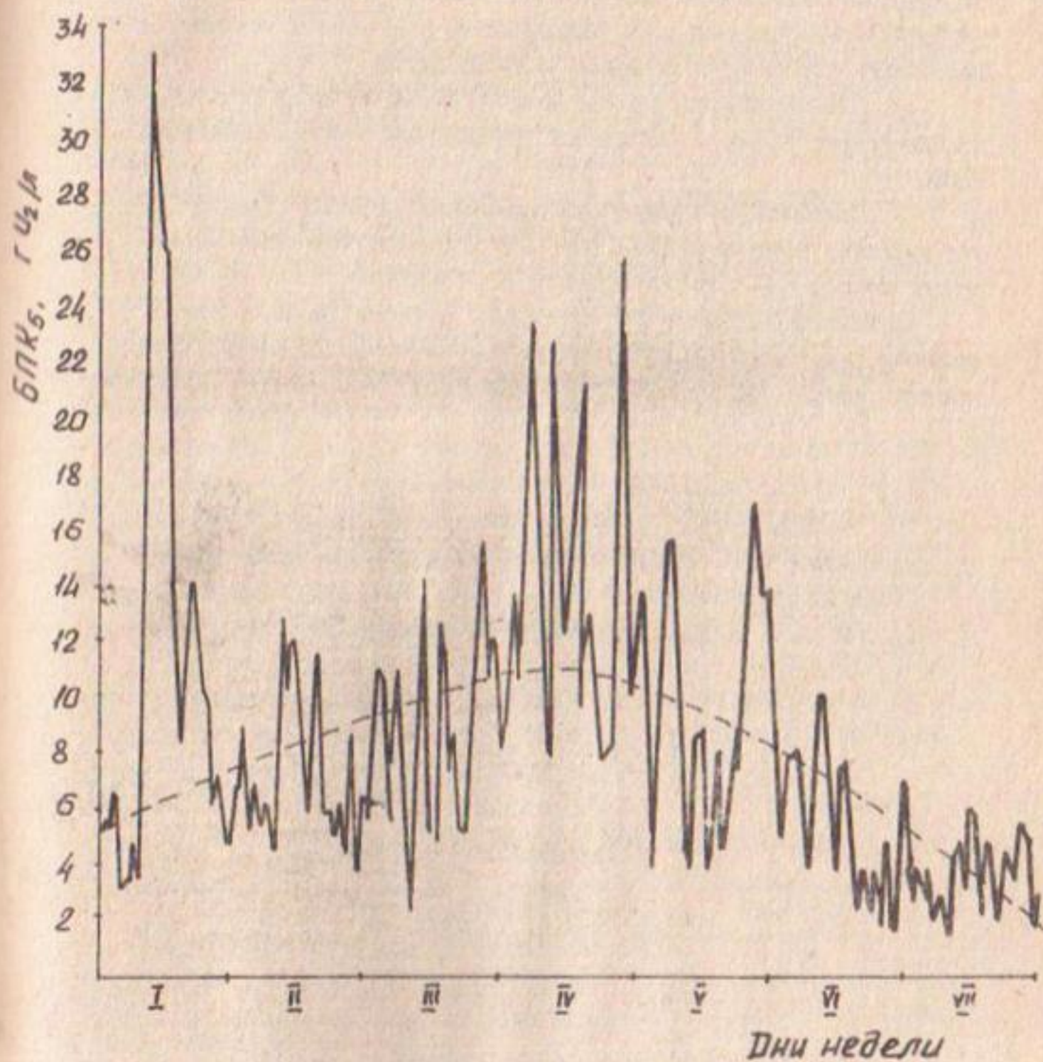
Рис. 3. График колебаний концентраций загрязнений по БПК 5 в течение недели.
