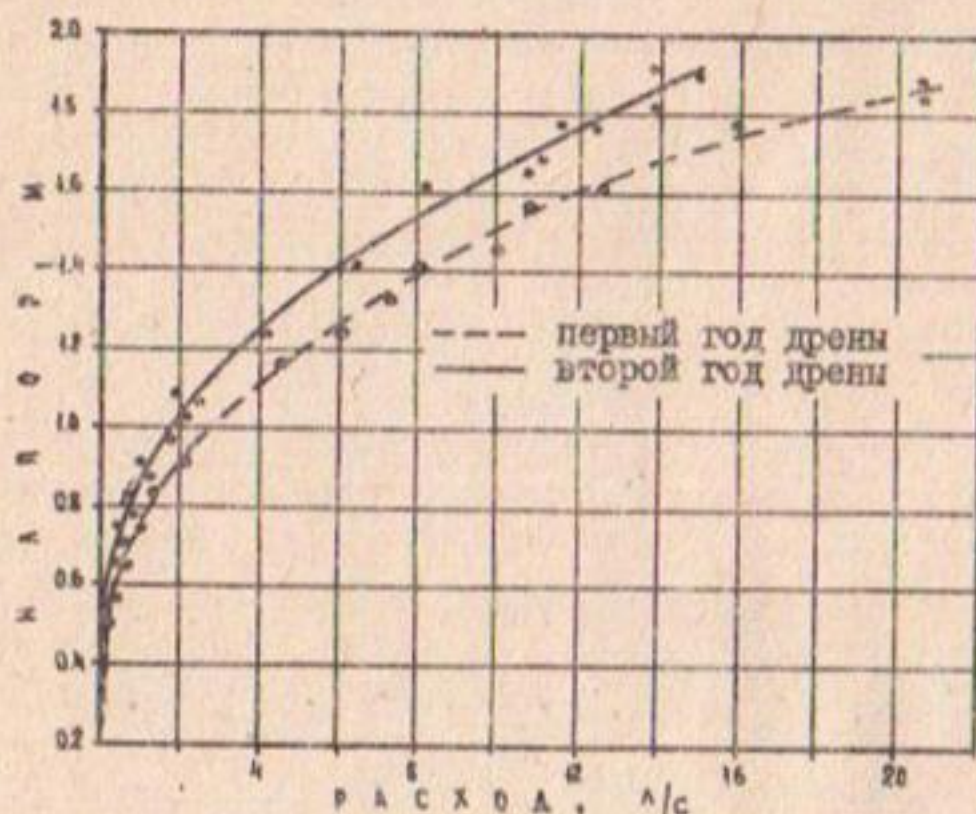
Рис. 2. Графики зависимости расхода воды в дренае ДТ-5 от напора.
