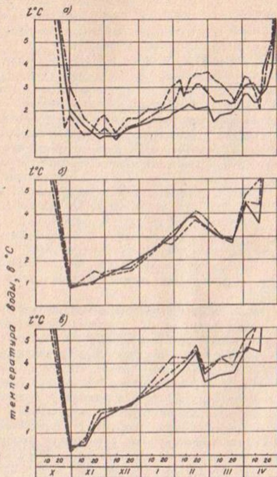
Рис.4. Температурный режим водохранилищ канала Иргыш-Караганда зимой 1977-1978 гг.
