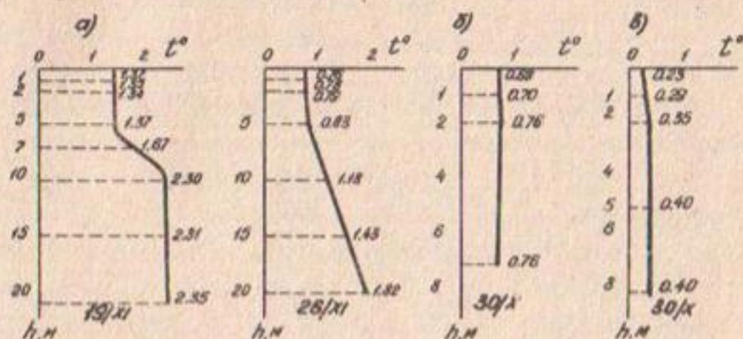
Рис.2. Температурные эпюры водохранилищ канала Иртыш-Караганда перед замерзанием: а) гидроузел №1; б) гидроузел №4; в) гидроузел №5.
