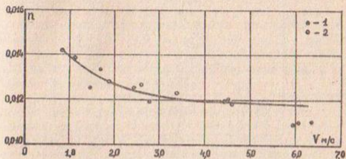
Рис.1. Зависимость коэффициента шероховатости в параболических лотках от скорости потока.
