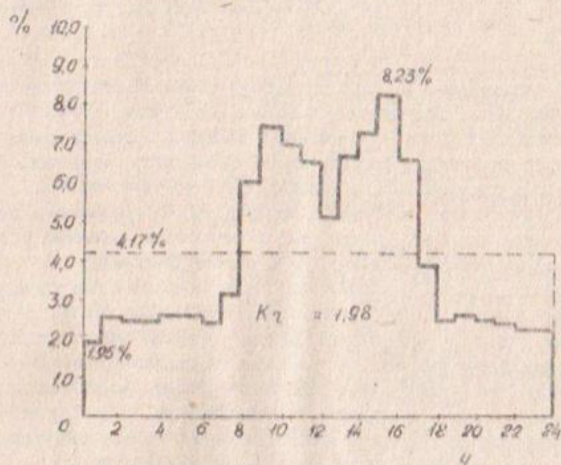
Рис. 1. График поступления расхода сточных вод в приемный резервуар по часам суток в процентах от суточного расхода.
