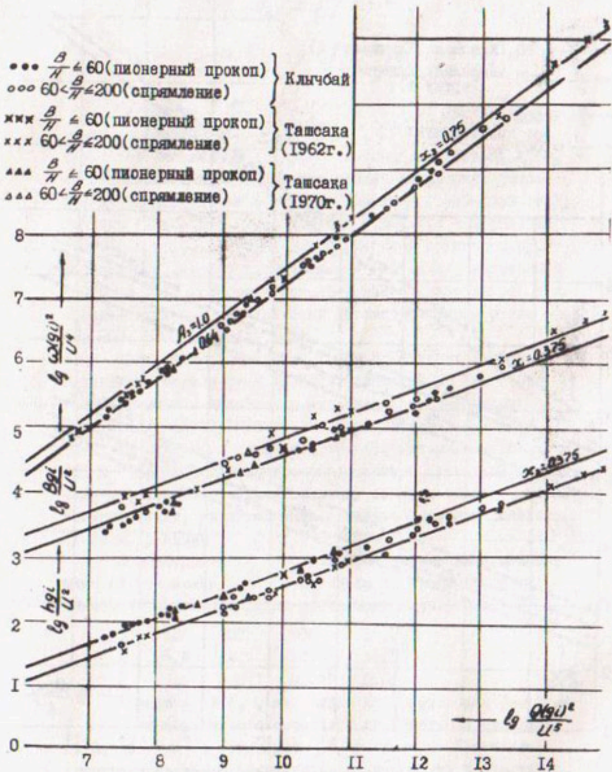
Рис.2. Совмещенный график зависимости между критериями \frac{Bq}{U^2} , \frac{hq}{U^2} , \frac{\omega(q)^2}{U^4} и \frac{Q(q)^2}{U^5} для спрямлений.
