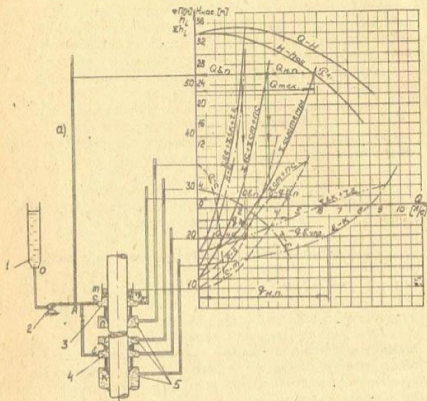
Рис. 2. Гидравлические характеристики работы системы технического водоснабжения насоса ОП10-260 на насосных станциях КМК: а) Схема технического водоснабжения подшипников насоса ОП10-260; 1 - отстойник; 2 - насос техводоснабжения 2К6; 3, 4 - камеры подшипников; 5 - полости насоса, куда течет смазывающая вода;
