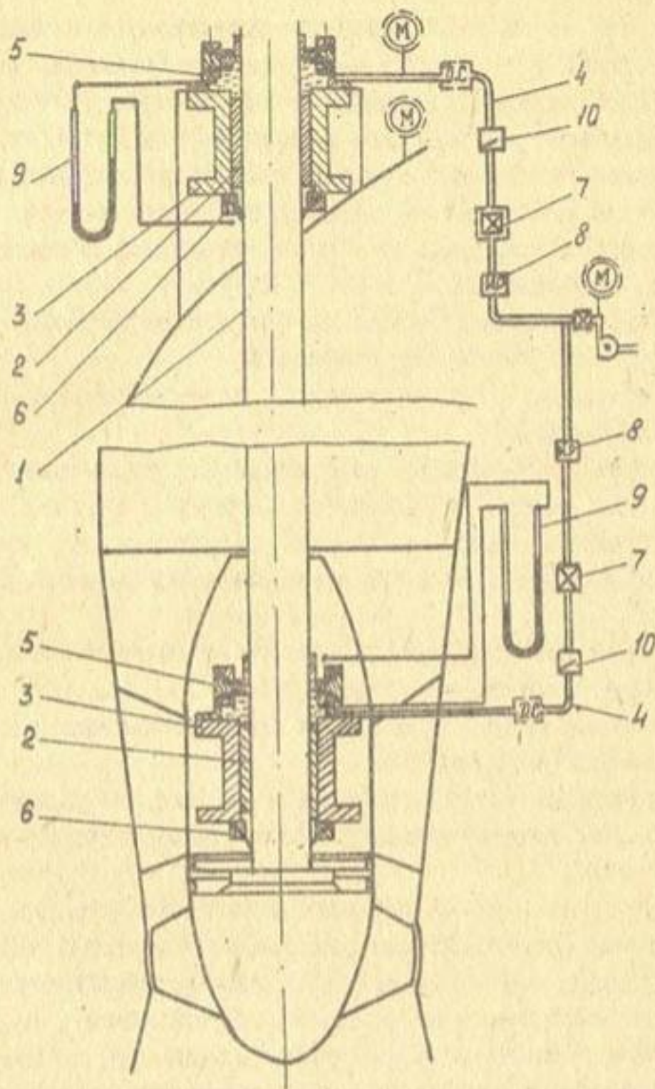
Рис.1. Принципиальная схема существующего техводоснабжения подшипников насоса ОП10-260: 1 - вал насоса; 2 - вкладыш подшипника; 3 - его корпус; 4 - труба для подачи технической воды; 5 - верхнее уплотнение; 6 - нижнее уплотнение; 7 - дроссельное устройство; 8 - измеритель расхода; 9 - дифманометр; 10 - обратный клапан; ДС - датчик струи. Примечание: имеющиеся на станции приборы и устройства обведены пунктиром.
