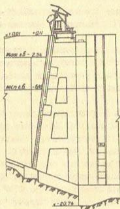
Рис. I. Прилонное-сороудерживающее сооружение насосной станции Шерабад.
