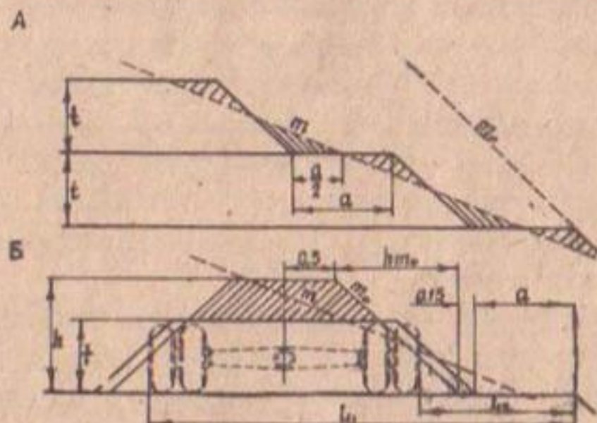
Рис. 4. А - схема отсыпки грунта у откоса плотины; Б - схема для расчета значения "Л".
