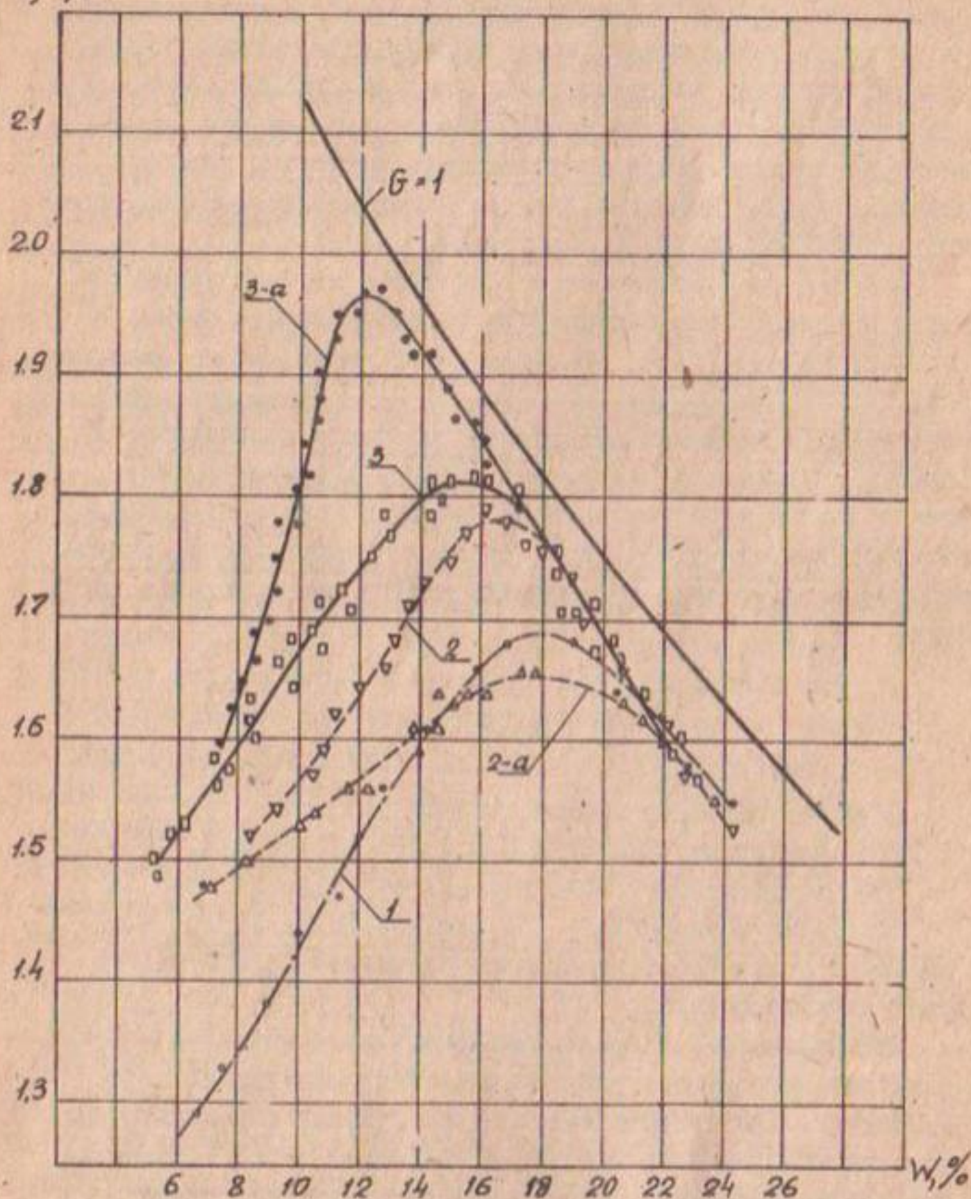
Рис.3. Зависимость плотности исследуемых грунтов " \delta " от их влажности " W " при работе уплотнения 0,045 \text{ кг/см}^2 : 1, 2 и т.д. — номера исследуемых грунтов.
