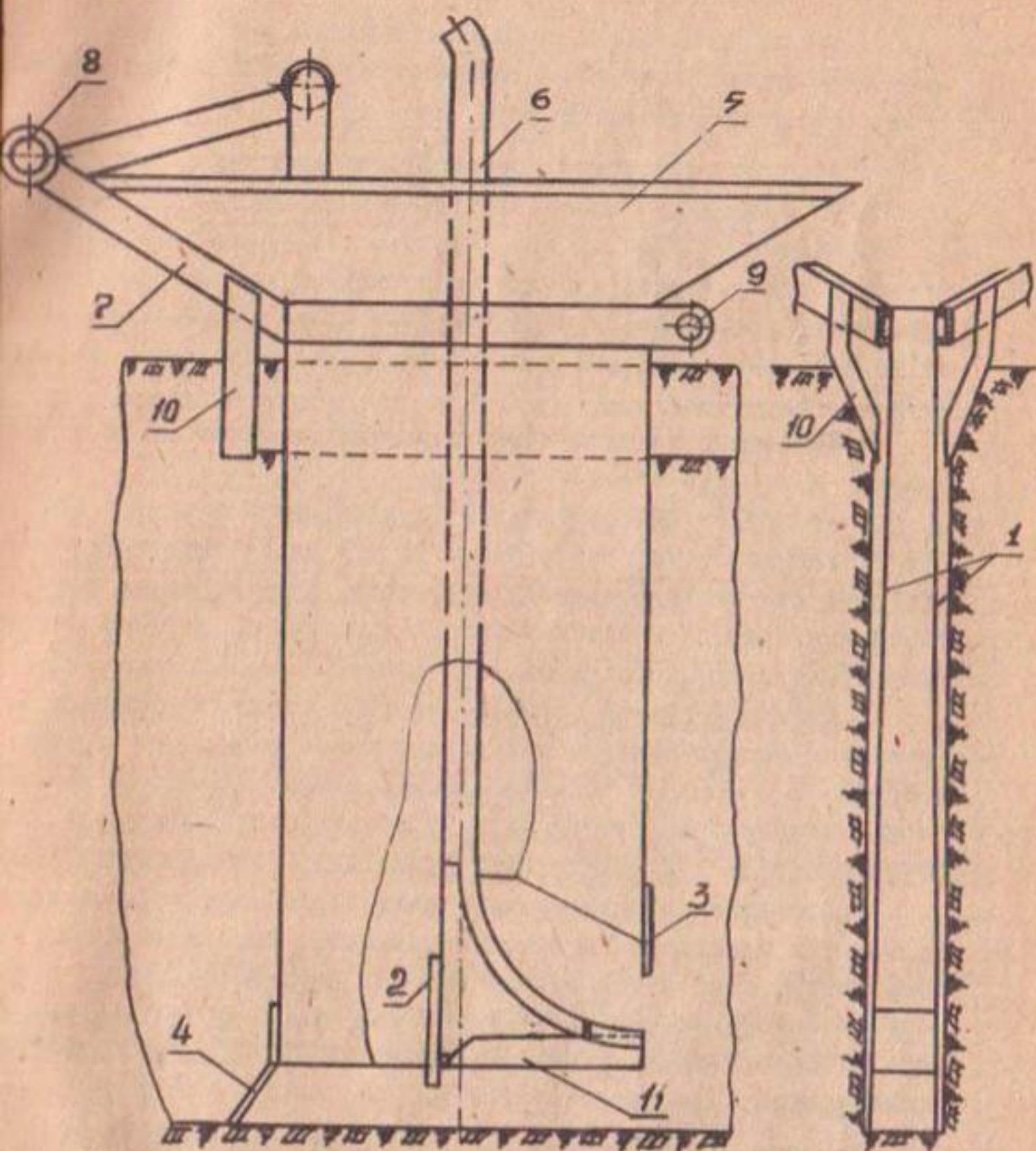
Рис. 3. Бункер дренаукладчика.
