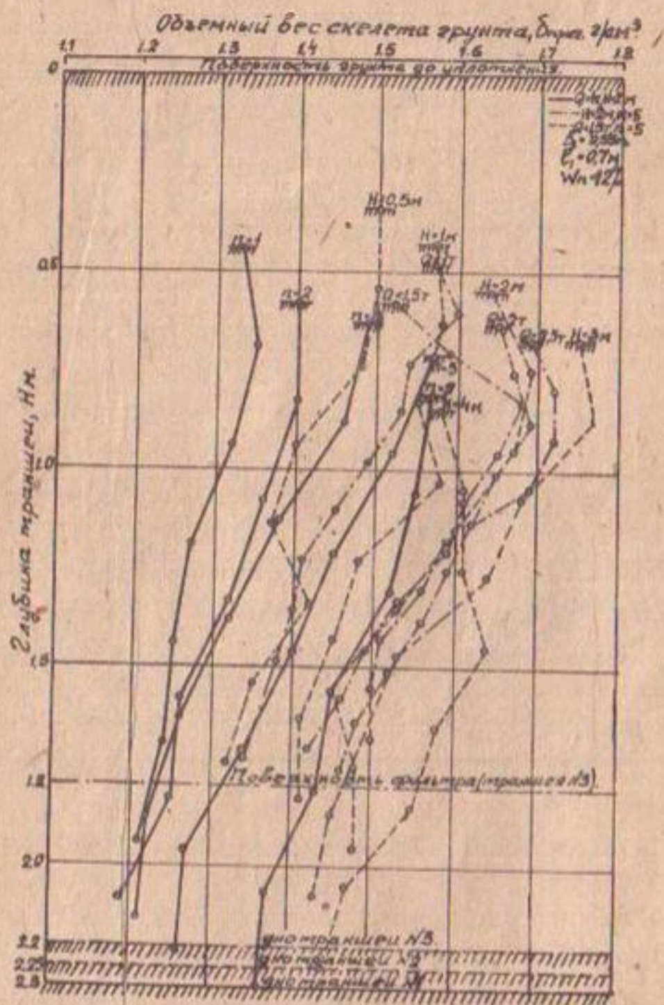
Рис. 5. Изменение плотности грунта \delta_{прив} от веса \alpha , высоты сбрасывания и числа ударов n трамбующего органа длиной 0,7 м.
