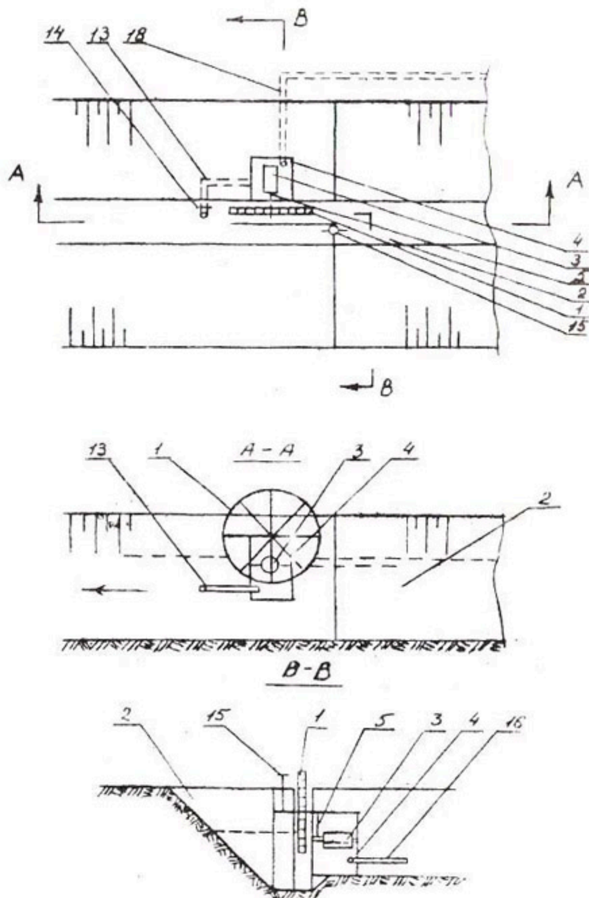
Рис. I. Схема расположения приводного устройства и рабочего органа водоподъемной установки
