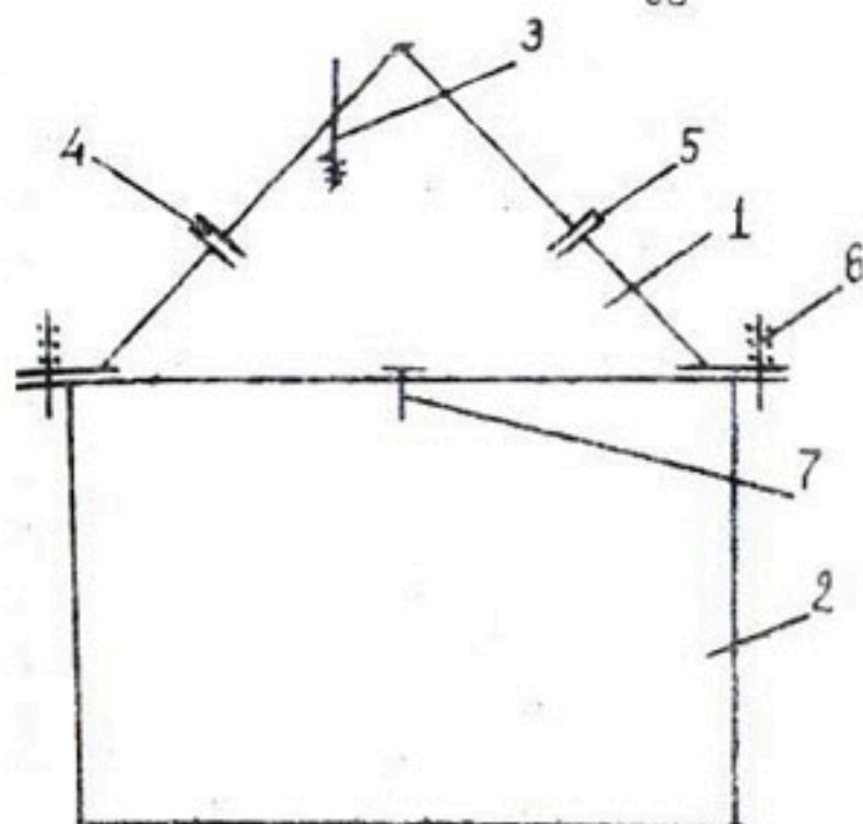
Рис.1. Газовзрывное устройство:
