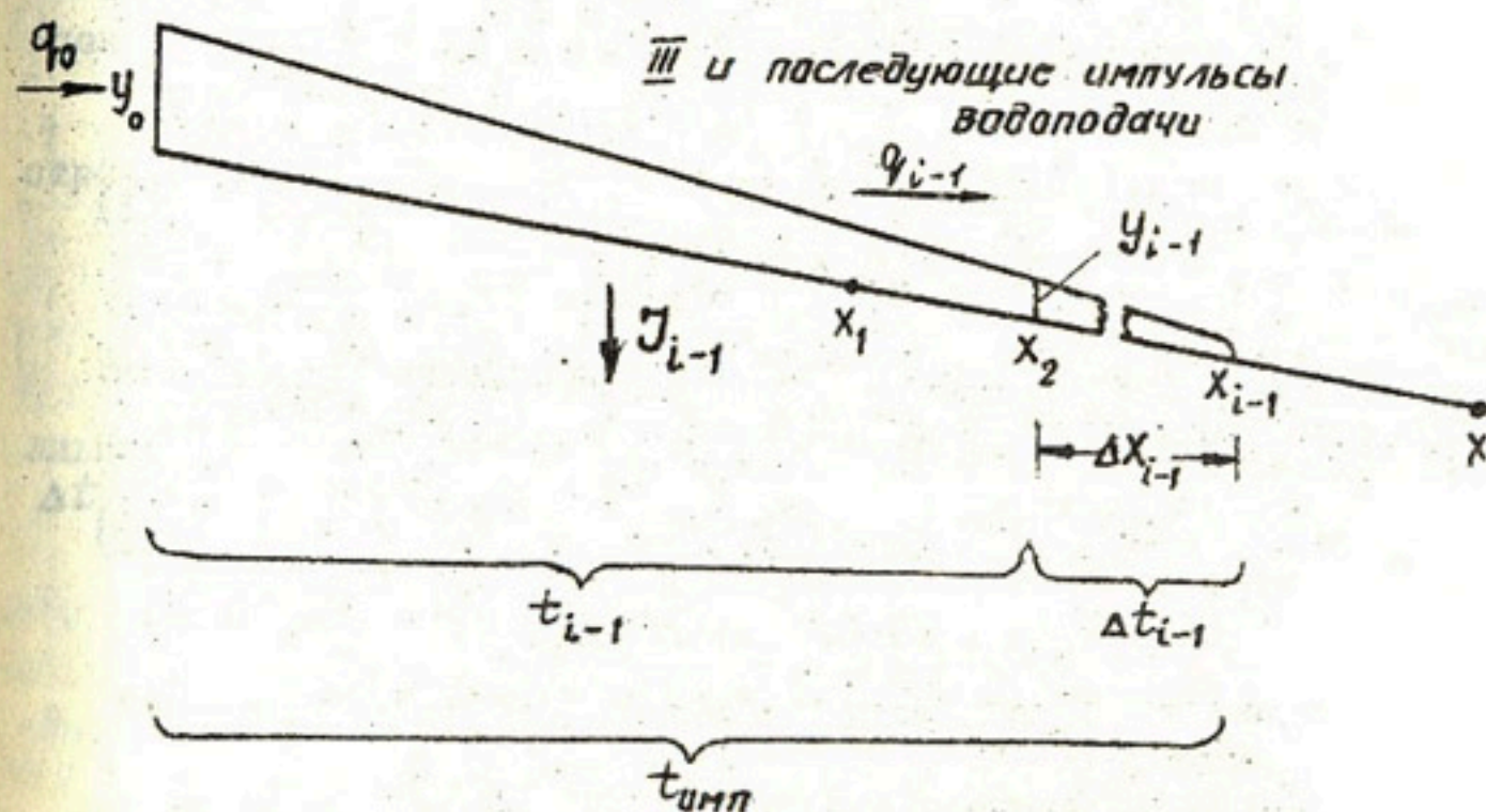
Схема к расчету дискретного регулирования водоподачи в поливные борозды
