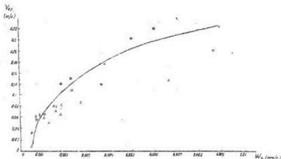
Рис.5. График зависимости критической скорости V_{кр} от средневзвешенной гидравлической крупности частиц наилок
