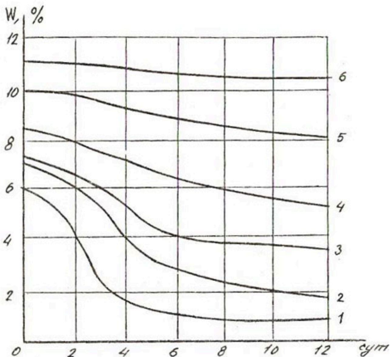
Рис.2. Динамика изменения влажности под влажнопесчаным покрытием в течение 12 сут при T=75^{\circ}\text{C} : глубина (см): 1-0; 2-5; 3-10; 4-20; 5-25; 6-30.
