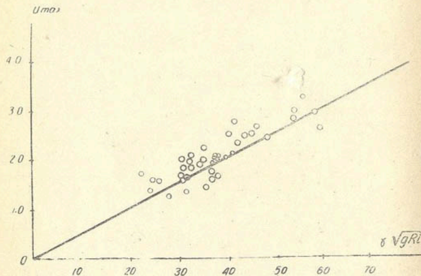
Рис. 23. Зависимость максимальной гидравлической крупности от динамической скорости потока.
