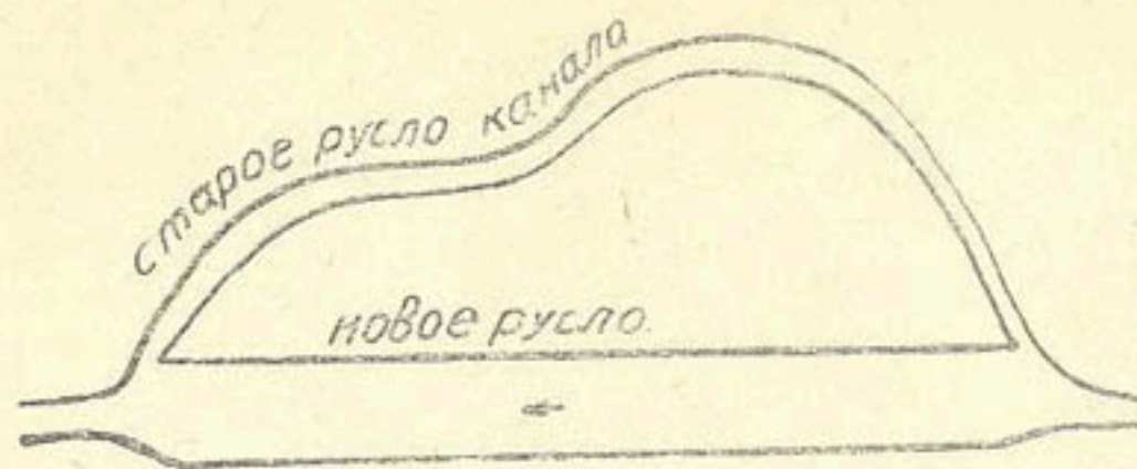
Рис. 26. План участка спрямления канала имени Ленина.
