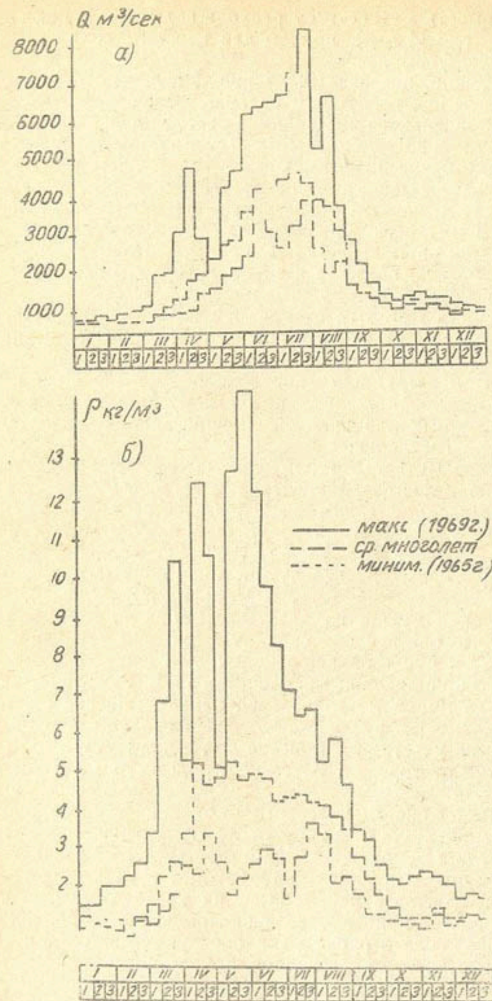
Рис. 2. Гидрографы среднедекадных расходов (а) и мутности (б) воды по створу Керки.
